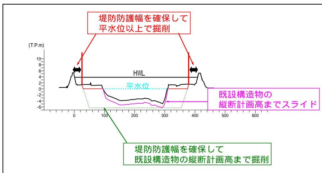
図 5-2 旧北上川設定河道横断面図
