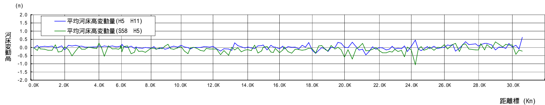
図2-3 【江合川】低水路平均河床高縦断面図(上)、河床変動高縦断面図(下)
