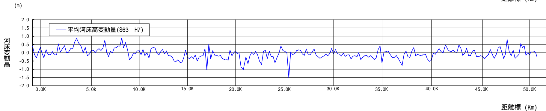
図2-1(1) 【北上川：宮城県】低水路平均河床高縦断図(上)、河床変動高縦断図(下)
