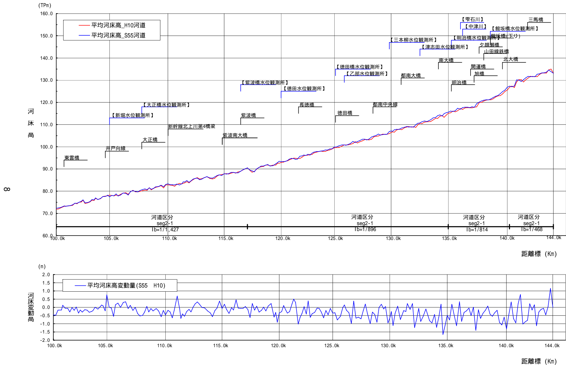
図2-1(4) 【北上川：岩手県】低水路平均河床高縦断図(上)、河床変動高縦断図(下)
