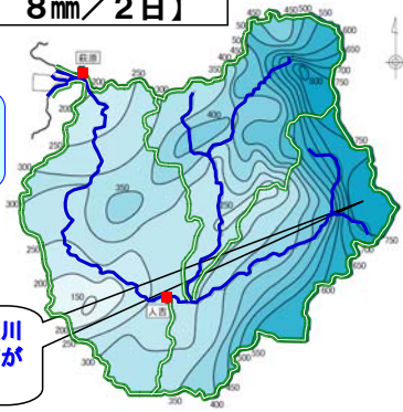
平成17年9月洪水 【460.8mm/2日】
