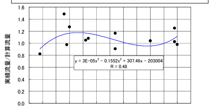
1995年(平成7年)適合モデルによる計算流量と実績流量の比
