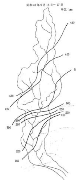
図 4-4 大井川流域の等雨量線図
