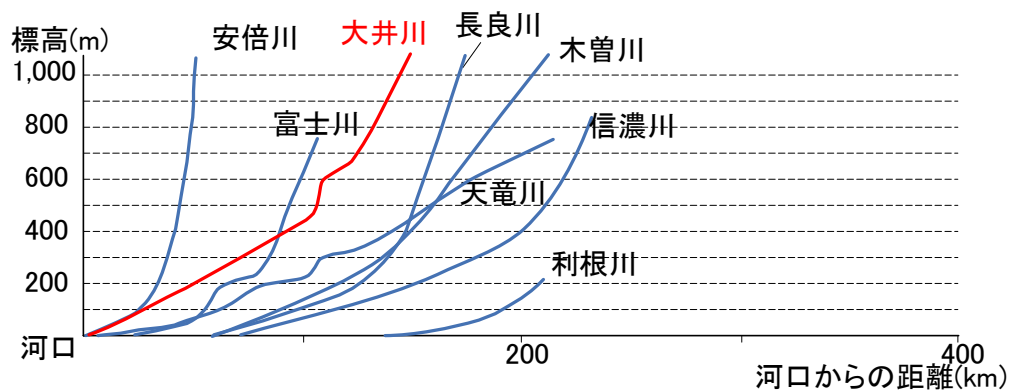
図 8-1 河床勾配の比較
