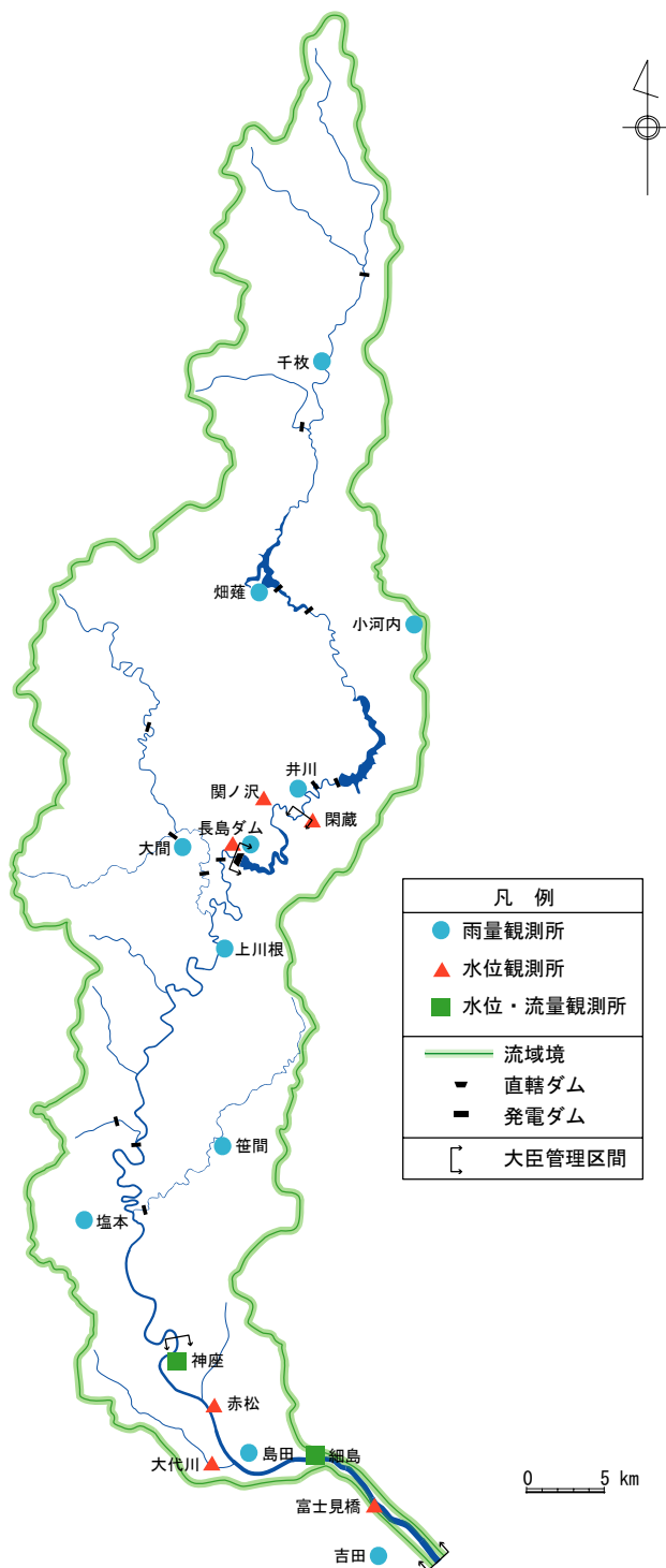
図 9-2 大井川水系雨量観測所・水位観測所位置図
