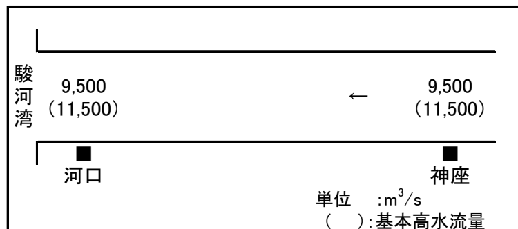
図 4-12 大井川水系工事実施基本計画の流量配分 (昭和 49 年 3 月)
