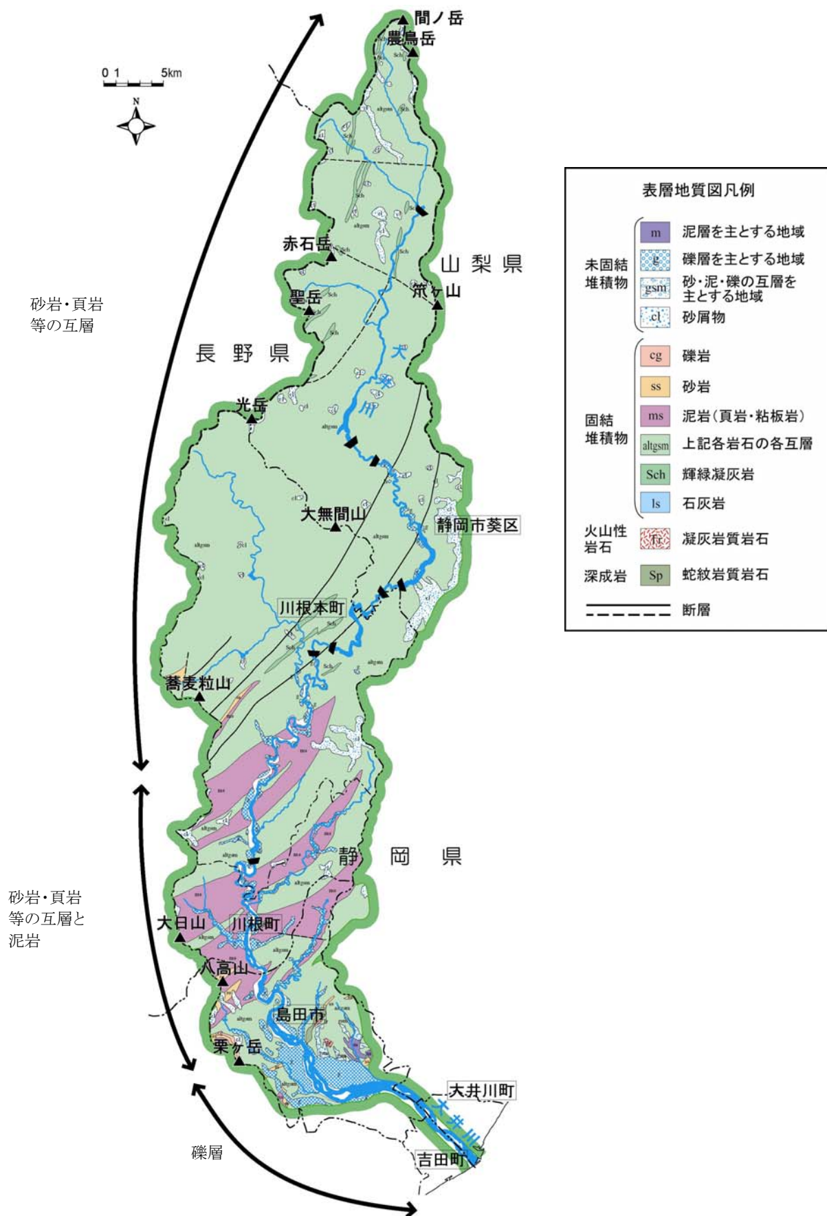
図 1-8 大井川流域の地質図
