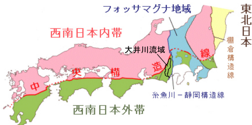
図 1-7 中央構造線と糸魚川静岡構造線の位置
