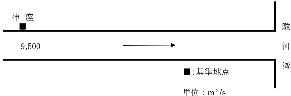
図 6.1 大井川計画高水流量図
