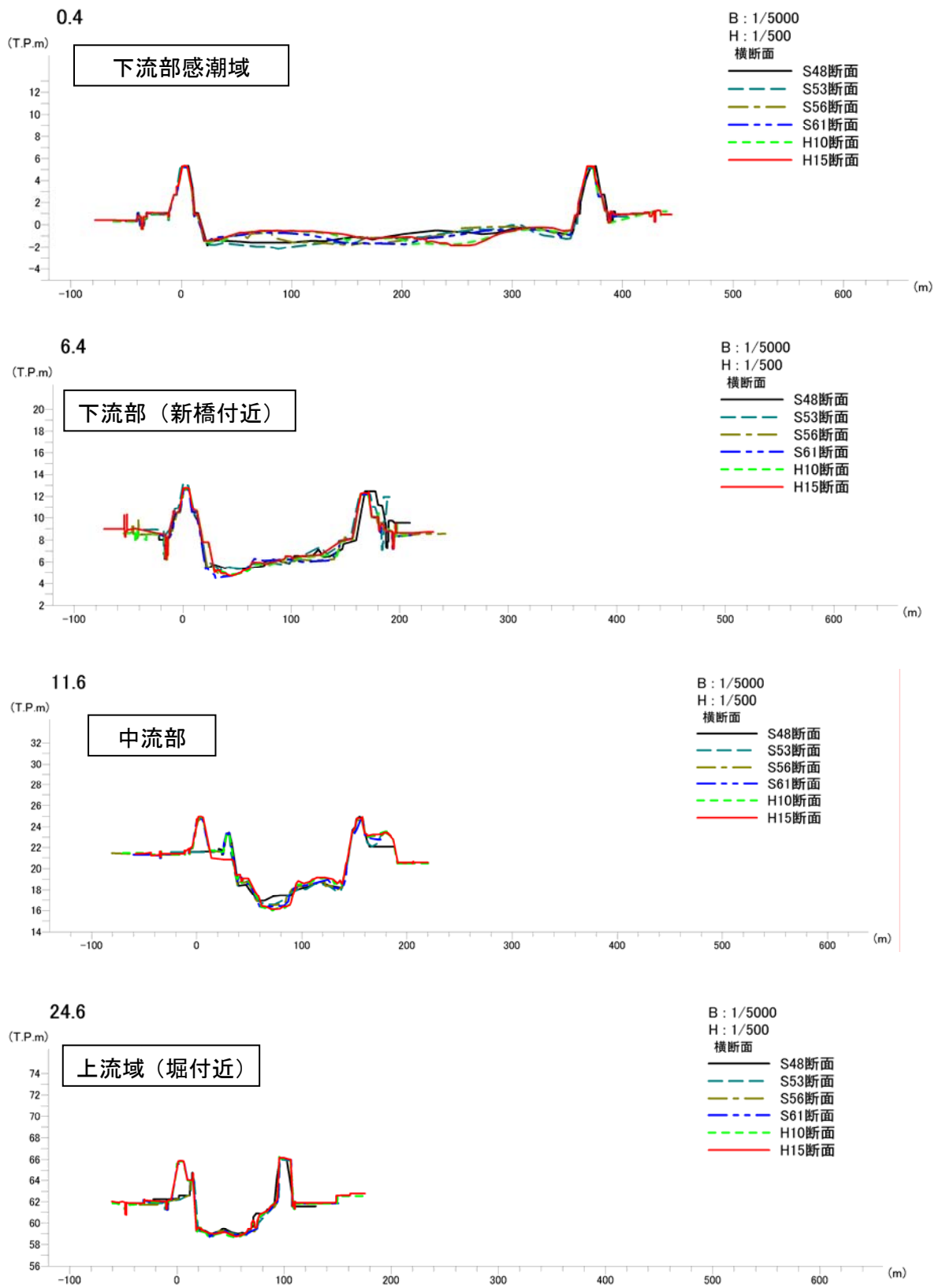
図 2-4 佐波川横断面図経年変化（各河川区分毎）
