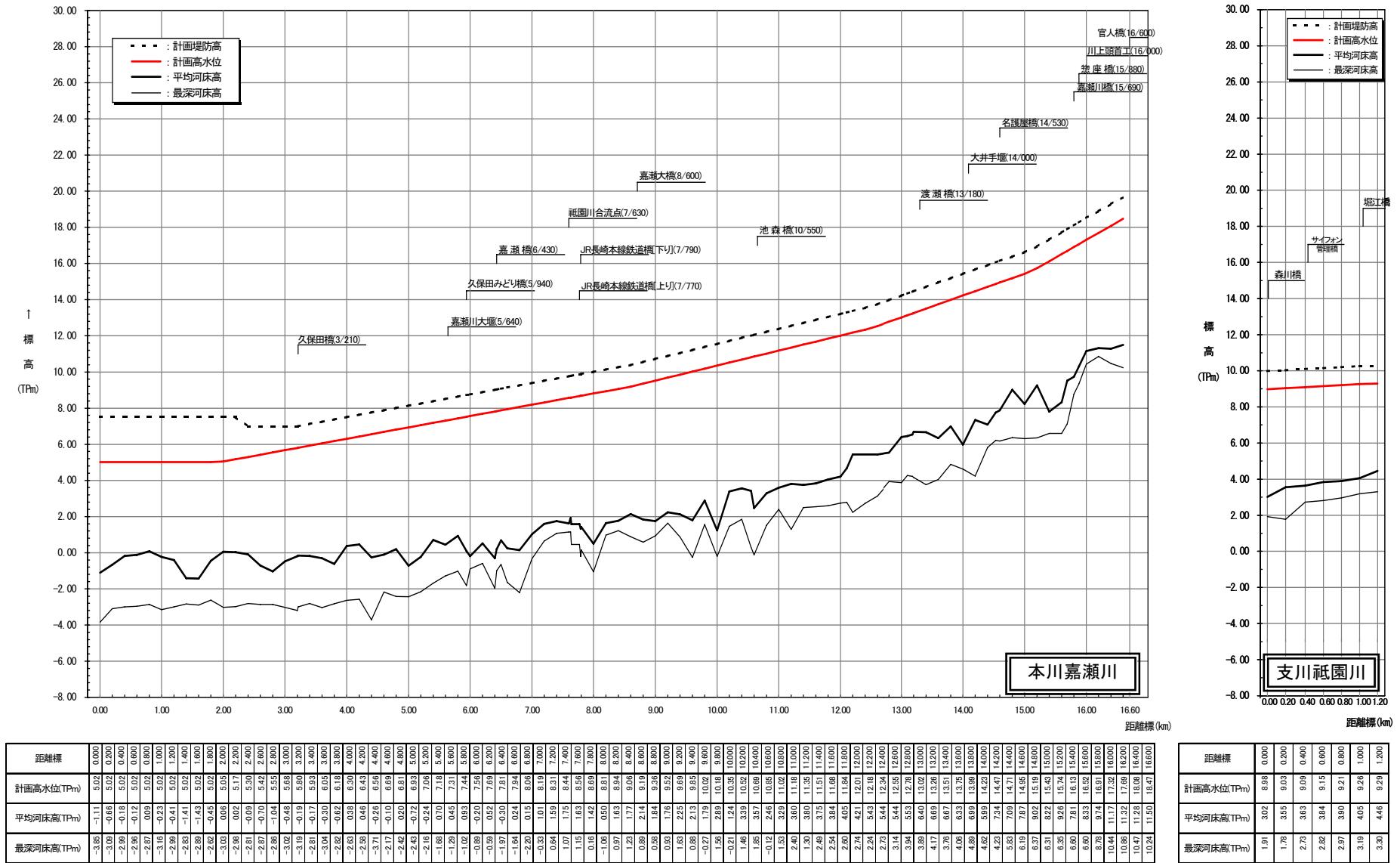
図 7 - 1 計画縦断図 (左 : 本川嘉瀬川、右 : 支川祇園川)
