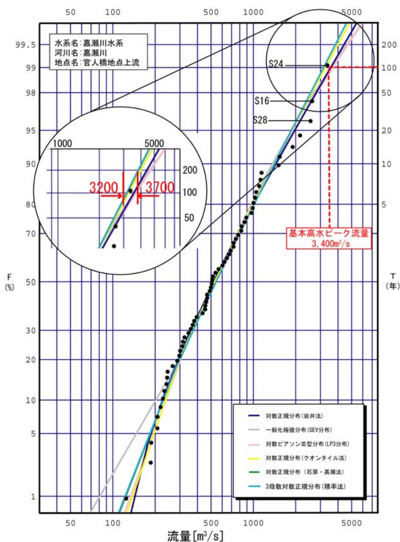
図 4-7 官人橋地点流量確率計算結果図
