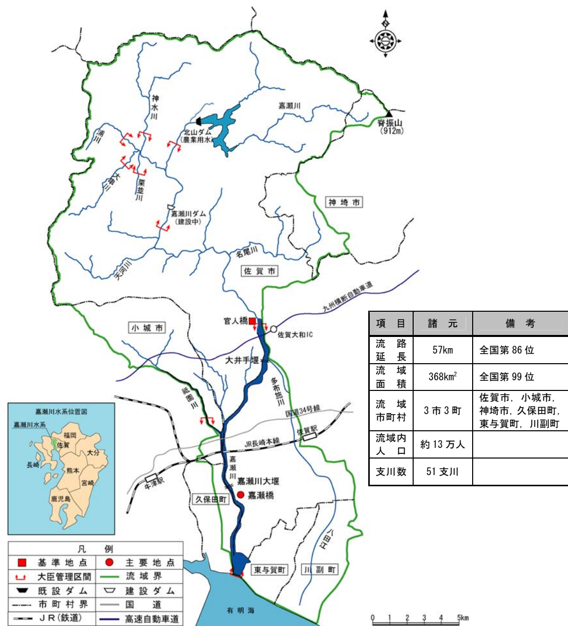
図 1-1-1 嘉瀬川水系流域概要図
