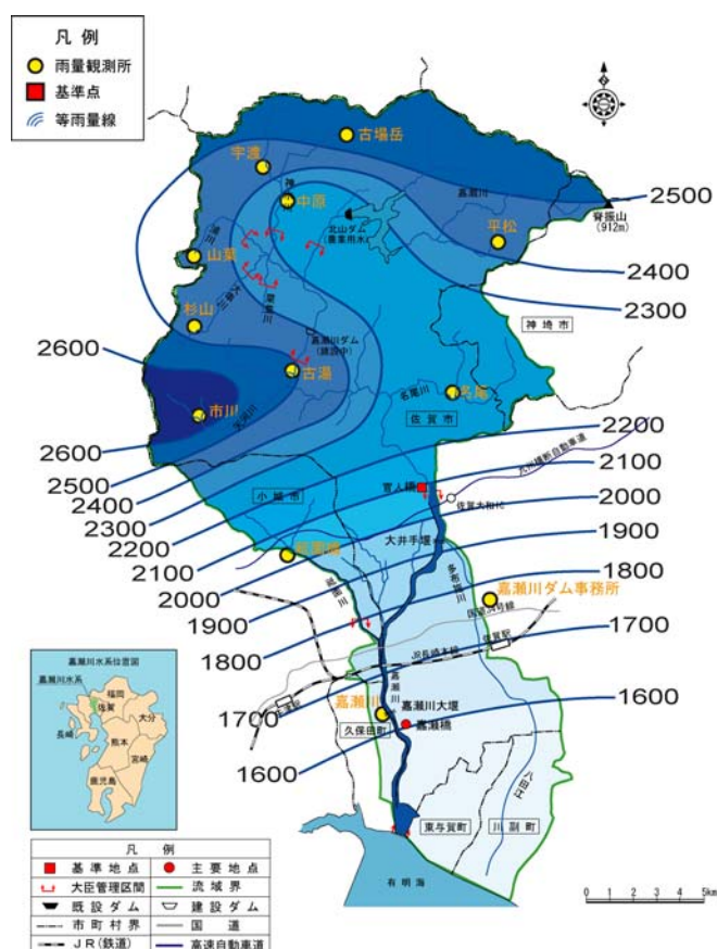
図 1-4-3 嘉瀬川年等雨量線図 (1995～2004 年までの 10 年間の年平均降水量)
