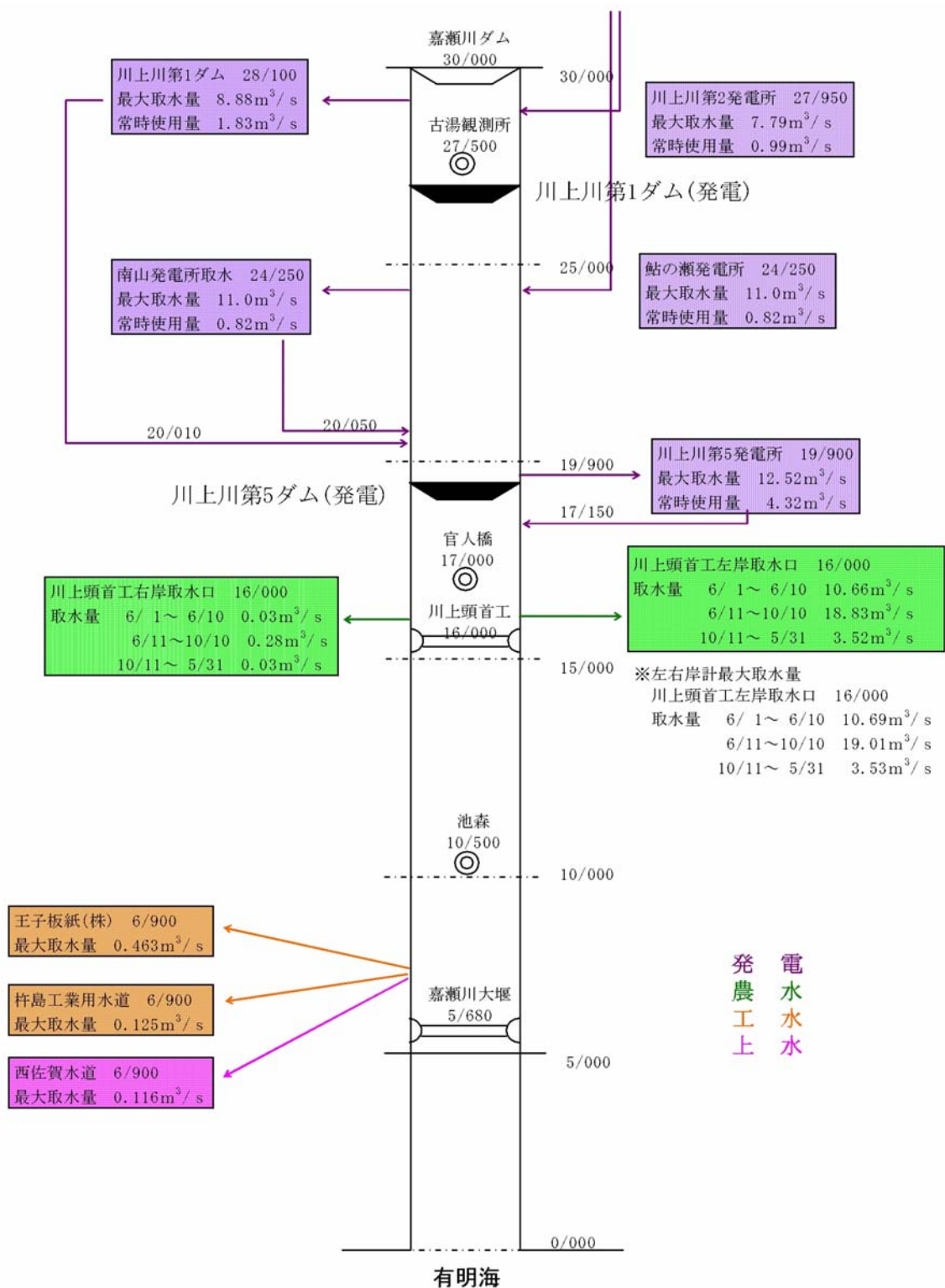
図5-1-5 嘉瀬川の水収支模式図
