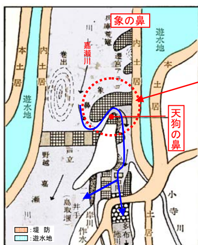
図5-1-1 石井樋等の利水施設の機能説明図
