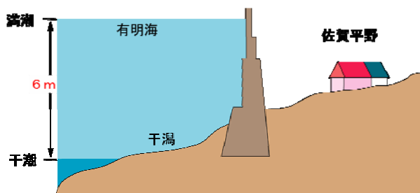
図 2-2-1 有明海特有の干満差
