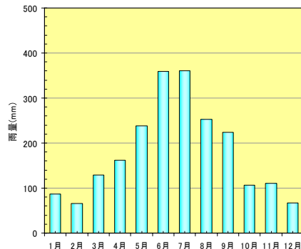
図 1-4-2 官人橋上流の月別降水量 (1995～2004 年までの 10 年間の月別平均降水量)
