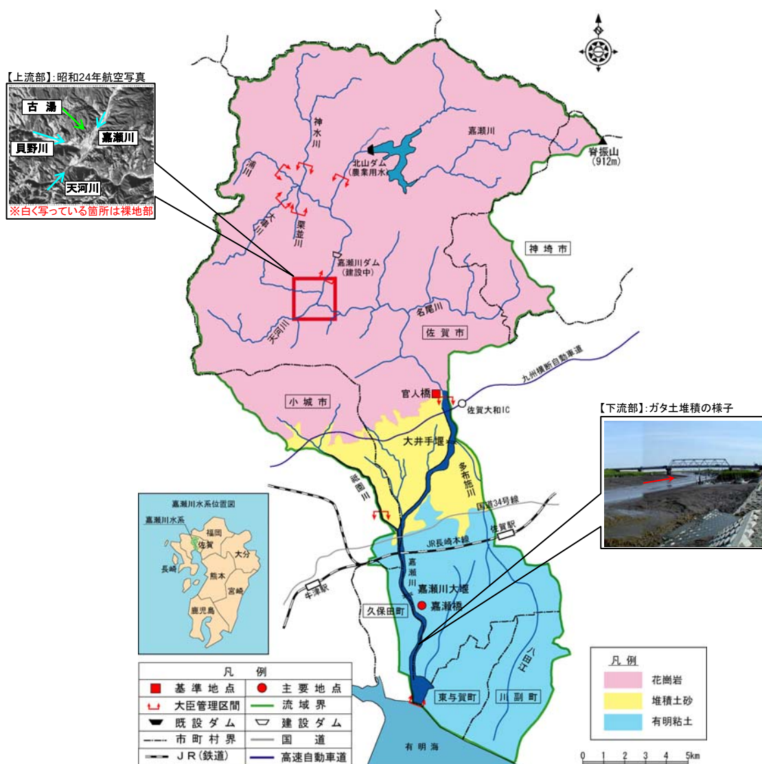
図 1-3-1 嘉瀬川流域地質図
