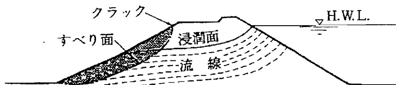
図2 堤防の浸透破壊の機構
