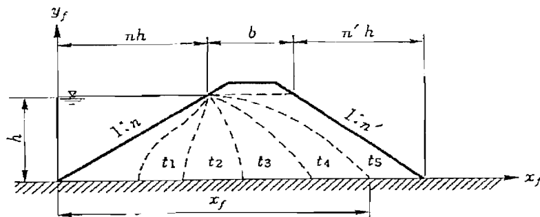
図1 堤体内の浸潤面の時間的变化
