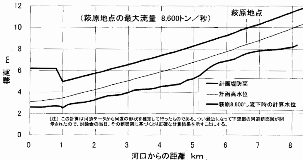
図15 川辺川ダムがない場合の八代地区の最高洪水位(不等流計算)
