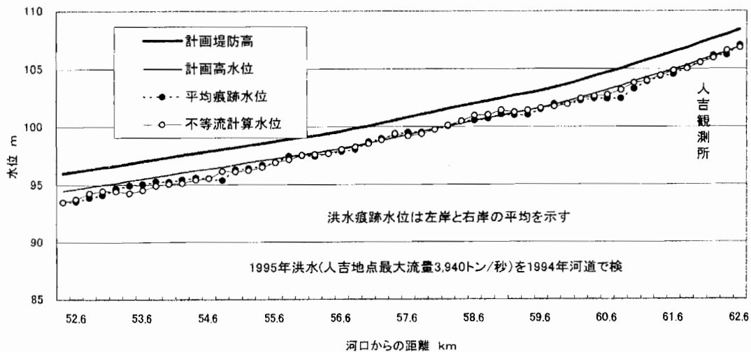
図12 1995年洪水の再現計算(人吉地区)
