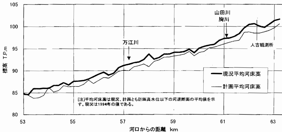
図9 人吉地区の河床高
