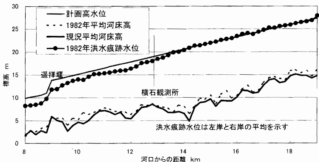
図18 球磨川中流部(坂本村)
