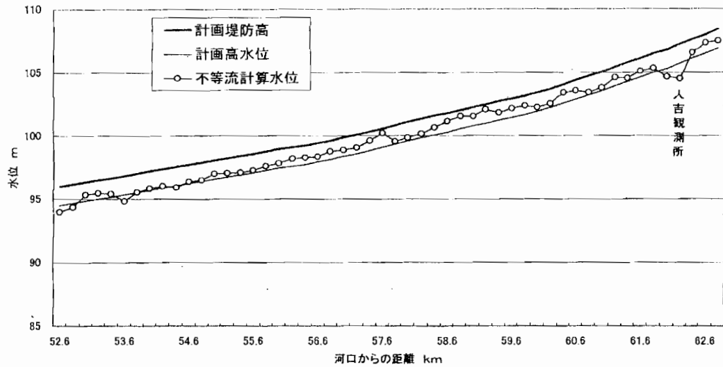
図13 計画河道を6,150トン/秒の洪水が流れた時の最高水位(人吉地区区)
