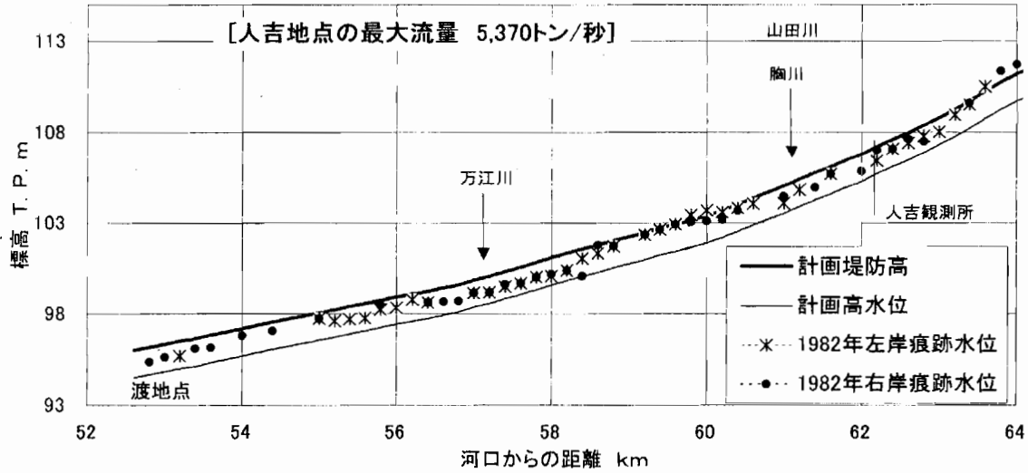
図11 計画河道を1982年洪水が流れたときの水位(人吉地区)
