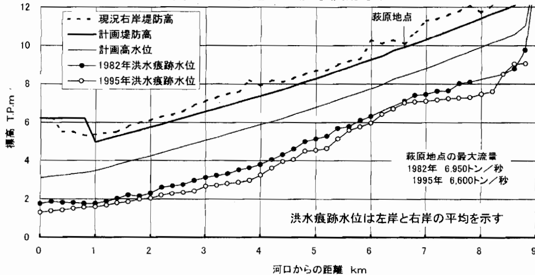
図14 八代地区の洪水痕跡水位
