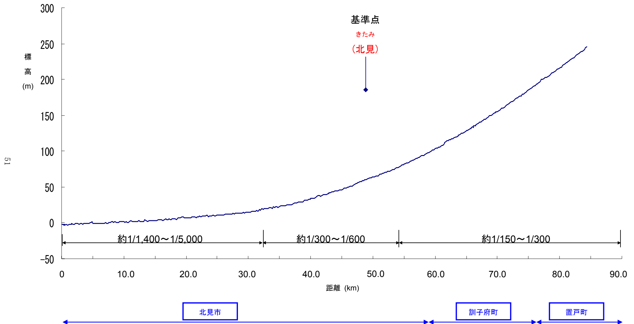
図 8-1 常呂川水系 常呂川 河床高縦断面図
