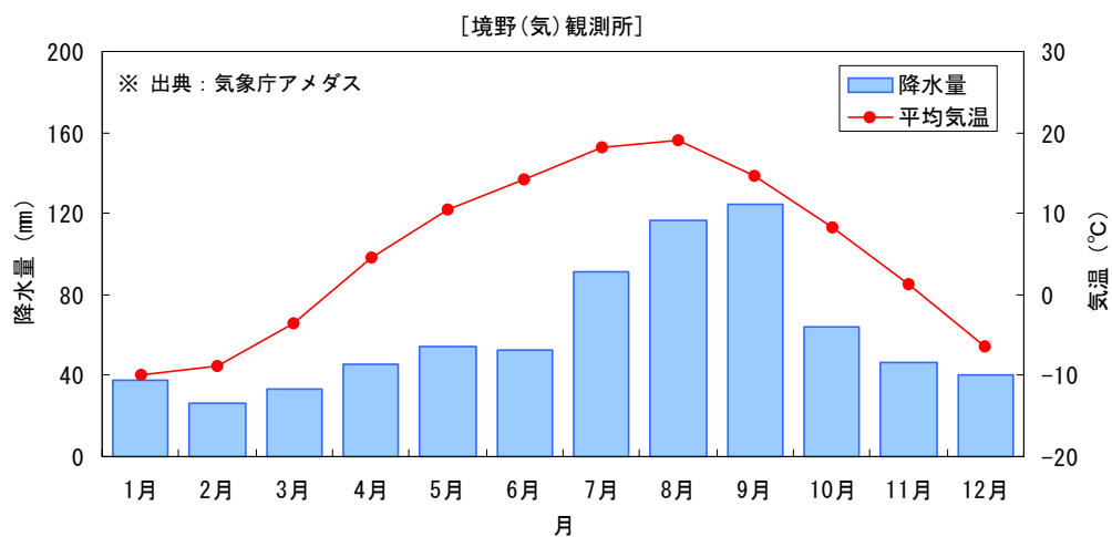
図 1-7 境野地点の降水量と平均気温[過去 20 ヶ年(1985～2004)の平均]
