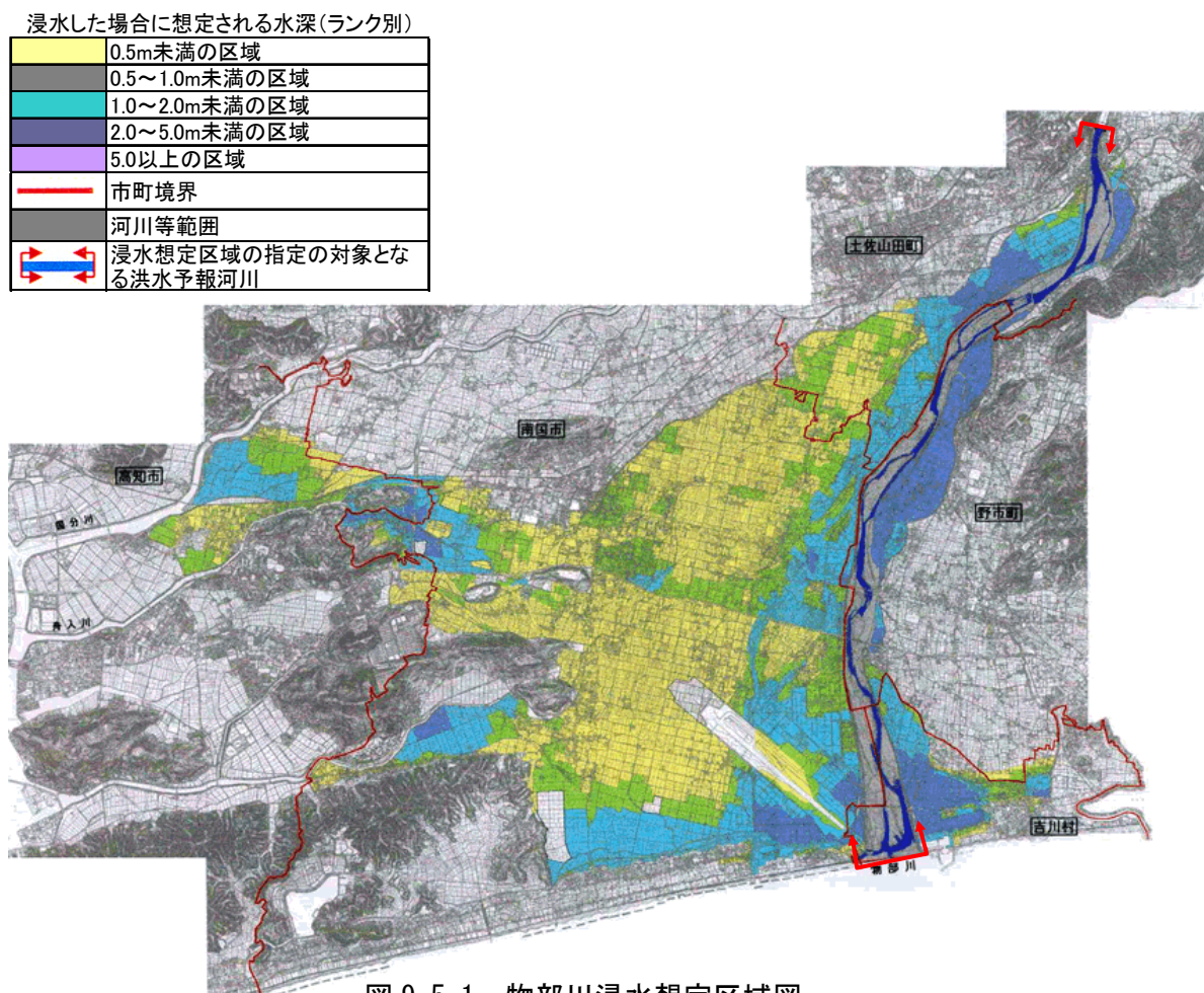
図 9.5.1 物部川浸水想定区域図
