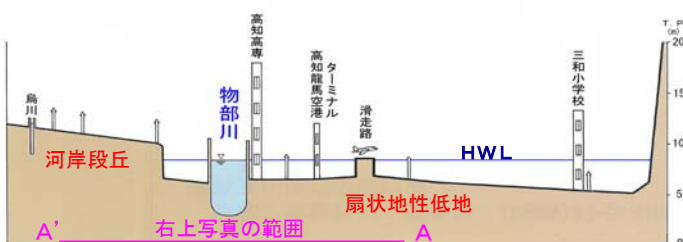
図 1.2.3 下流部の地形縦断面図
