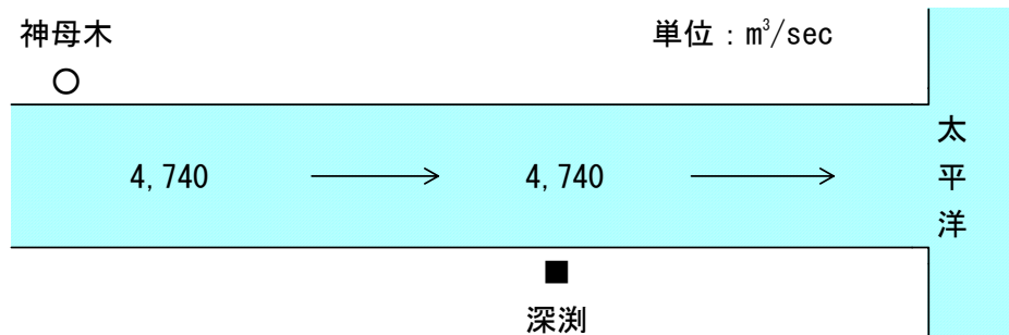
図 4.3.4 工事実施基本計画流量配分図
