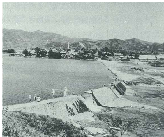
図 4.3.2 明治 44 年当時の山田堰（現在は撤去）
