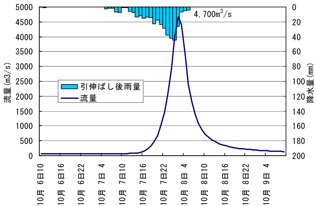
図 4-4 (1) 昭和 19 年 10 月型のハイドログラフ（名取川名取橋地点）
