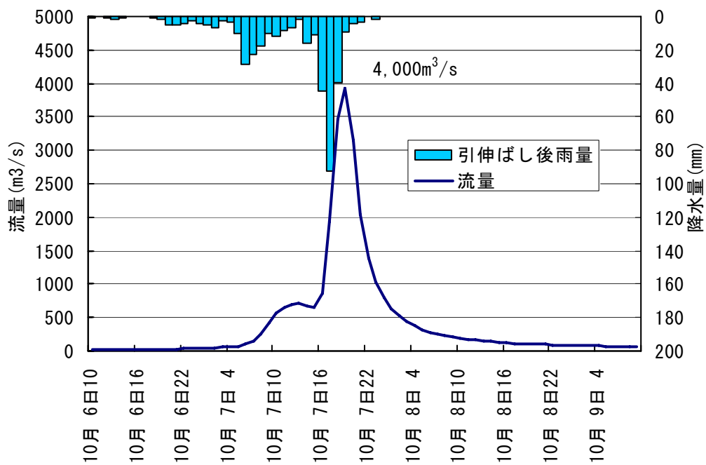
図 4-4 (2) 昭和 22 年 9 月型のハイドログラフ（広瀬川広瀬橋地点）
