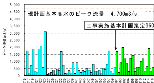
図 4-5 (2) 年最大流量（ダム・氾濫戻し流量、名取川名取橋地点）
