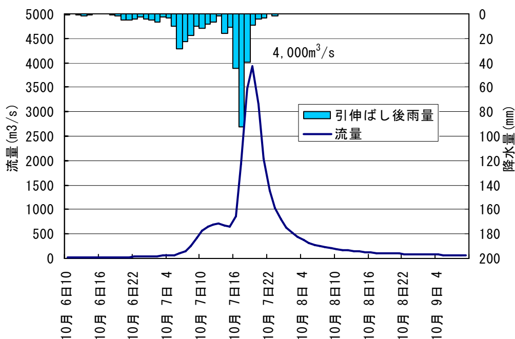
図 4-10 (2) 昭和 22 年 9 月型ハイドログラフ (広瀬川広瀬橋地点)
