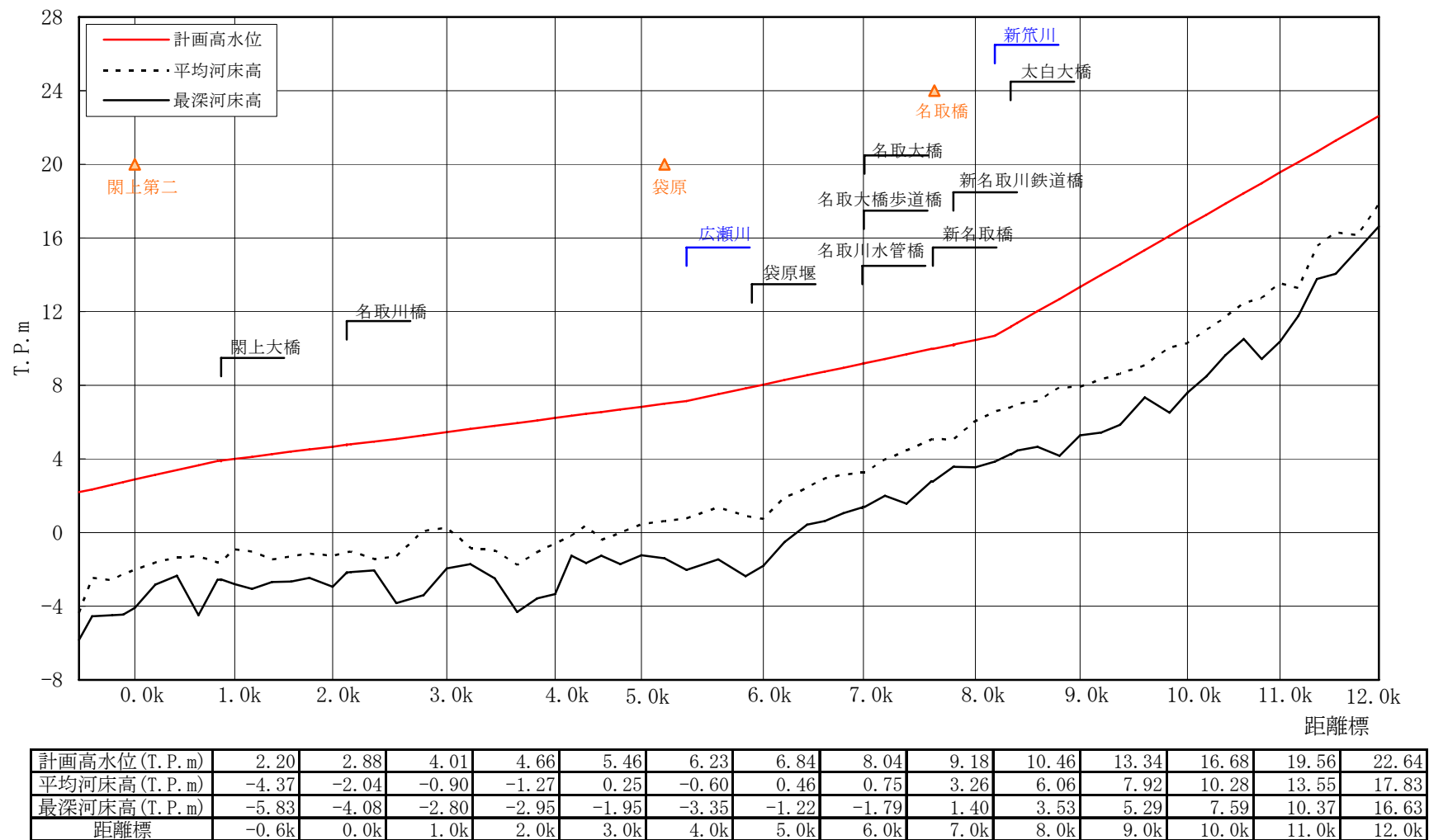
図 8-1 名取川計画縦断面図
