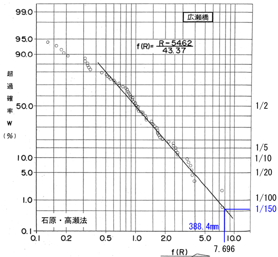
図 4-1 (2) 広瀬川広瀬橋地点における雨量確率評価
