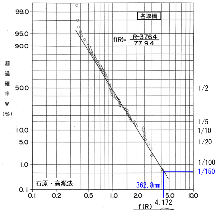
図 4-1 (1) 名取川名取橋地点における雨量確率評価
