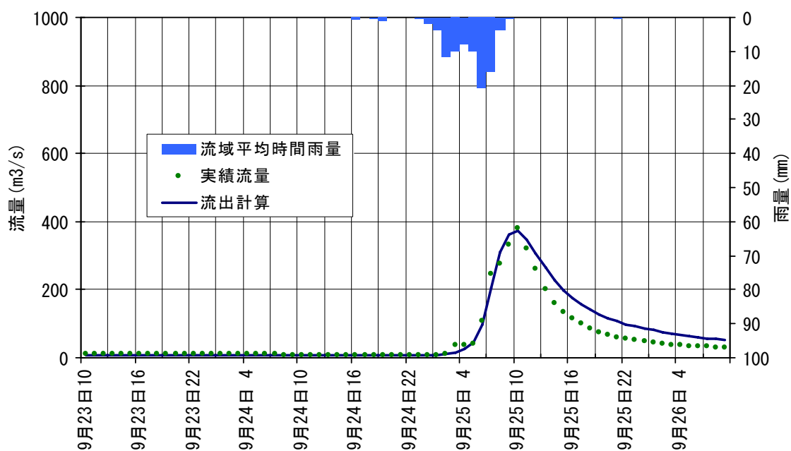
図 4-2 (2) 既往洪水の再現計算結果（広瀬川広瀬橋地点、昭和 41 年 9 月洪水）
