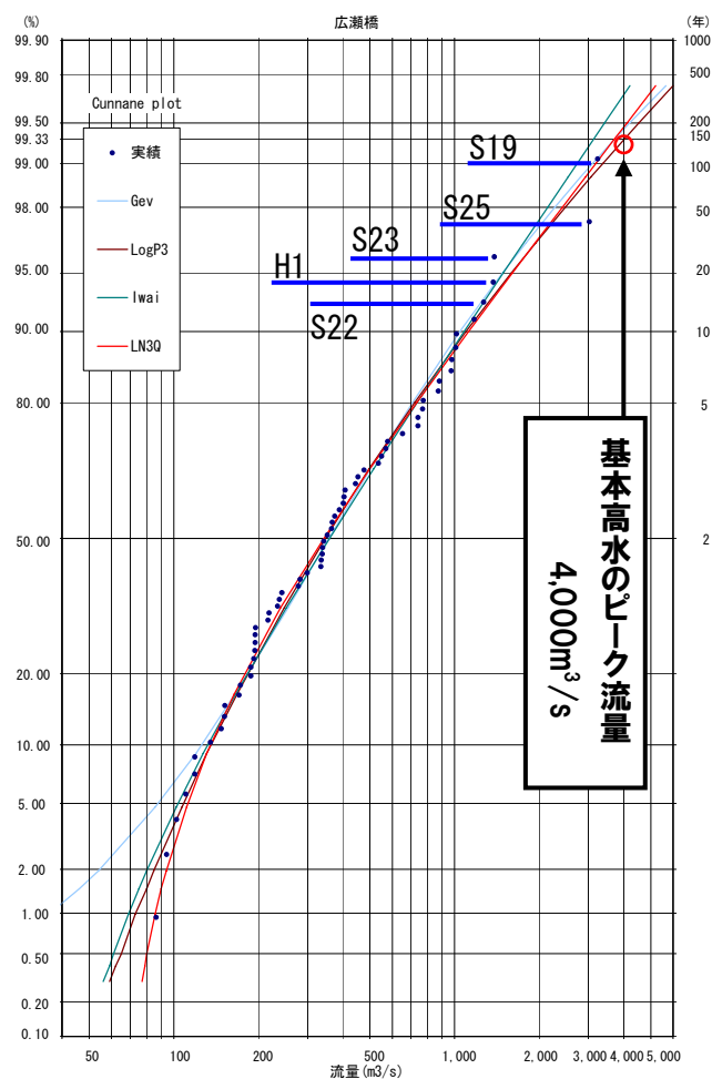
図 4-7(2) 広瀬川広瀬橋地点における流量確率図
