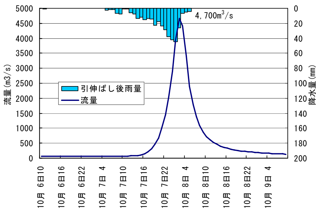
図 4-10 (1) 昭和 19 年 10 月型ハイドログラフ (名取川名取橋地点)
