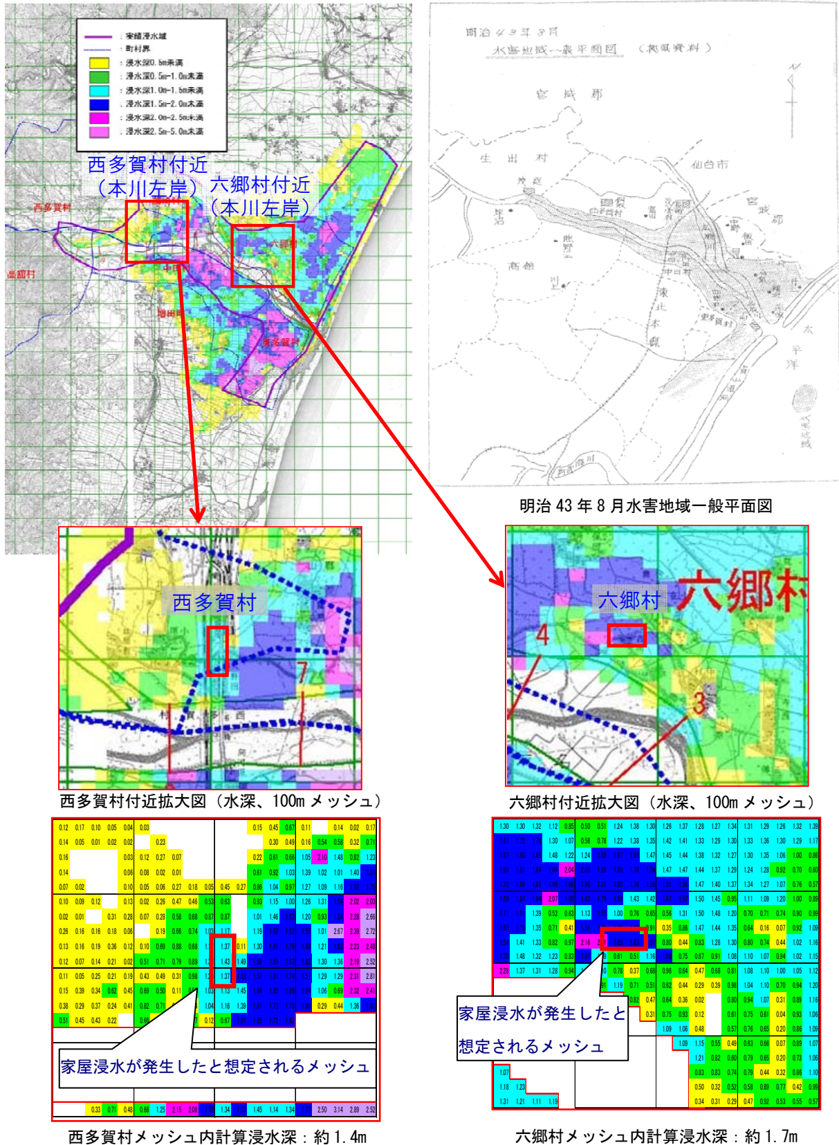
図 4-9 氾濫計算結果
