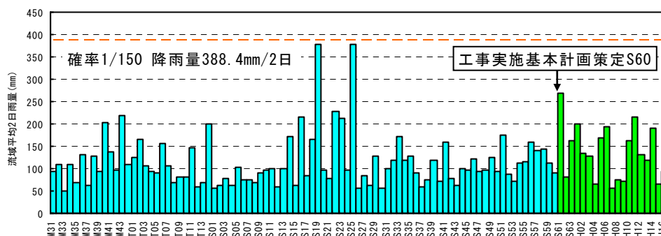
図 4-6 (1) 年最大 2 日雨量（広瀬川広瀬橋地点）
