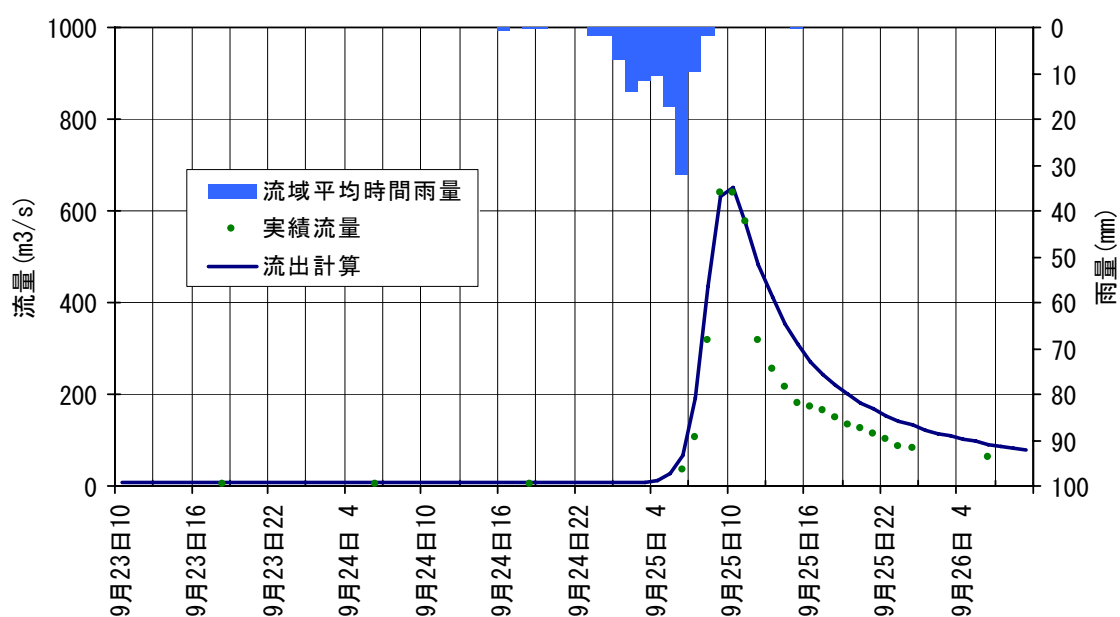
図 4-2 (1) 既往洪水の再現計算結果（名取川名取橋地点、昭和 41 年 9 月洪水）
