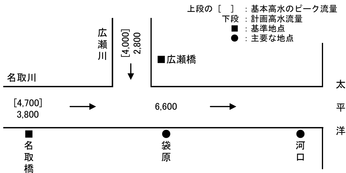
図 6-1 計画流量配分図
