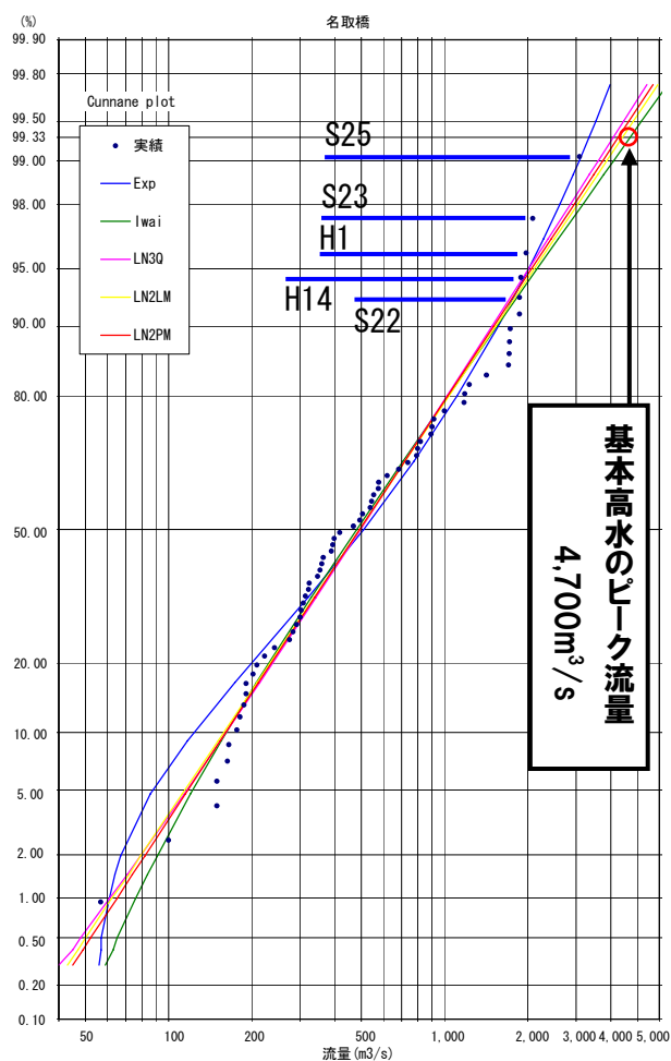
図 4-7(1) 名取川名取橋地点における流量確率図
