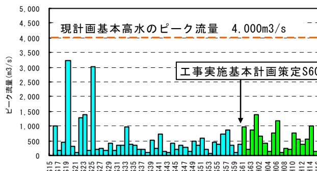
図 4-6 (2) 年最大流量（ダム・氾濫戻し流量、広瀬橋地点）
