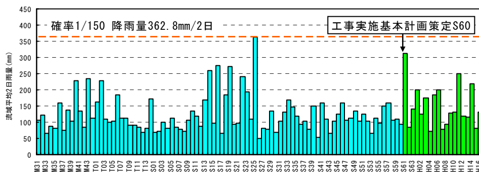
図 4-5 (1) 年最大 2 日雨量（名取川名取橋地点）
