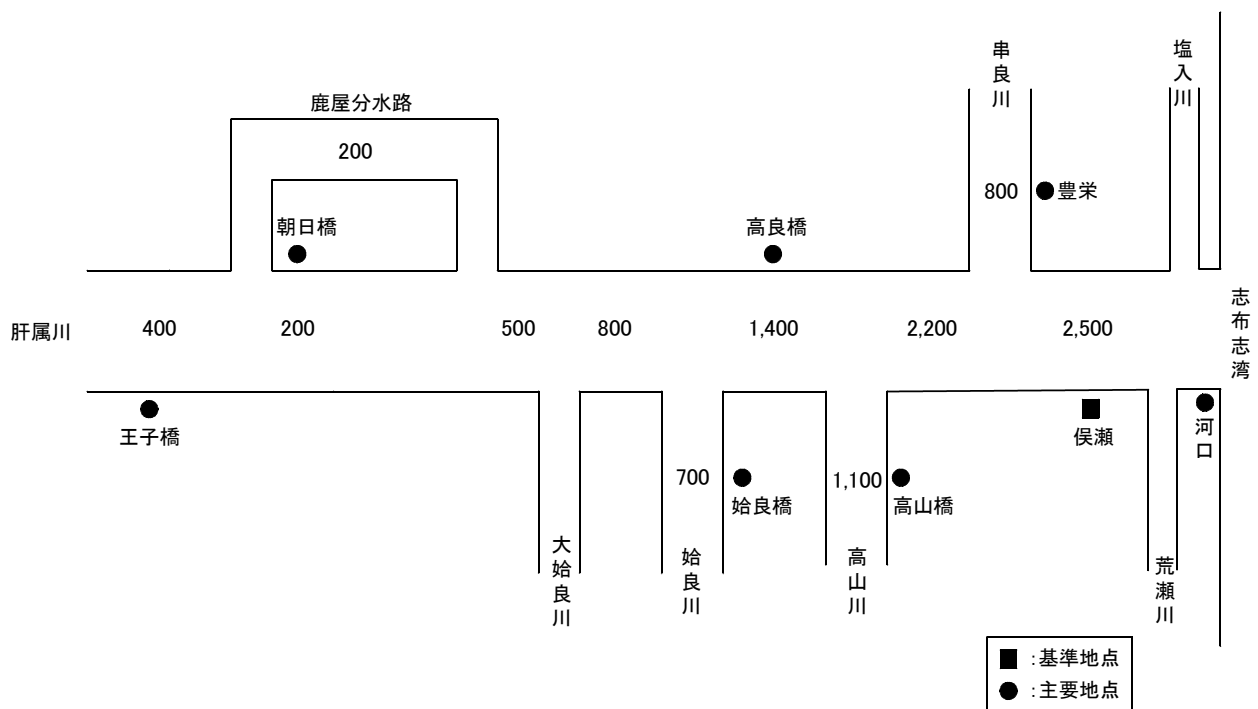
肝属川計画高水流量図
