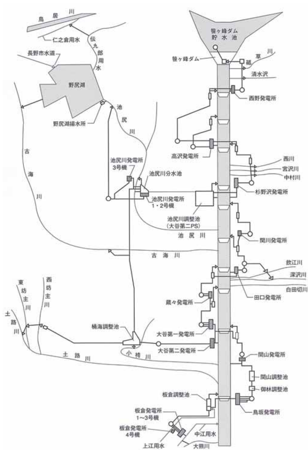
図 5-3 関川水系発電系統図（東北電力株式会社作成）
