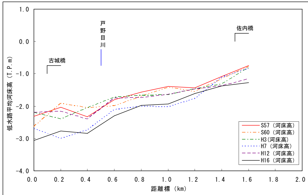
图 2-3 低水路平均河床高縦断図 (保倉川)
