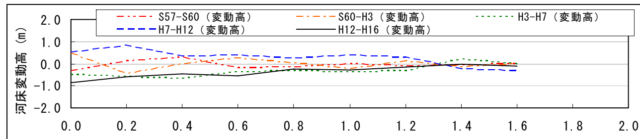
图 2-4 河床変動縦断図 (保倉川)
