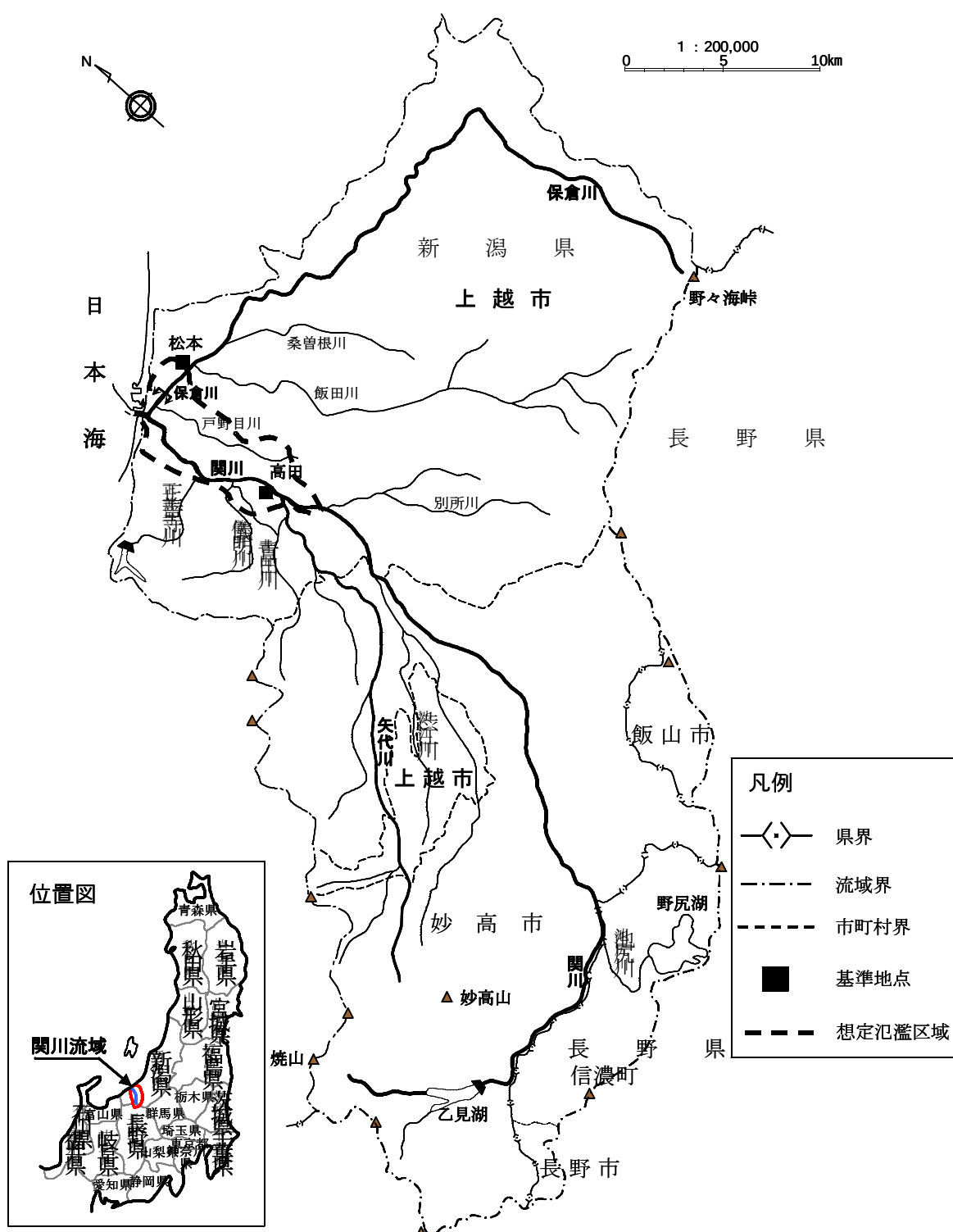
(参考図) 関川水系図
