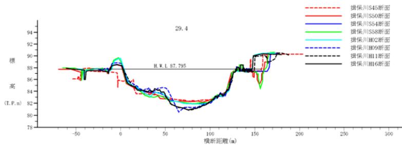
図 2-6 (3) 揖保川 中流部 (山崎大橋上流 29k4) 断面図
