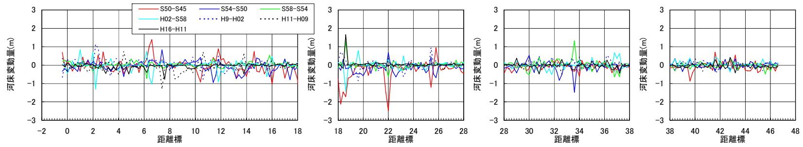
図2-2 河床変動縦断面図(揖保川)
