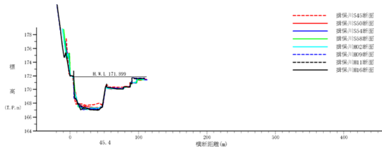
図 2-6 (4) 揖保川 上流部 (安積橋上流 45k2) 横断面図
