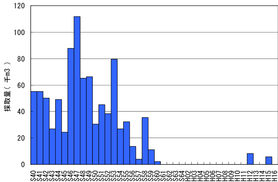
図 2-7 S40 以降の土砂採取量の経年変化
