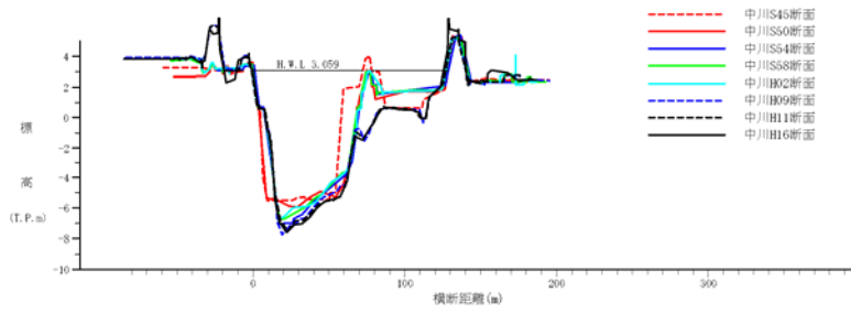
图 2-6 (5) 中川 (中川橋下流 1k2) 横断面
