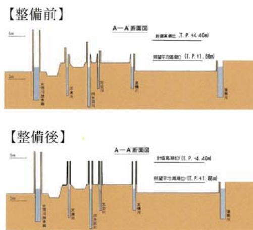
図-4.3.1 河口域(広島デルタ)地盤高図
