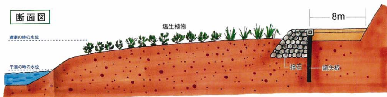
図-9.4.4 断面図
