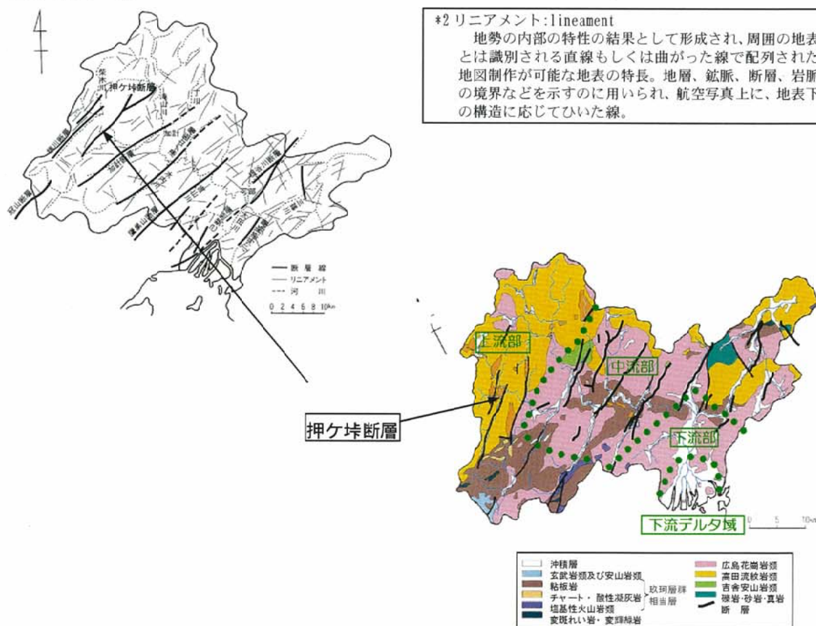
図-1.3.1 地質図
