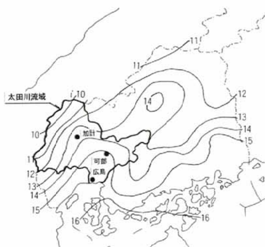
年平均気温(°C)の分布 (出典:広島県地方気象台「広島気象百年誌」)
