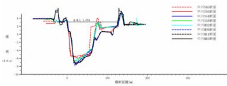
图 2-6 (5) 中川 (中川橋下流 1k2) 横断面
