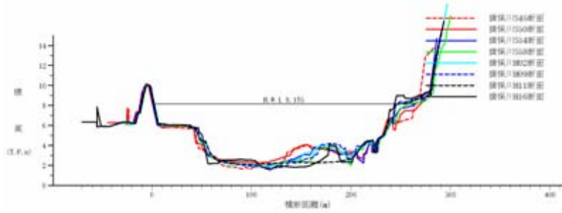
図 2-6 (1) 揖保川 河口部 (王子橋上流 4k2) 横断面図
