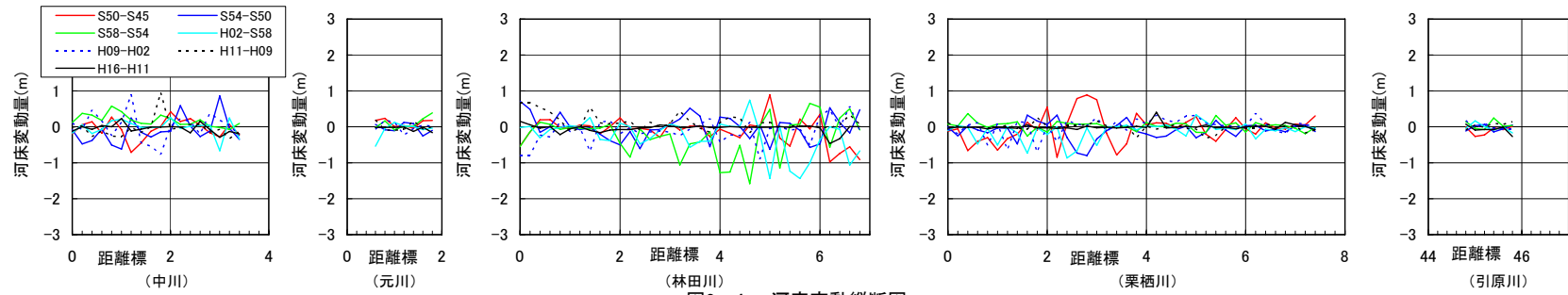
図2-4 河床変動縦断面図
