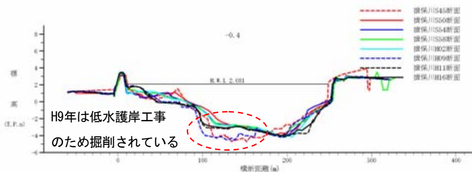
図 3-2 河口部 (-0k4) の横断面図
