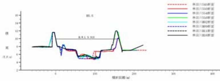
图 2-6 (7) 林田川 (真砂橋下流 0k6) 横断面
