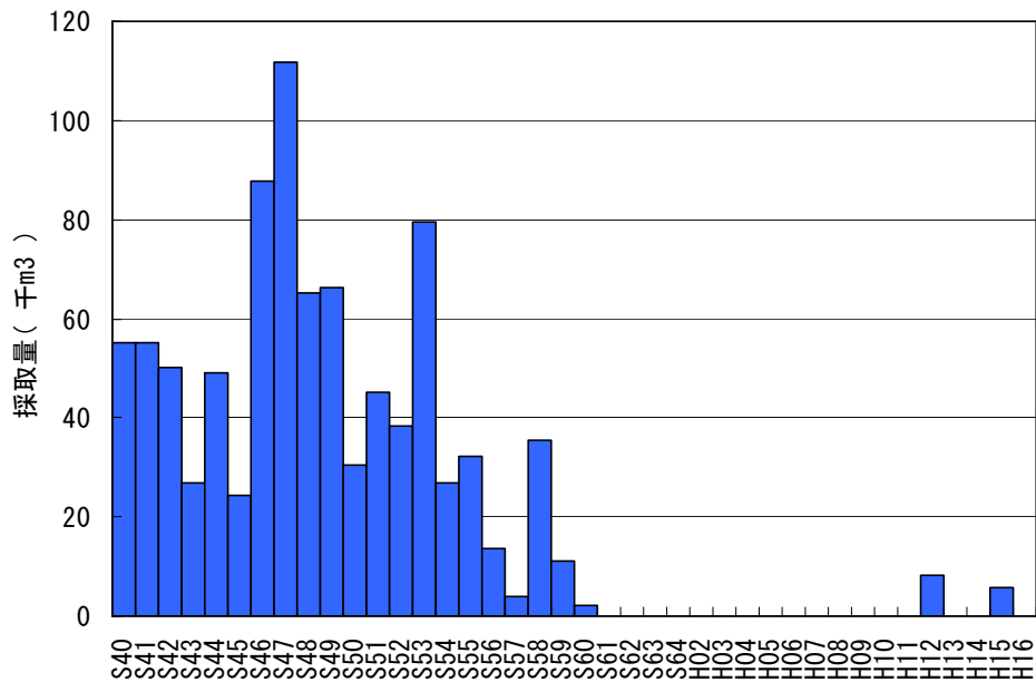
図 2-7 S40 以降の土砂採取量の経年変化
