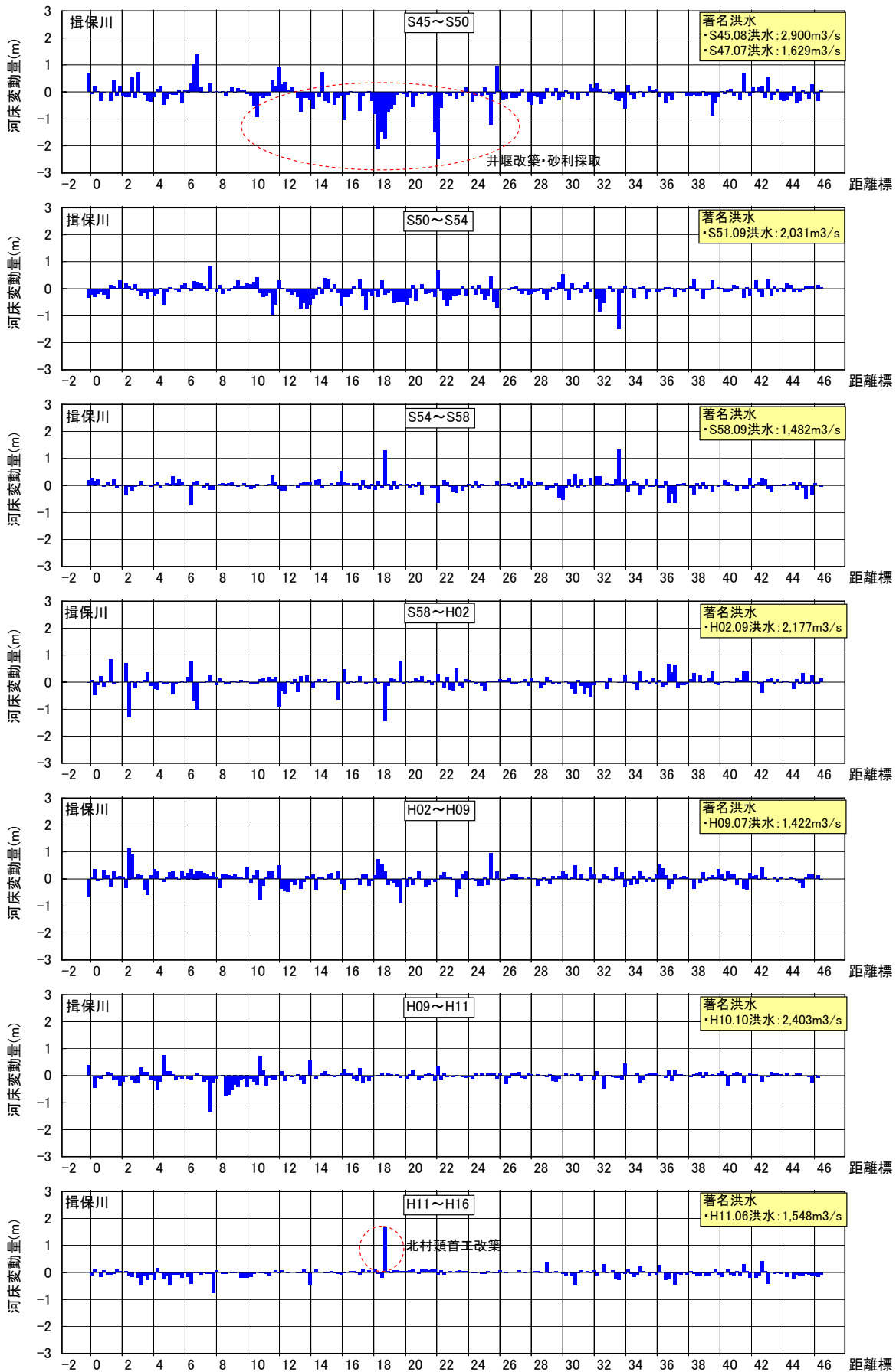
図 2-5 河床変動高の経年変化 (揖保川)
