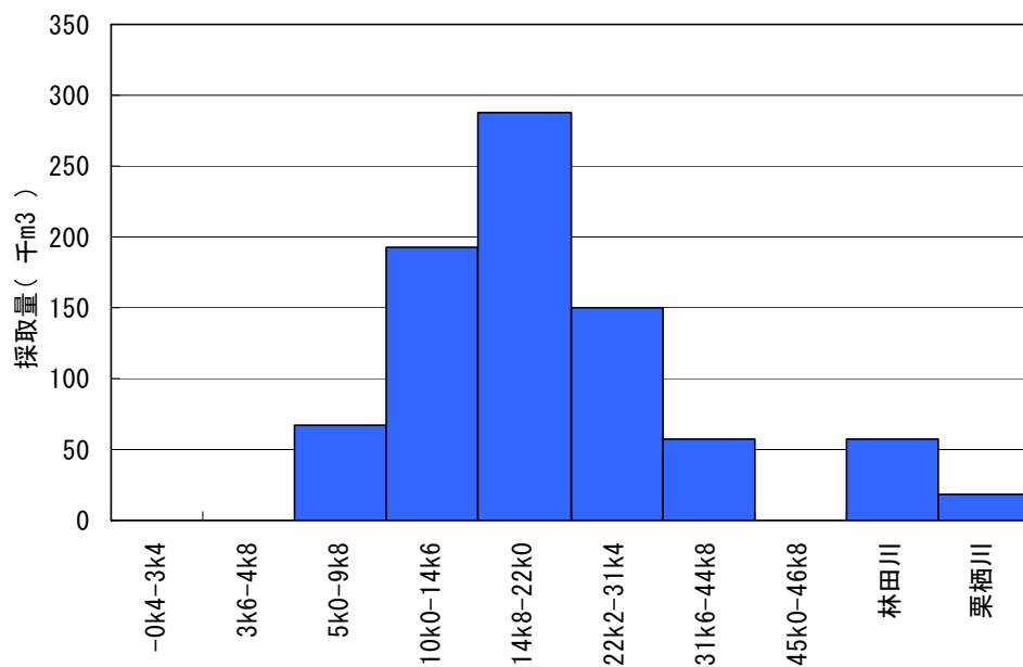
図 2-8 S40 以降の区間毎の土砂採取量
