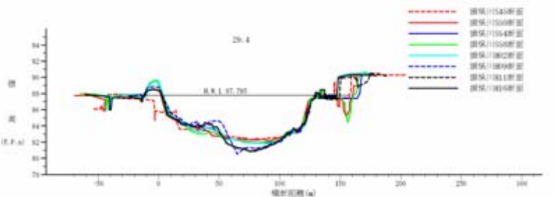
図 2-6 (3) 揖保川 中流部 (山崎大橋上流 29k4) 断面図
