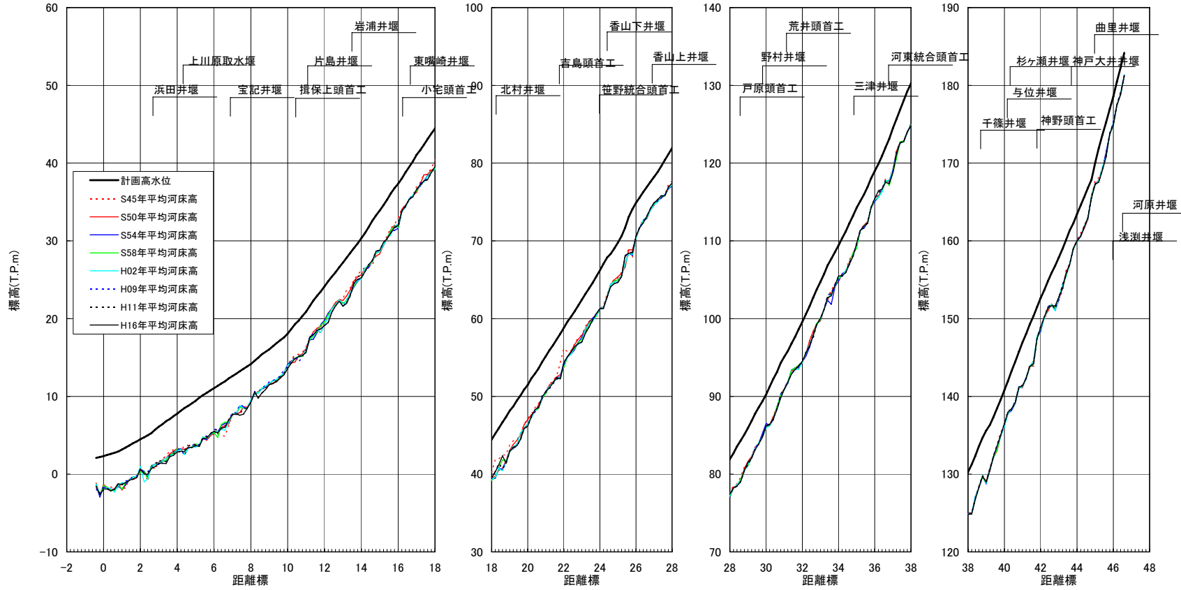
図2-1 低水路の平均河床縦断面図(揖保川)
