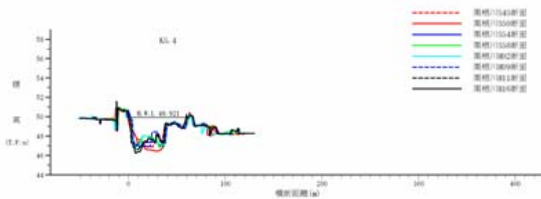
图 2-6 (8) 栗栖川 (芝田橋上流 5k4) 横断面
