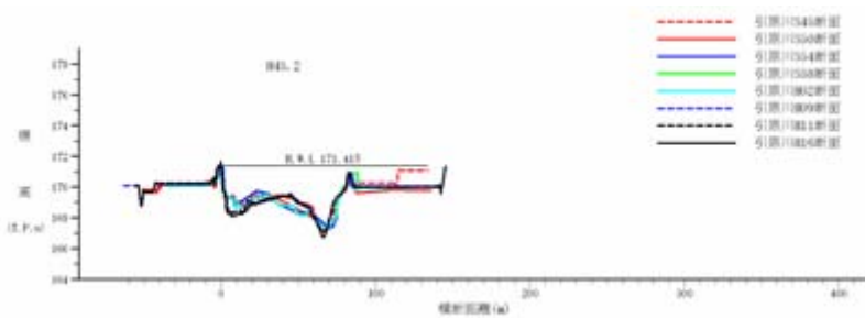
图 2-6 (9) 引原川 (西安積橋下流 45k2) 横断面
