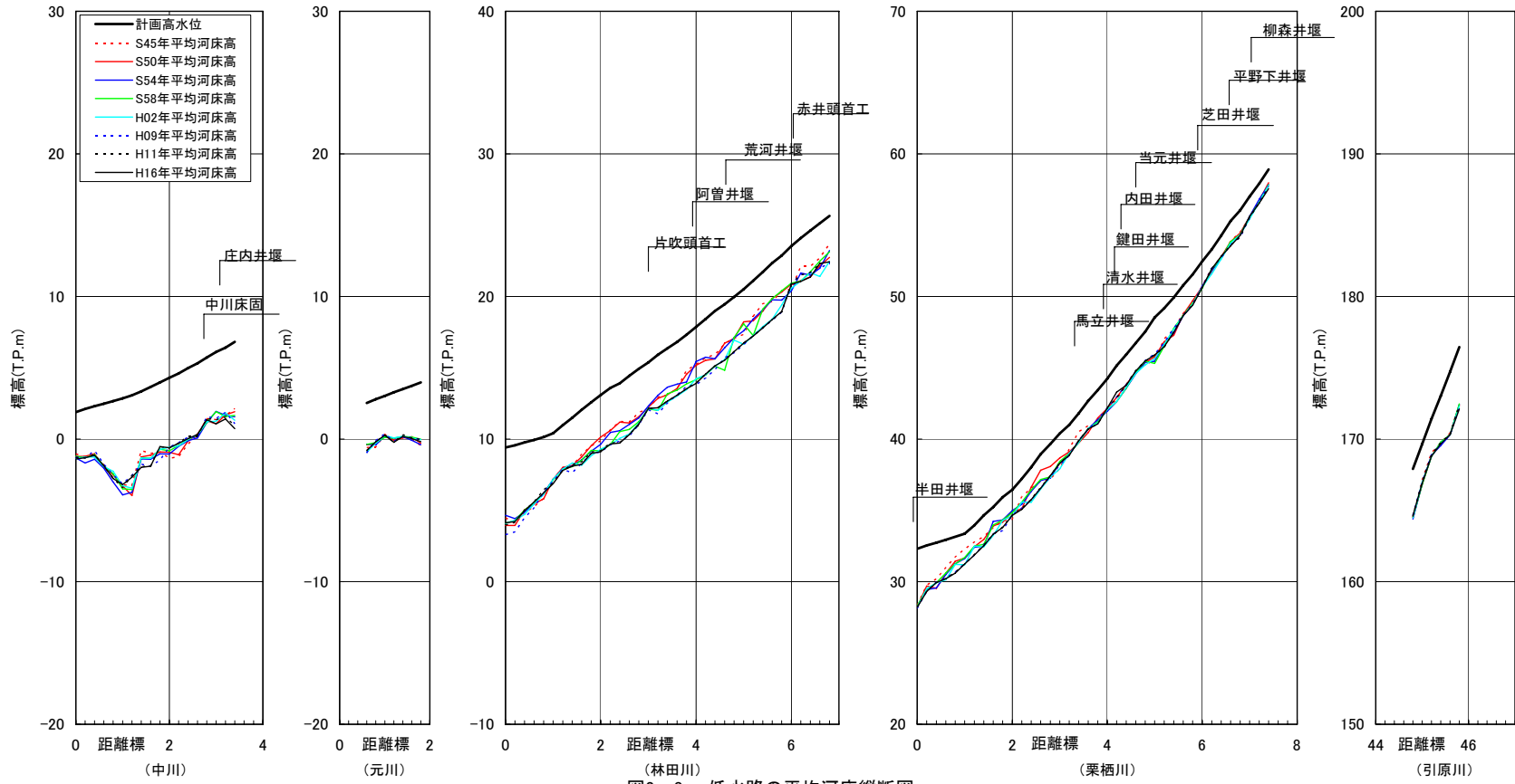
図2-3 低水路の平均河床縦断面図
