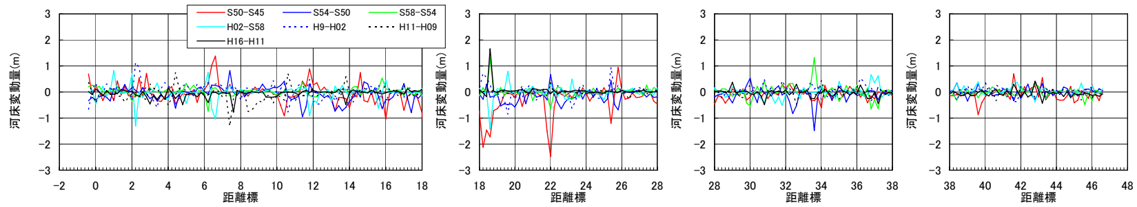
図2-2 河床変動縦断面図(揖保川)
