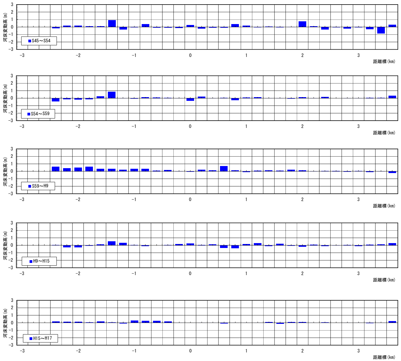
図 2-8(1) 低水路内河床變動量経年変化図(市内派川：天満川)
