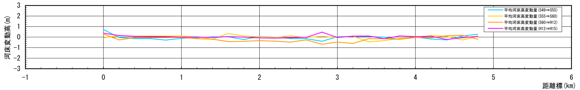
图 2-6(4) 河床変動縦断図(支川：根谷川)
