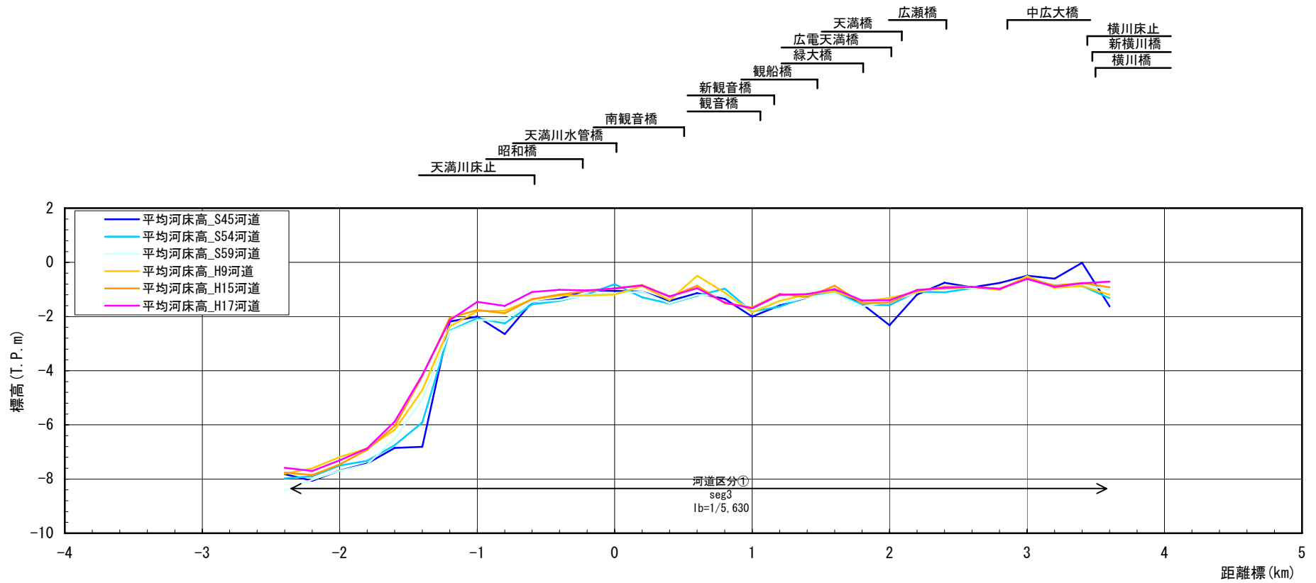
図 2-3(1) 低水路平均河床高縦断図(市内派川：天満川)
