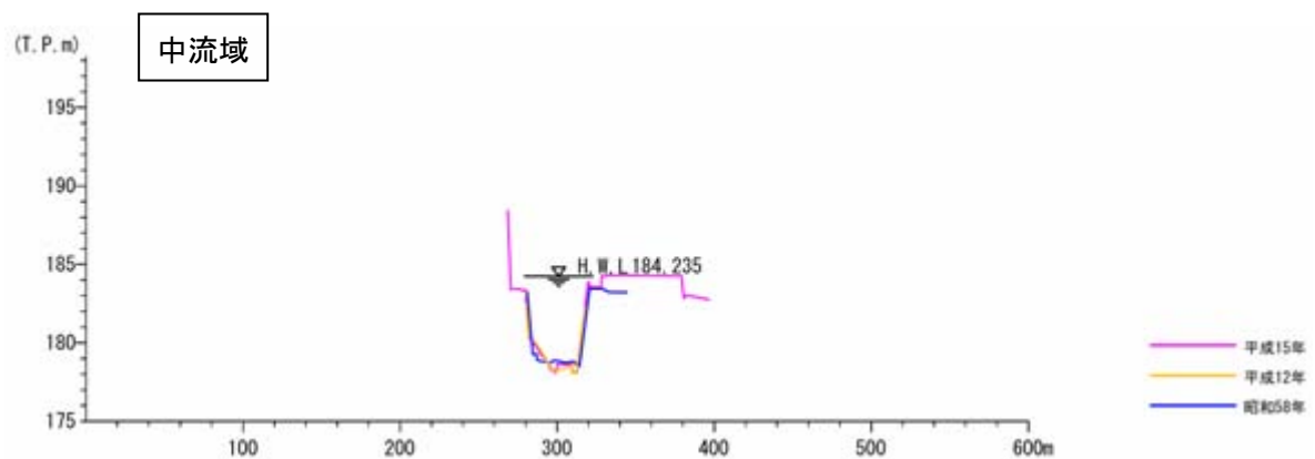
図 2-12 (6) 経年変化横断面図(支川：中祖川)
