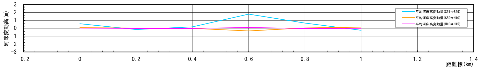
図 2-6(2) 河床変動縦断図(支川：第 2 古川)
