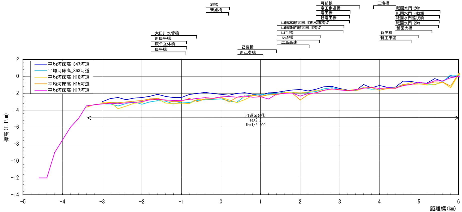
図 2-1 (1) 低水路平均河床高縦断図(太田川本川 : -3K400~6K000)
