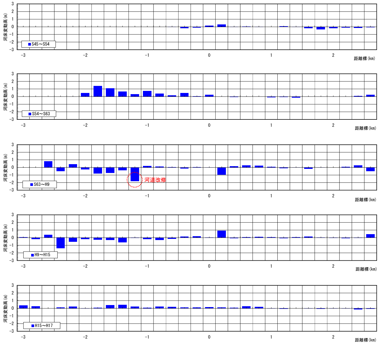
圖 2-8 (3) 低水路内河床變動量經年變化圖(市内派川：元安川)
