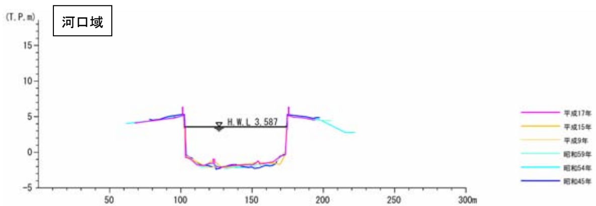
図 2-11 (1) 経年変化横断面図(市内派川：天満川)
