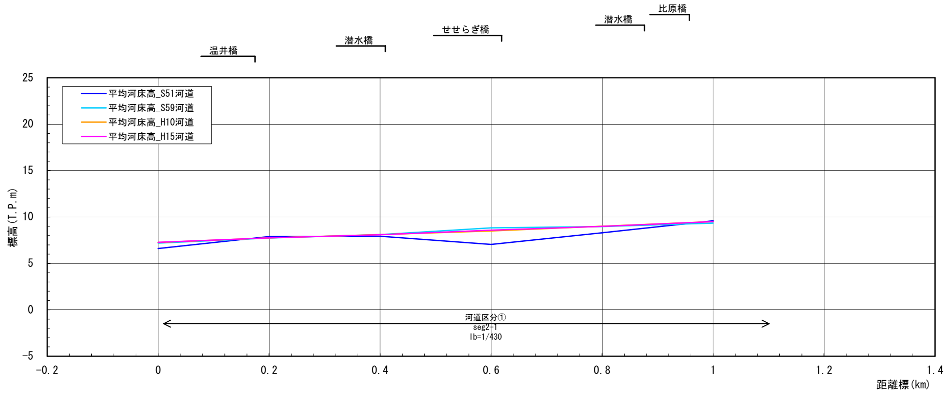
図 2-5(2) 低水路平均河床高縦断図(支川：第 2 古川)
