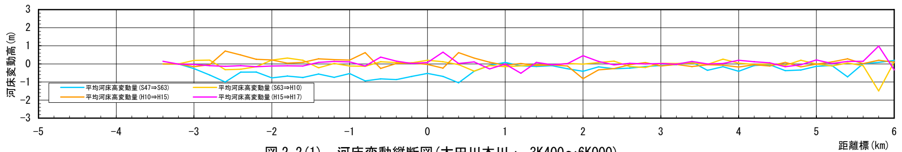
図 2-2 (1) 河床変動縦断図(太田川本川 : -3K400~6K000)
