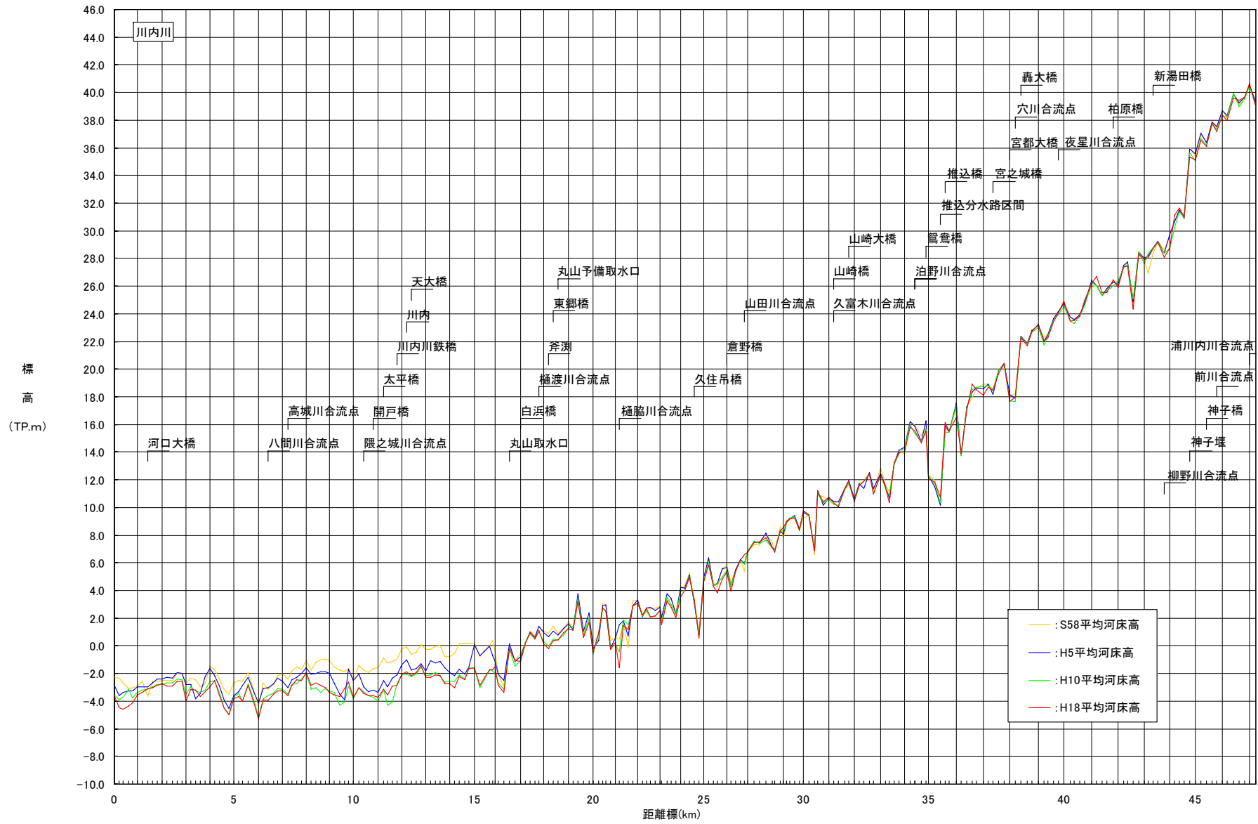
図 2-1 (1) 平均河床高縦断図 (川内川中下流区間)
