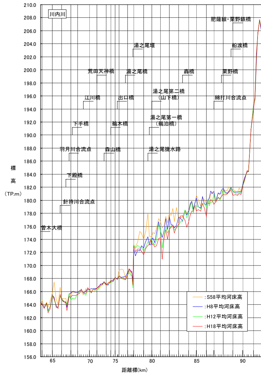
図 2-1 (2) 平均河床高縦断図 (川内川上流区間)
