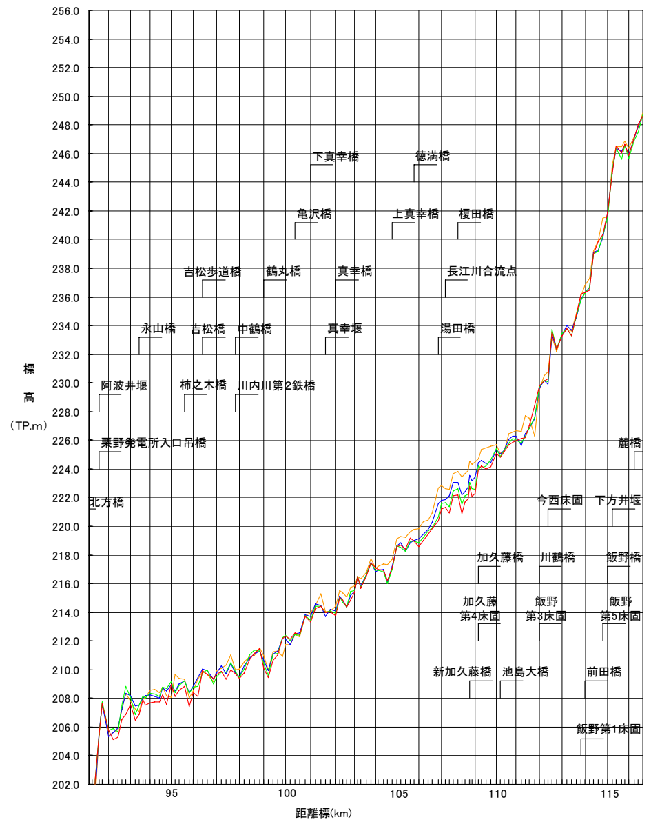
図 2-1 (2) 平均河床高縦断図 (川内川上流区間)
