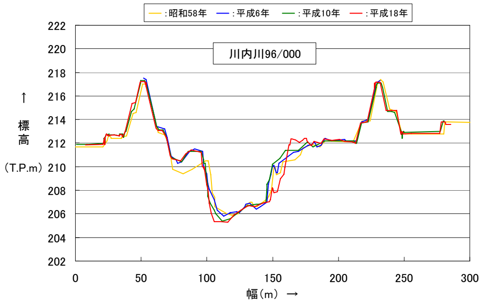
図 2-3 (3) 代表横断面図 (川内川 96/000 : 吉松)
