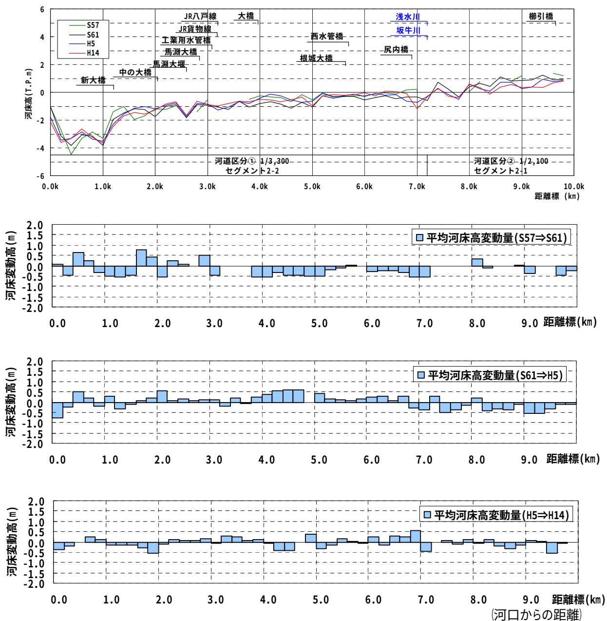
図 8-2 馬淵川の河床変動の経年変化
