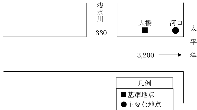
馬淵川計画高水流量図 (単位：m 3 /s)
