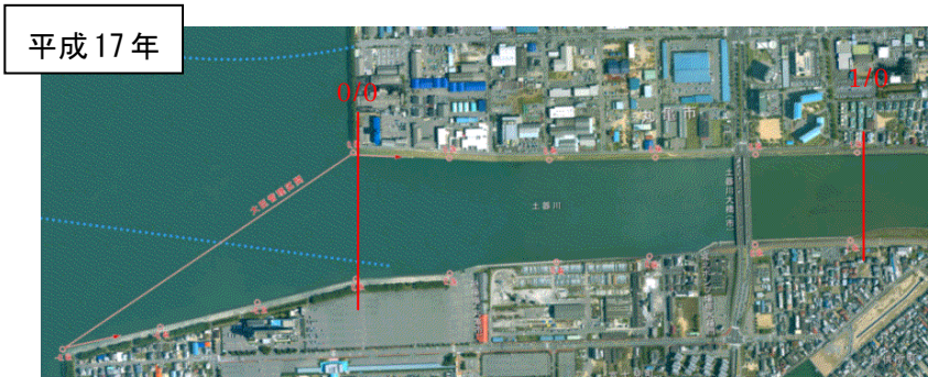
図 3-2 河口形状の経年変化
