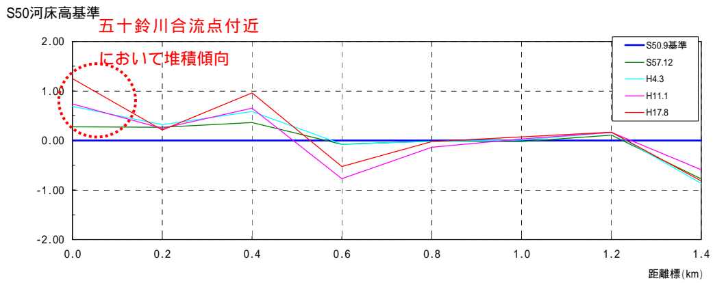
図 2 - 9 大湊川平均河床高縦断面図
