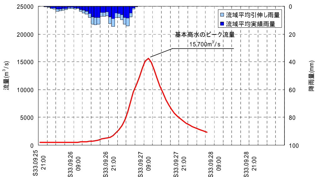
図-4-15 基本高水ハイドログラフ(昭和 33 年 9 月 26 日型 : 1/150 : 馬下)
