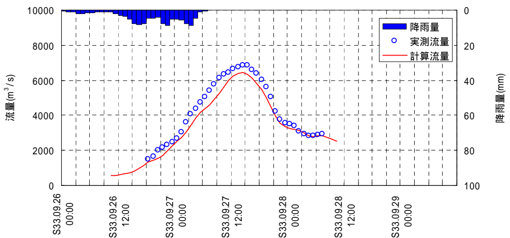
図 4-3 昭和 33 年 9 月 26 日洪水再現計算結果(馬下地点)
