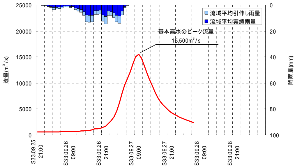
図 4-7 阿賀野川馬下地点基本高水決定洪水ハイドログラフ(昭和 33 年 9 月 26 日型)
