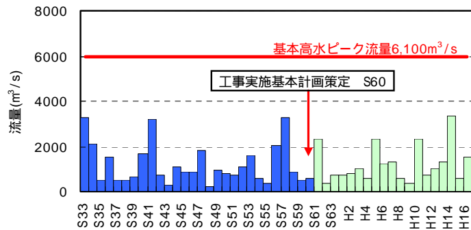
図 4-9 阿賀川山科地点 年最大流量(S33 ~ H16)
