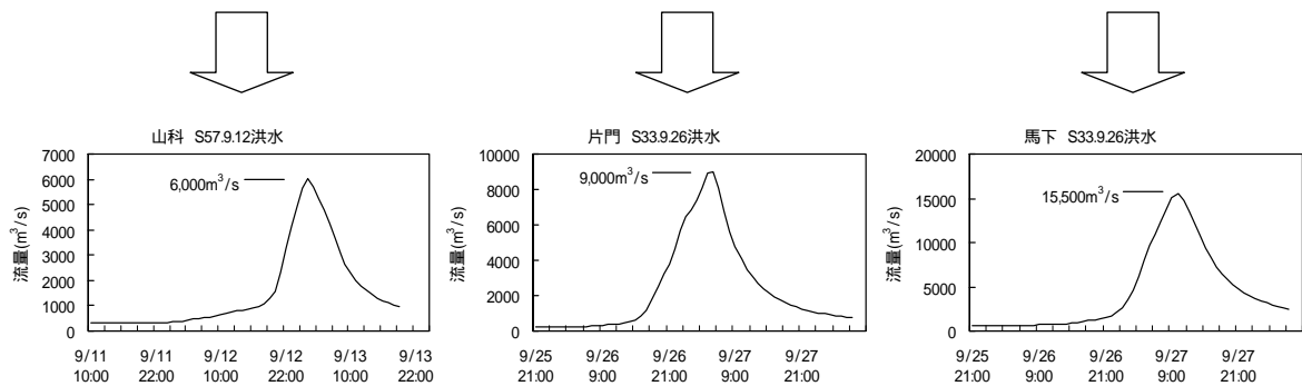
図 4-4 主要洪水における計画降雨量への引伸しと流出計算
