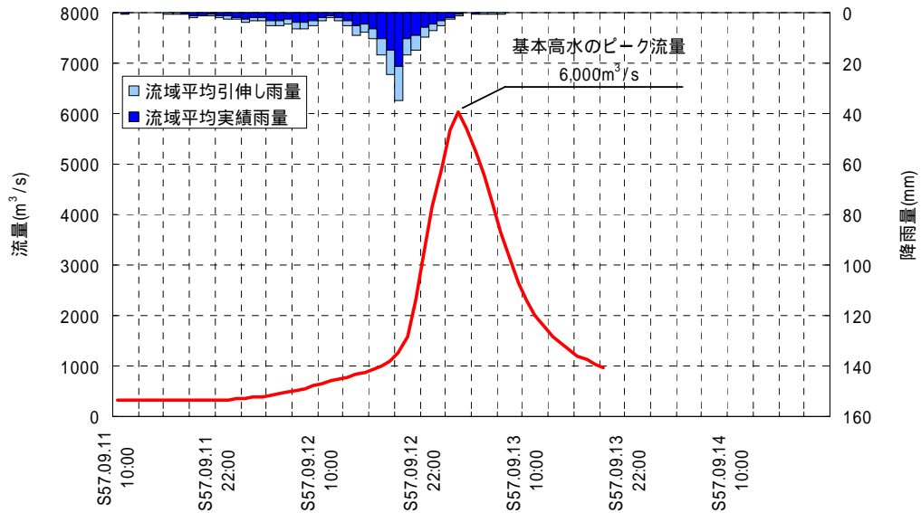
図 4-5 阿賀川山科地点基本高水決定洪水ハイドログラフ(昭和 57 年 9 月 12 日型)
