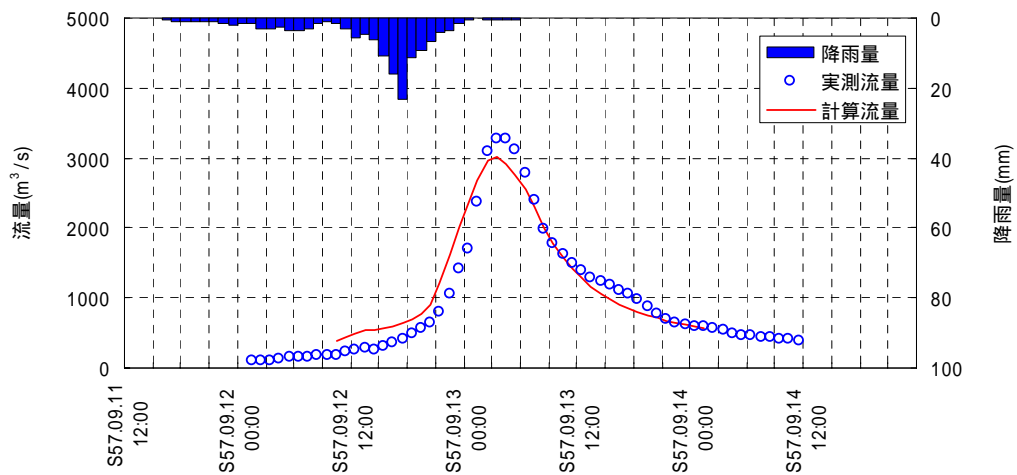
図 4-2 昭和 57 年 9 月 12 日洪水再現計算結果(山科地点)
