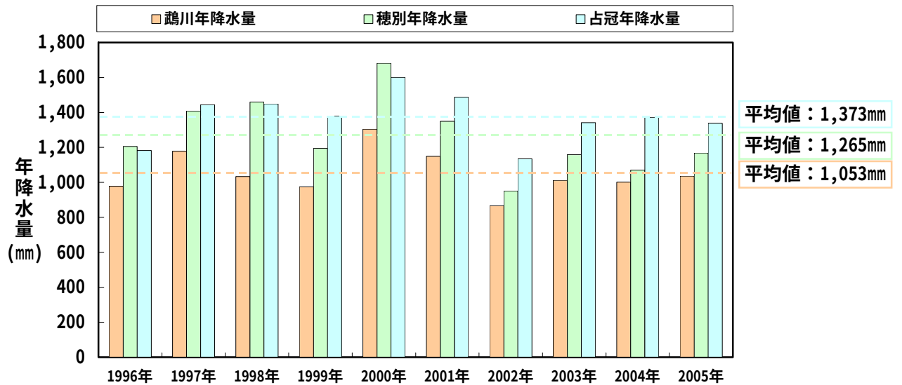
図 1-6 年降水量
