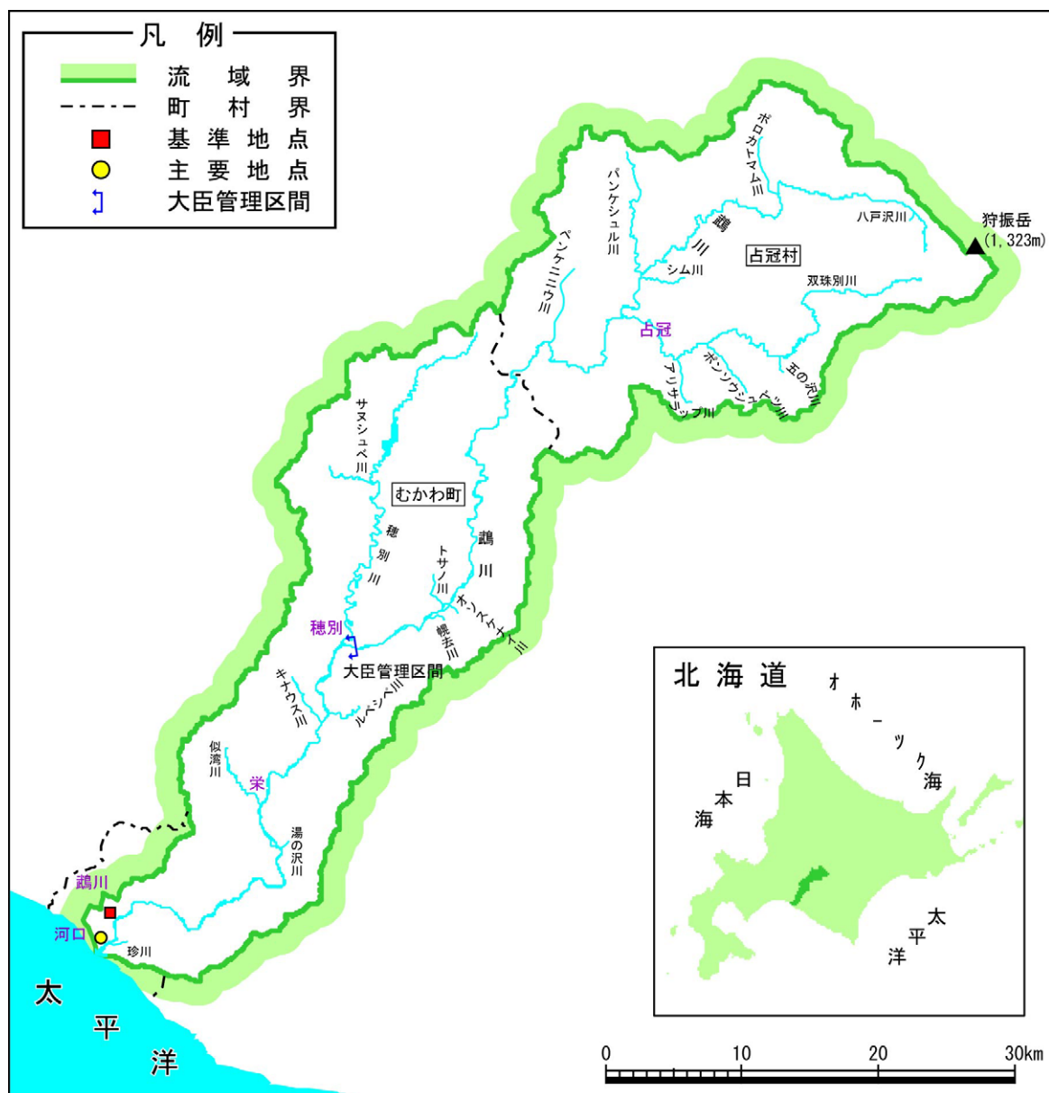
図 1-1 鵡川流域図
