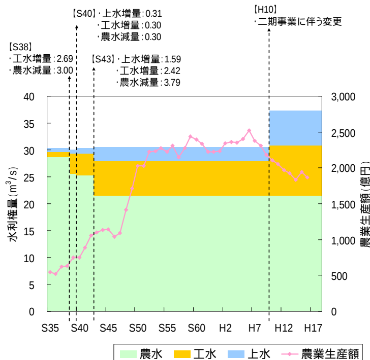
図 5.1.8 愛知用水の水利権量と木曽川水系水供給区域における農業生産額の推移
