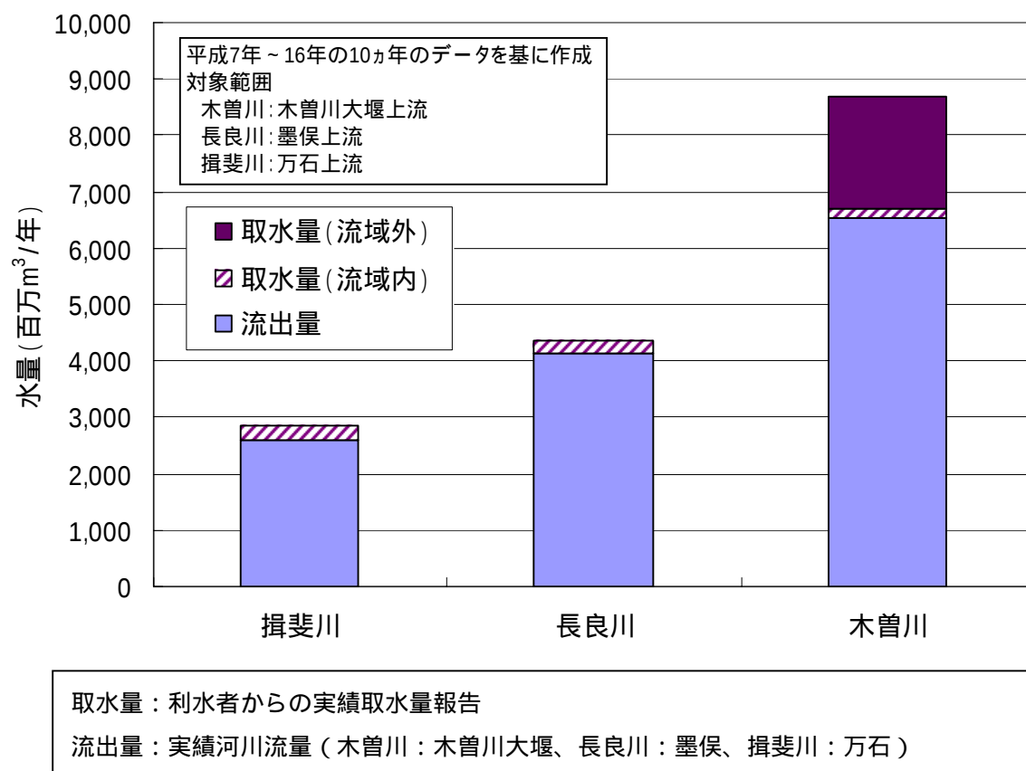
図 5.1.19 木曽川水系の年総流出量と取水量
