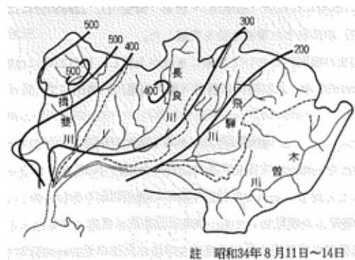
図 4.1.1 木曽三川総雨量分布図
