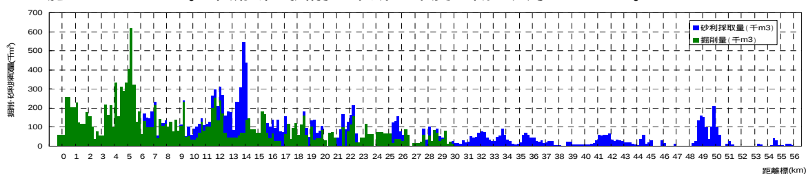
図8.2.10 掘削および砂利採取量
