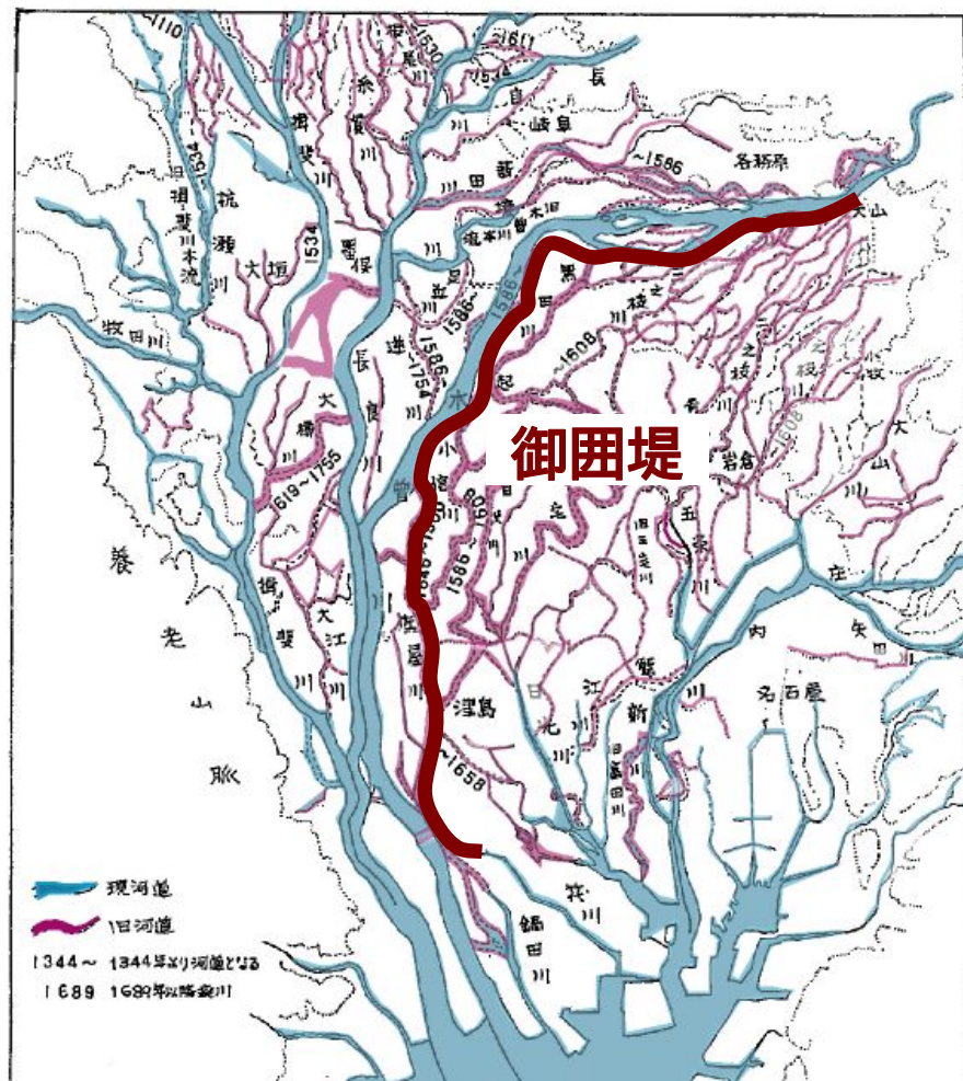
図 5.1.2 御囲堤の位置
