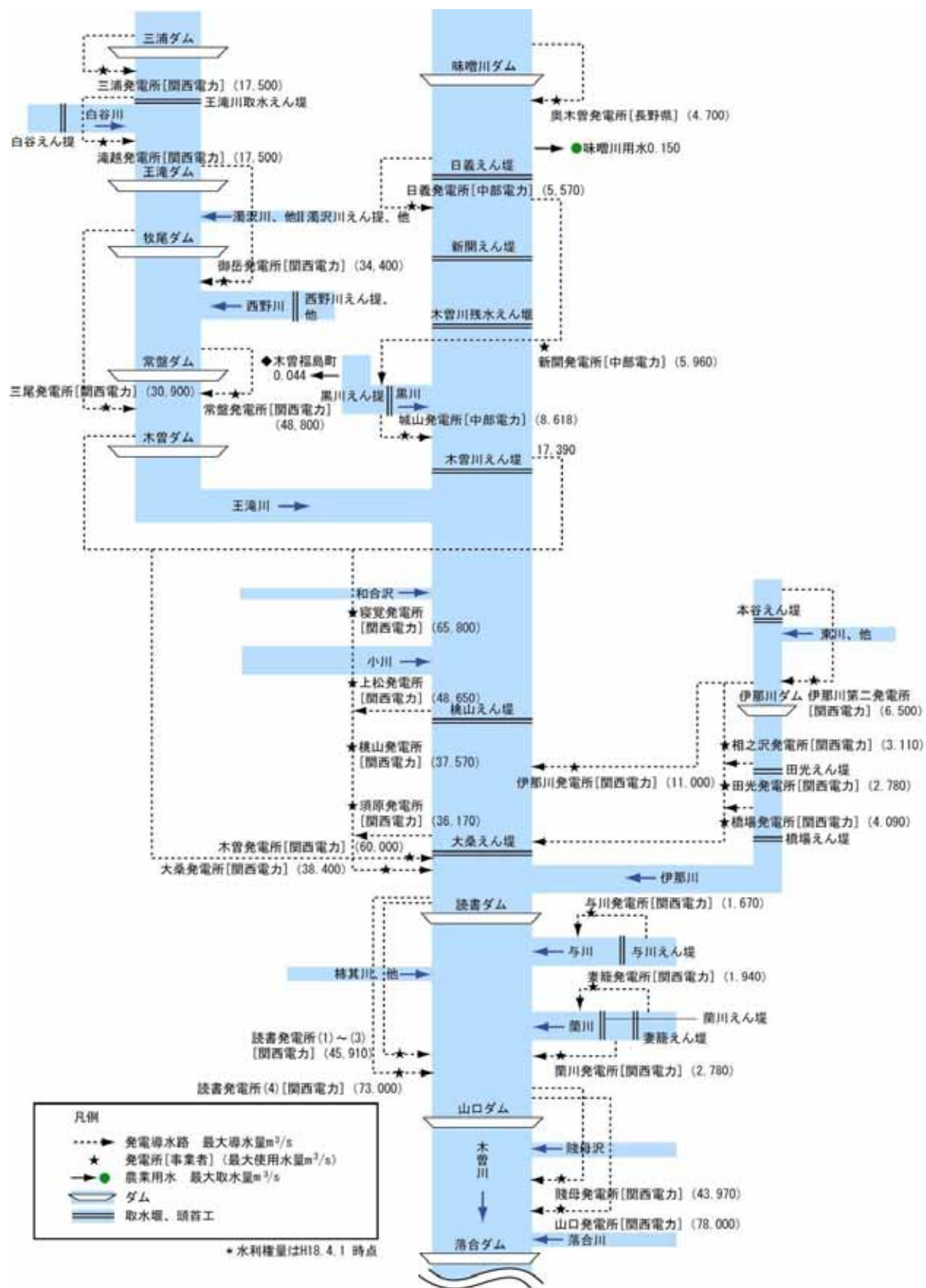
図 5.1.14(3) 木曽川水系木曽川 水利使用模式図 (3/3)(主要な水利権を記載) (単位: m^3/s )
