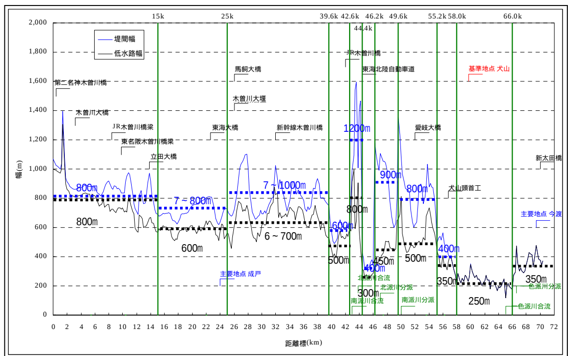
図 8.1.2 木曽川の堤間幅・低水路幅
