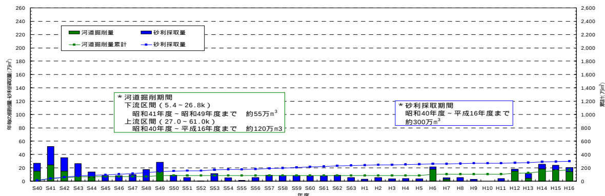
図8.2.17 掘削および砂利採取量
