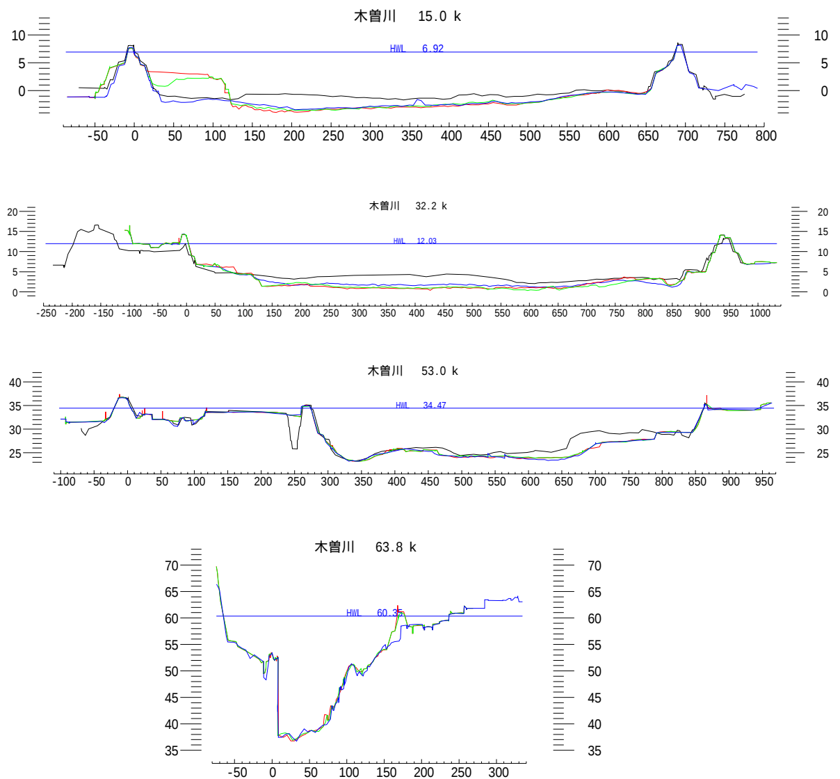
図8.2.6 河道横断形状の経年変化
