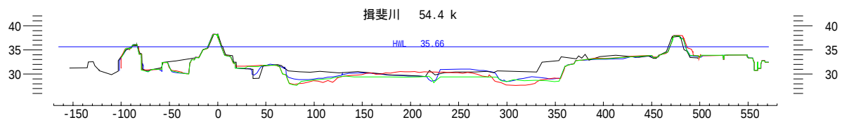
図8.2.18 河道横断形状の経年変化
