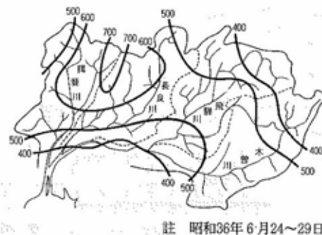
図 4.1.5 木曽三川総雨量分布 出典：木曽三川治水百年のあゆみ
