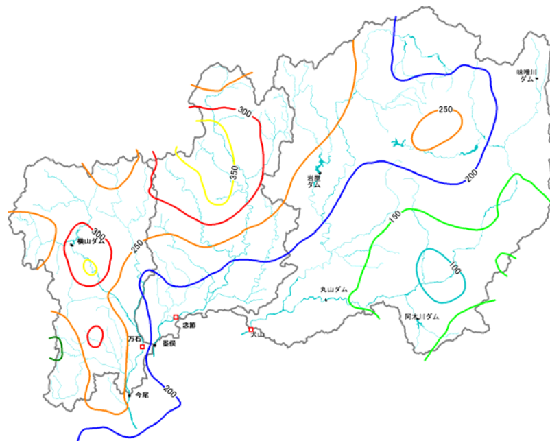
図 4.1.8 H16.10 洪水等雨量線図
