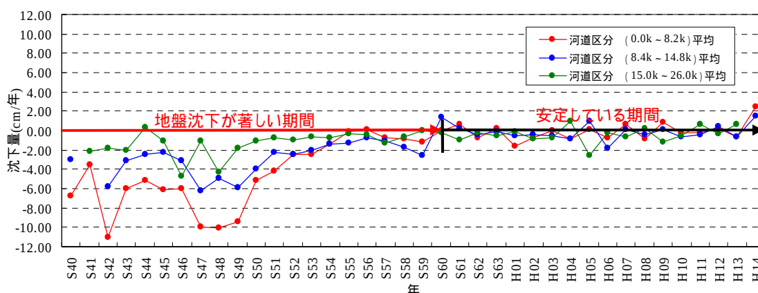
図8.2.3 河道の沈下量の変化
