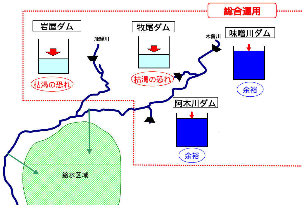
図 5.2.2 総合運用図
