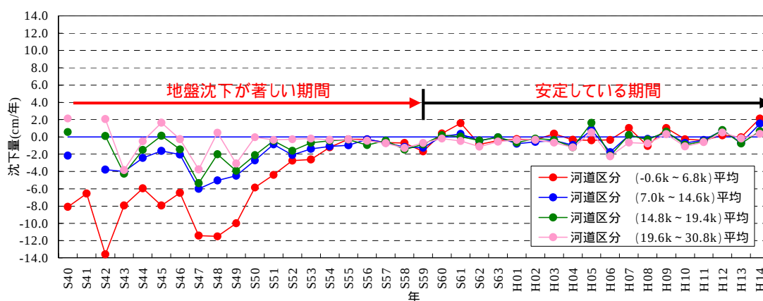
図8.2.9 河道の沈下量の変化
