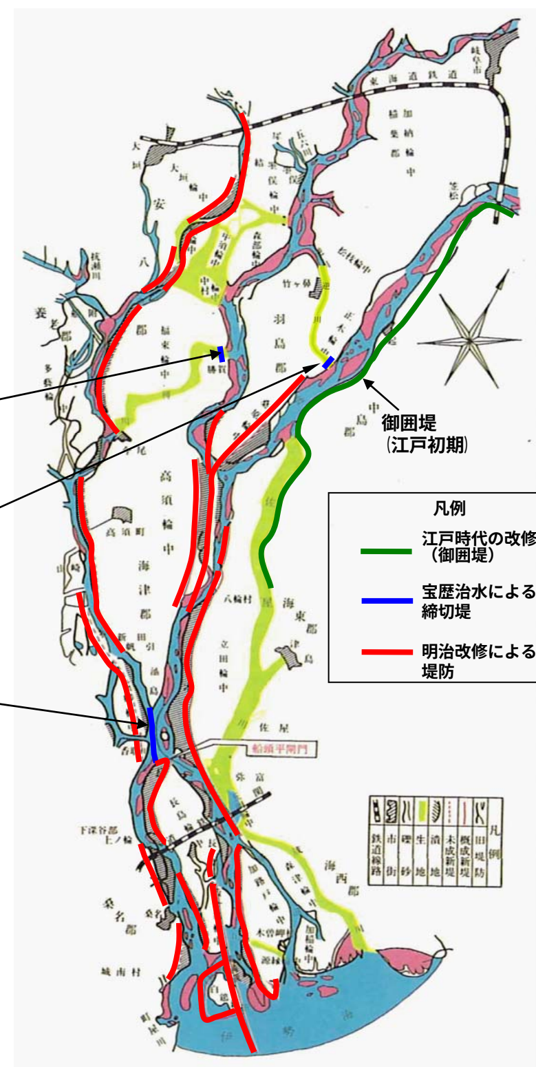
江戸時代～明治改修図
