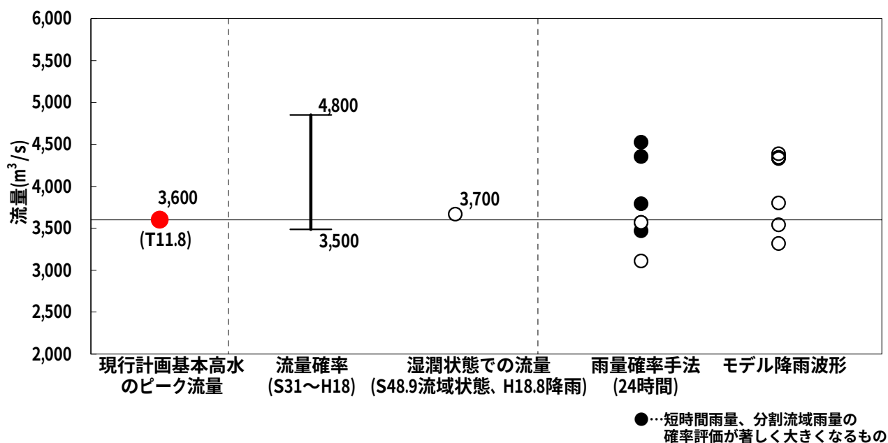
図 4-7 各手法による基本高水のピーク流量算定結果
