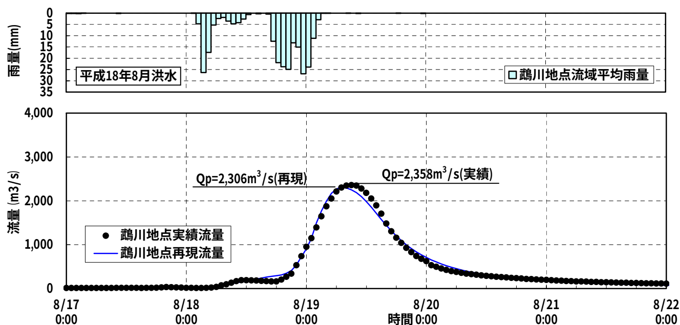
図 4-5 流出計算モデル再現ハイドログラフ(鵜川地点、平成 18 年 8 月洪水)
