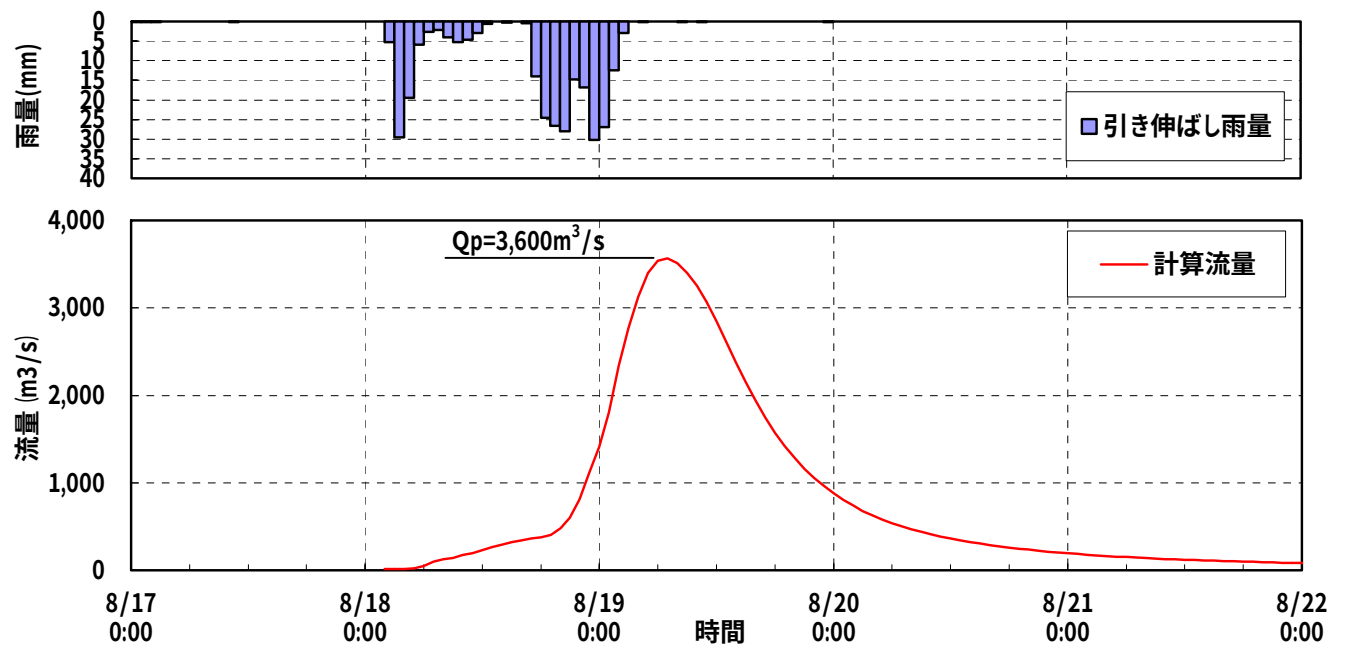
図 4-8 引伸ばし降雨によるハイドログラフ(鵜川地点 平成 18 年 8 月型降雨)
