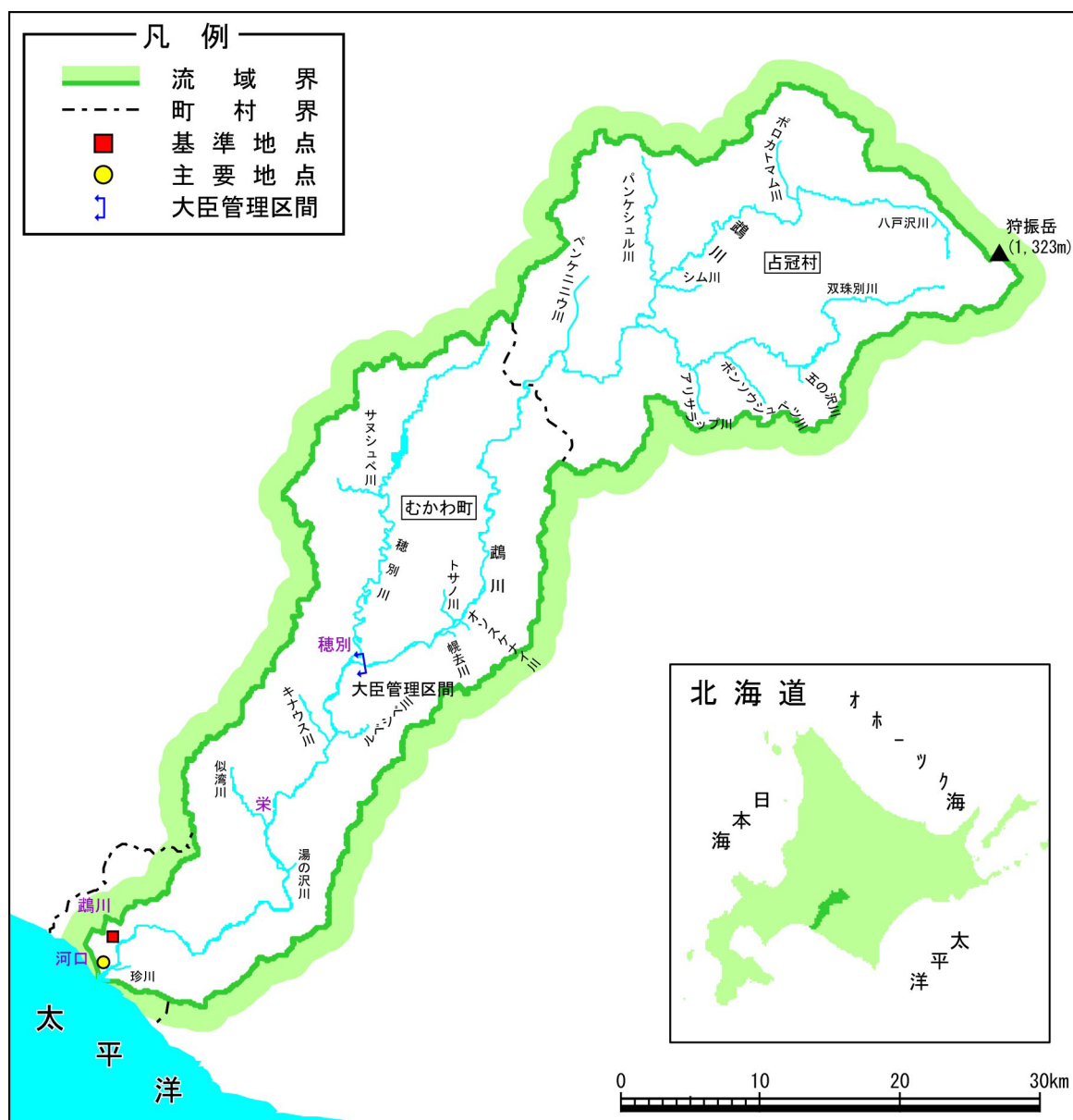
図 1-1 鵠川水系流域図
