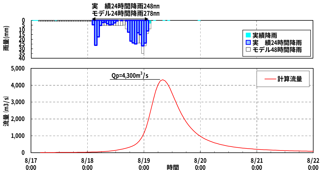
図 4-6 1/100 モデル降雨波形による流出計算結果(鵜川地点)
