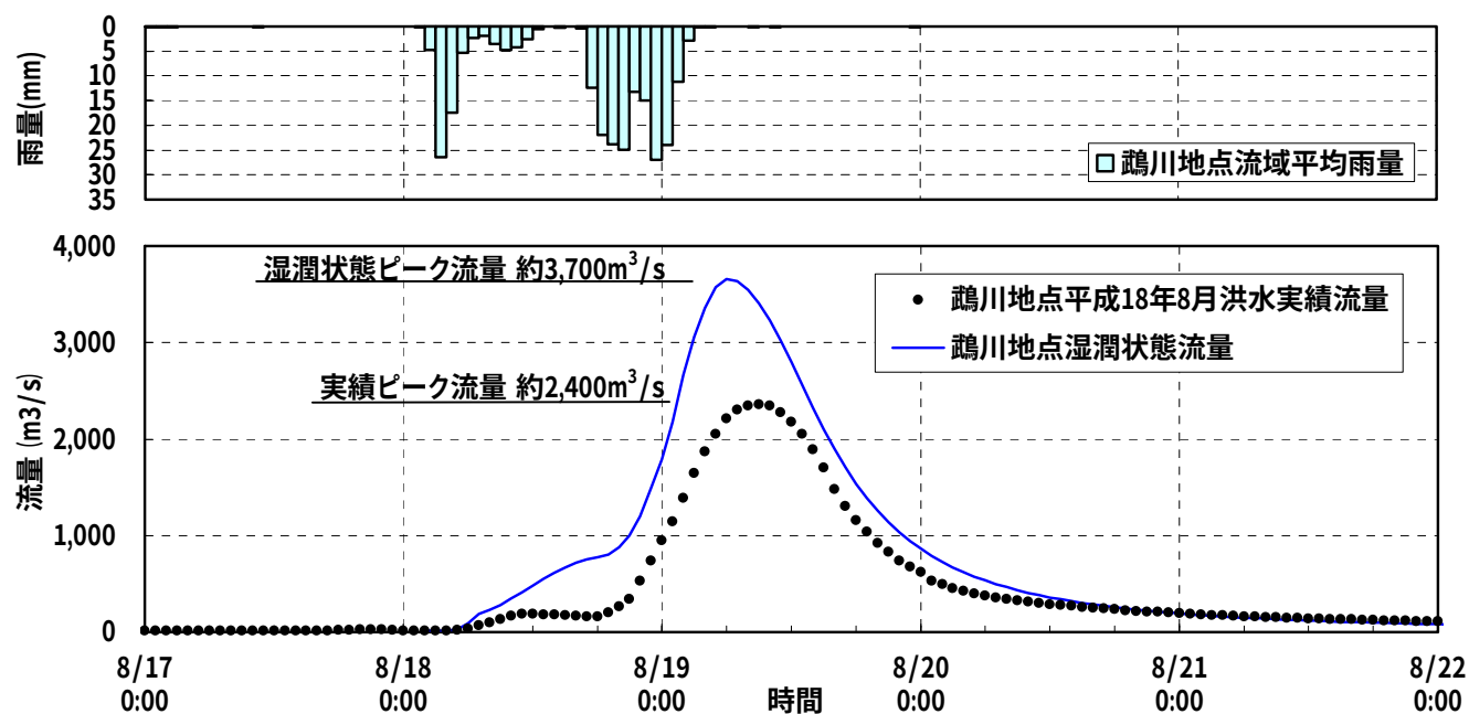
図 4-3 平成 18 年 8 月洪水ハイドロ・ハイトグラフ (昭和 48 年 9 月洪水流域湿潤状態)
