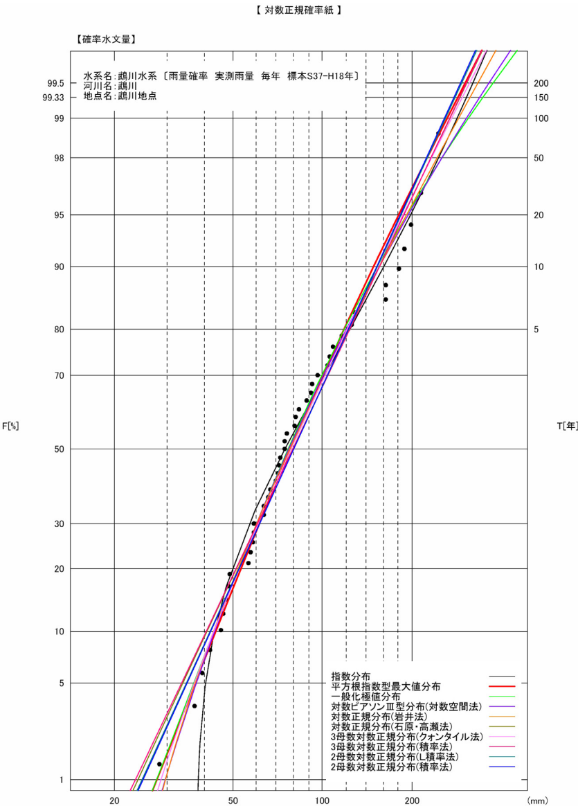
図 4-4 鵜川地点における雨量確率評価(昭和 37 年～平成 18 年:45 カ年)
