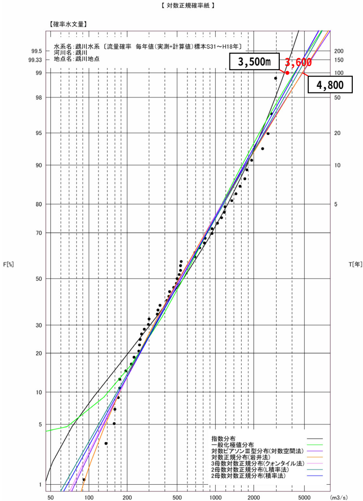
図 4-2 鷗川地点流量確率図(S31~H18:51 年間)
