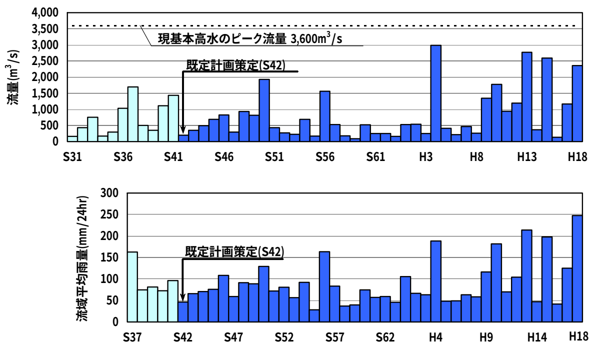
図 4-1 鵜川地点年最大流量と鵜川地点年最大流域平均 24 時間雨量(冬期、融雪期を除く)
