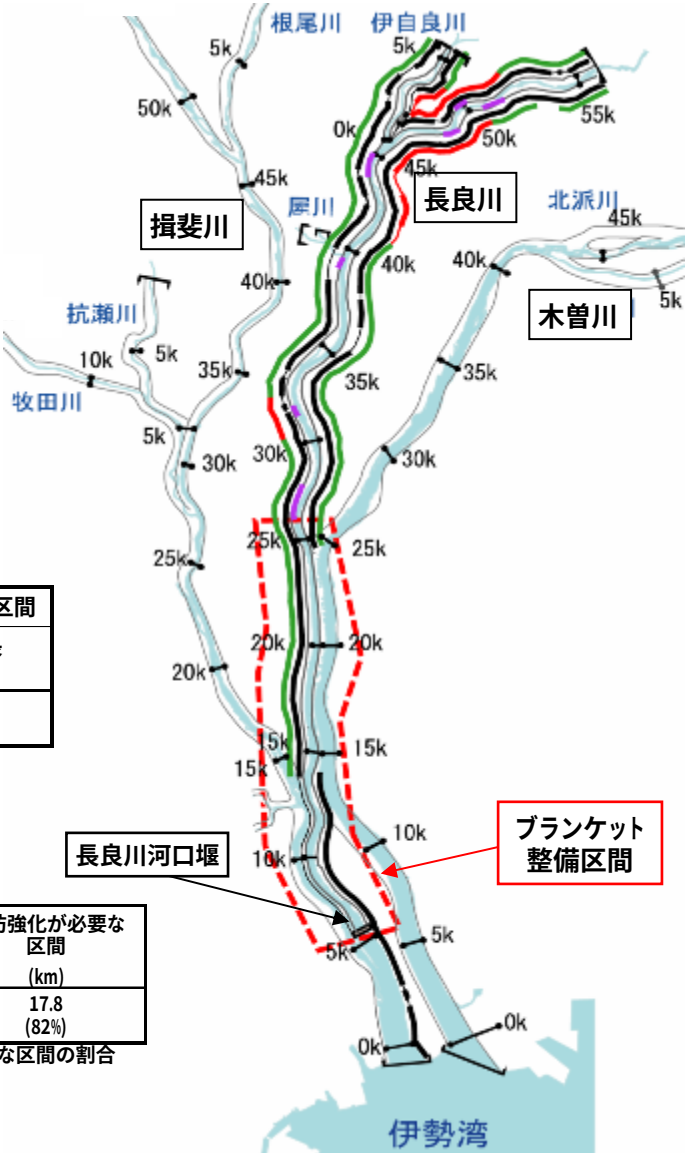
堤防詳細点検結果(H19.3現在)
