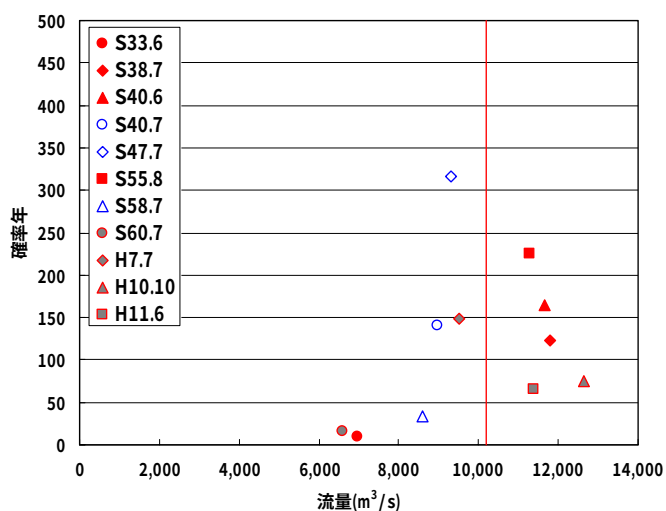
図 4-10 尾関山地点の引伸ばし後雨量確率と流出量の関係図
