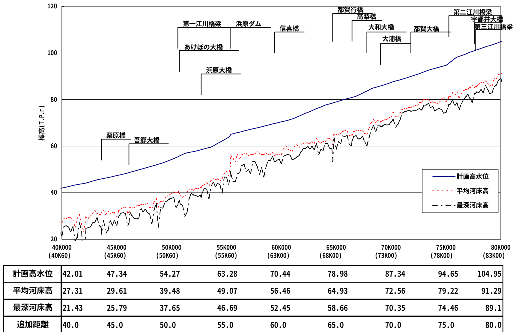
図 8-1(2) 江の川河道区分縦断図(本川：江の川)
