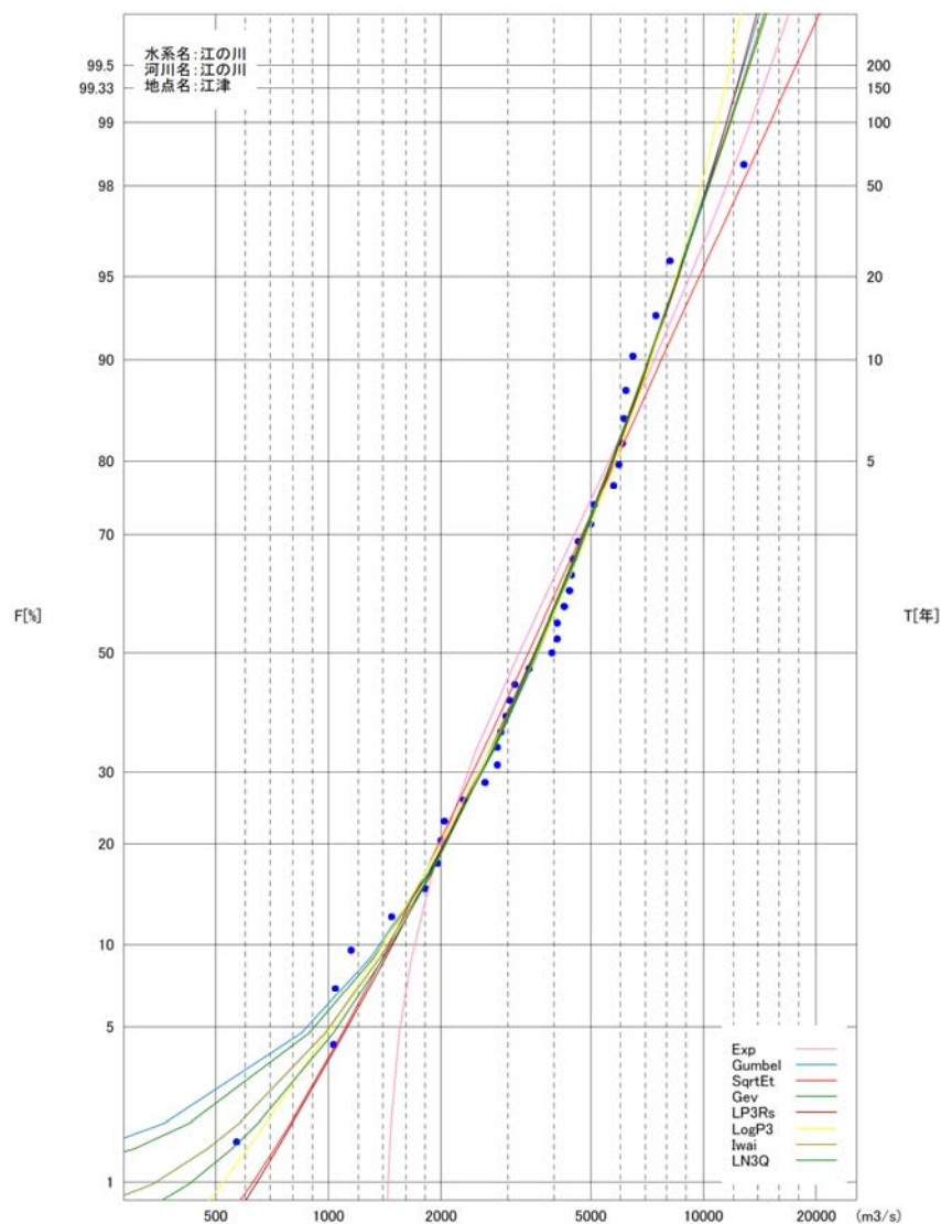
図 4-8 江津地点流量確率計算結果図
