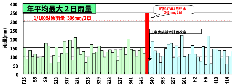
図 4-6(1) 江津地点 年最大2日雨量
