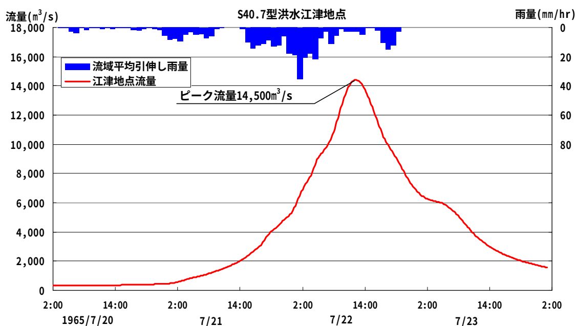
図 4-4(2) 基本高水流量決定洪水（江津地点）
