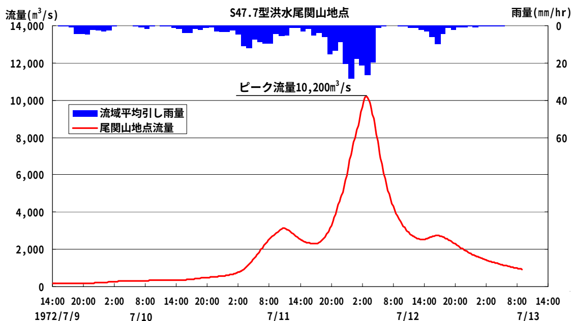
図 4-12(1) 基本高水流量決定洪水（尾関山地点）
