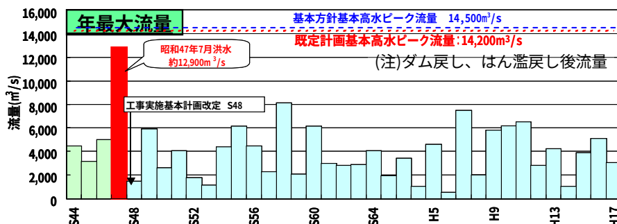
図 4-5(2) 尾関山地点 年最大流量
