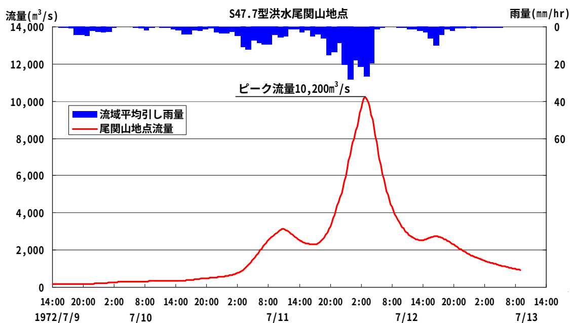
図 4-4(1) 基本高水流量決定洪水（尾関山地点）
