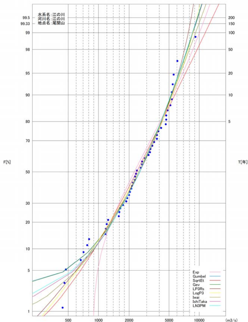
図 4-7 尾関山地点流量確率計算結果図
