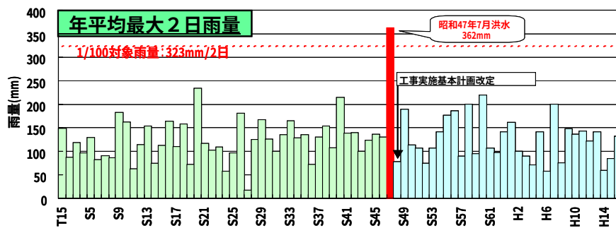
図 4-5(1) 尾関山地点 年最大2日雨量
