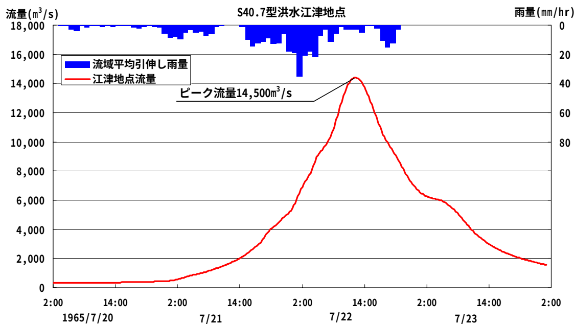
図 4-12(2) 基本高水流量決定洪水（江津地点）
