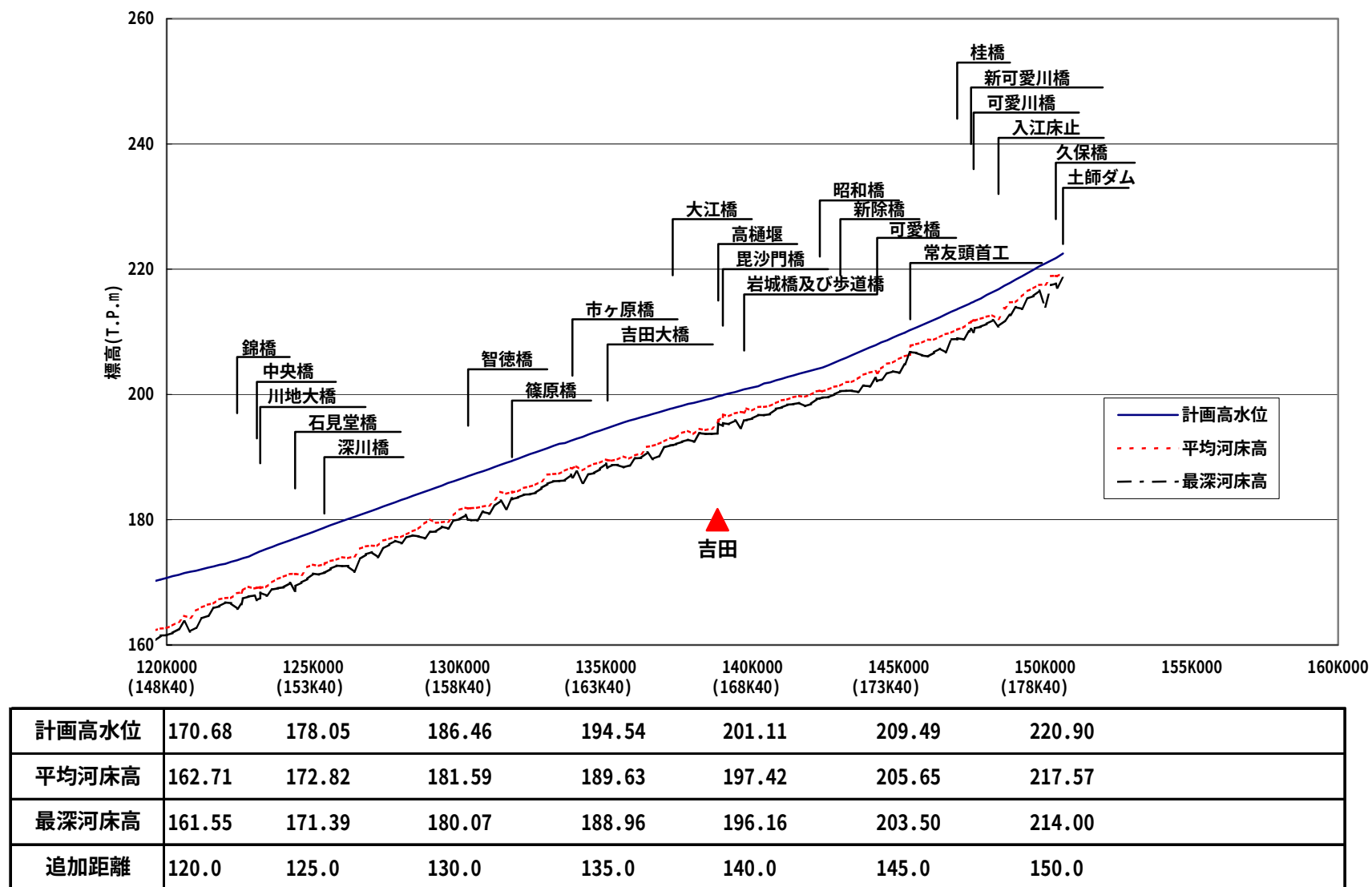
図 8-1(4) 江の川河道区分縦断図(本川：江の川)
