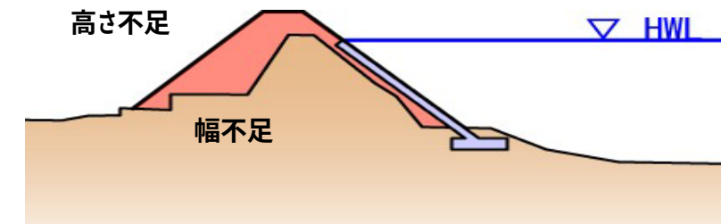
堤防断面不足対策 (堤防の整備)
