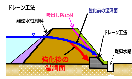
堤防強化対策のイメージ図
