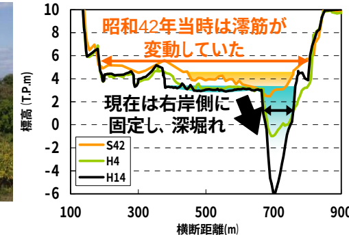
滞筋の固定化 (木曽川38k付近)
