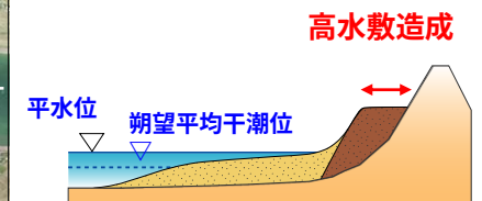
干潟再生断面イメージ
