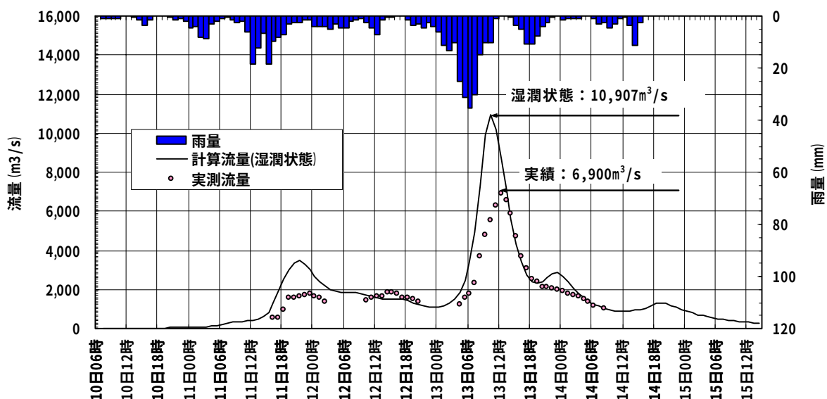
図 4-23 昭和 35 年 8 月洪水ハイト・ハイドログラフ（平成 14 年 7 月洪水流域湿潤状態）
