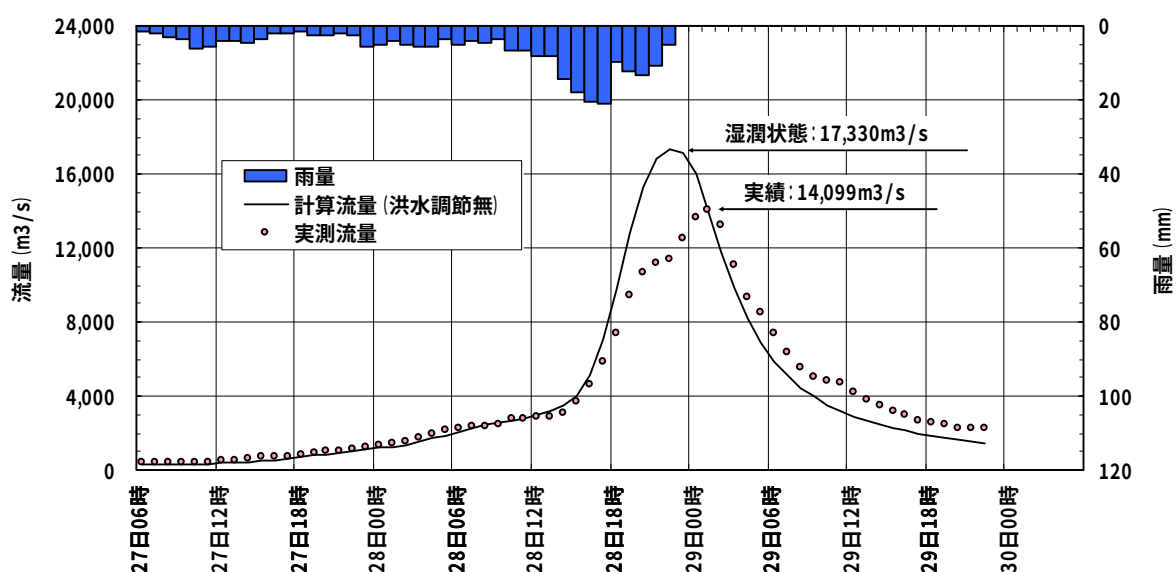
図 4-11 昭和 58 年 9 月洪水ハイレート・ハイドログラフ（昭和 39 年 9 月洪水流域湿潤状態）
