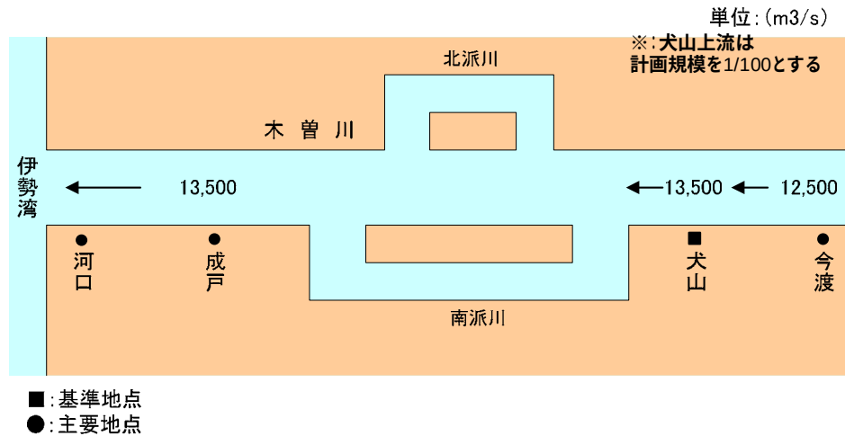
図 6-1 木曽川計画高水流量図 基本方針(案)
