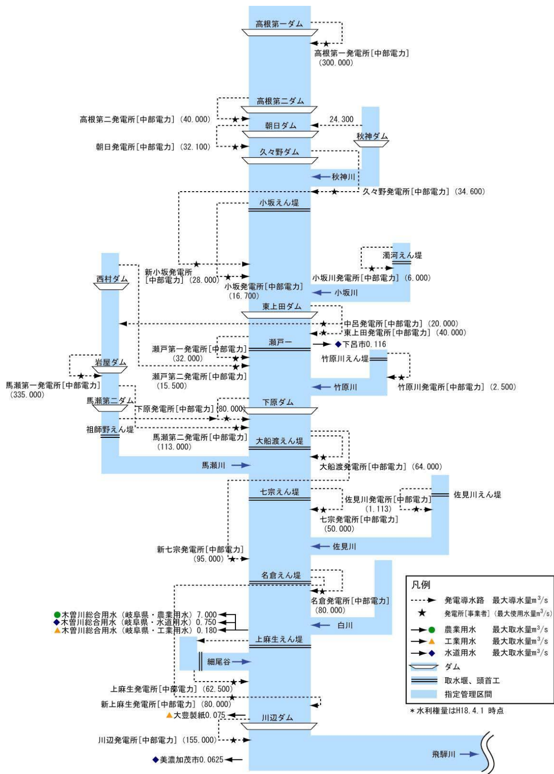
図 2.2(2) 木曽川水利模式図(2/3) (主要な水利権を記載)
