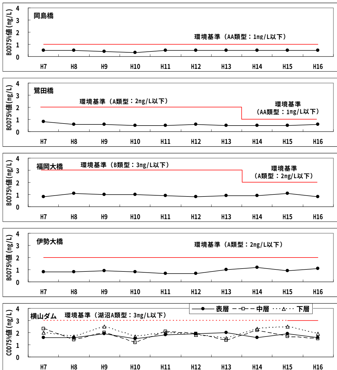
図 5.4 揖斐川環境基準点における BOD75%値経年変化 (平成 7 年～16 年)
