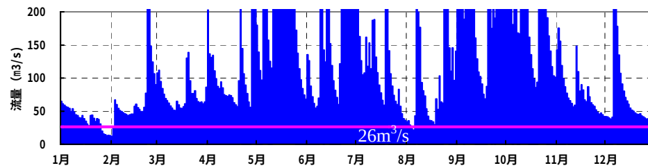
図 6.4(4) 日平均流量（長良川忠節地点：平成 12 年～平成 16 年）
