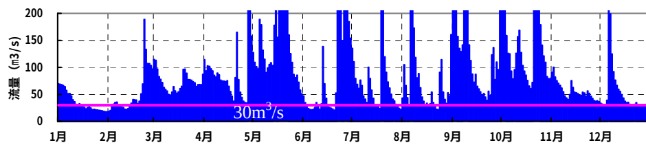
図 6.4(6) 日平均流量（揖斐川万石地点：平成 12 年～平成 16 年）
