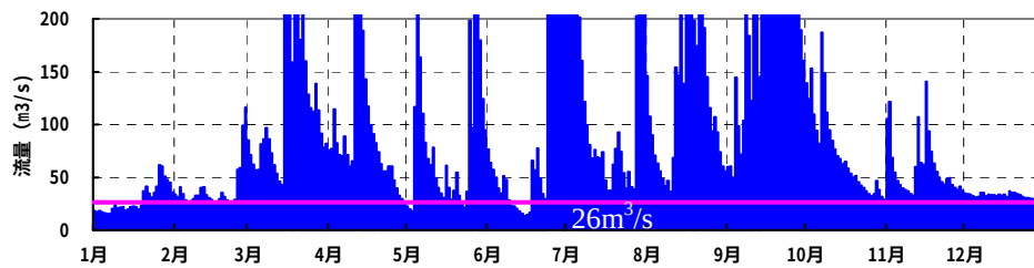
図 6.4(3) 日平均流量（長良川忠節地点：平成7年～平成11年）
