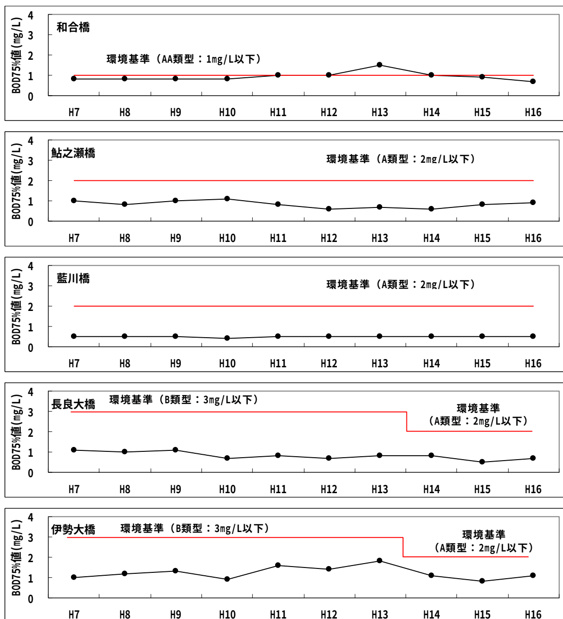
図 5.3 長良川環境基準点における BOD75%値経年変化 (平成 7 年～16 年)
