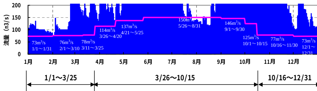
図 6.4(2) 日平均流量 (木曽川今渡地点：平成 12 年～平成 16 年)
