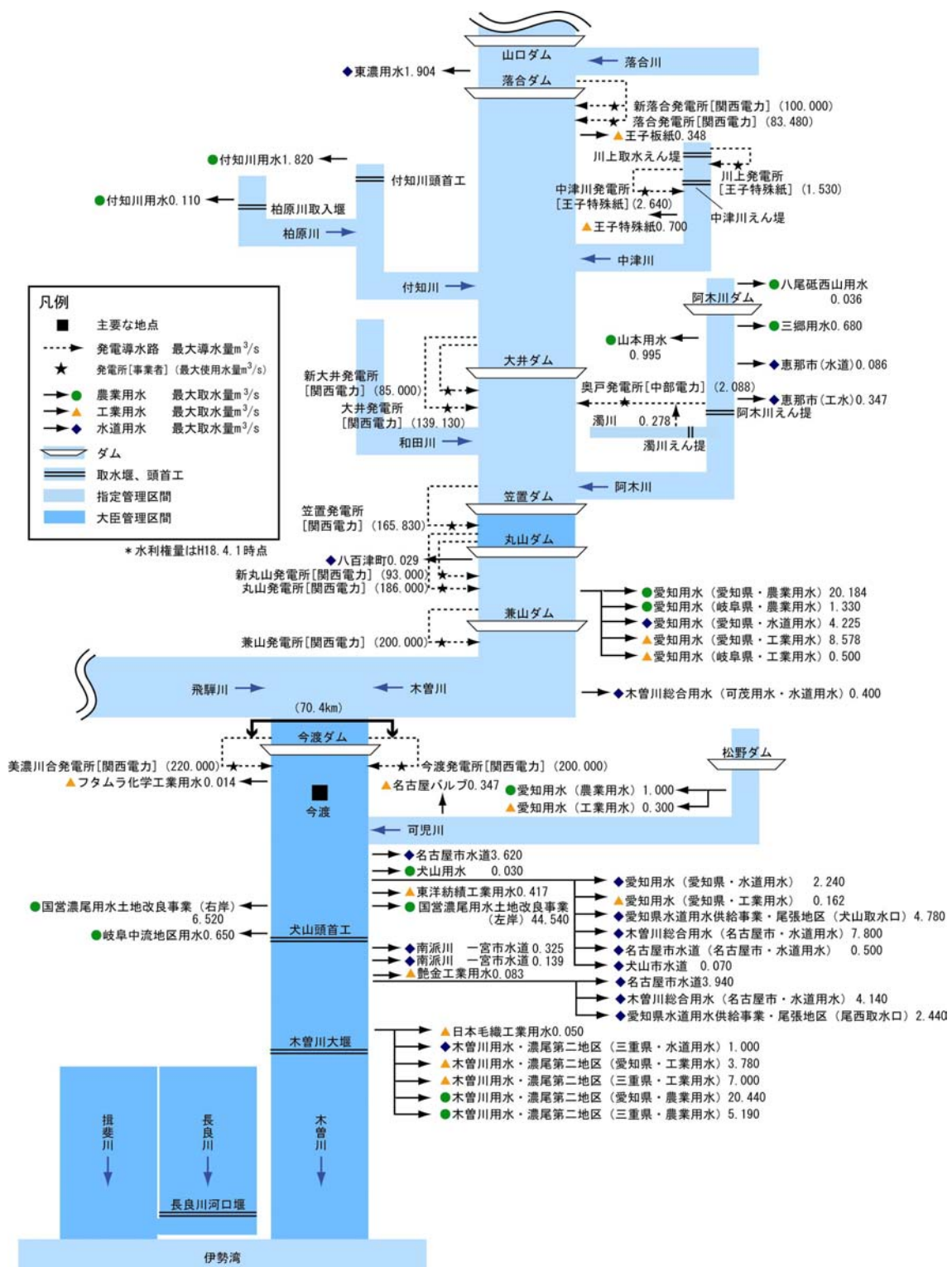
図 2.2(1) 木曽川水利模式図 (1/3) (主要な水利権を記載)
