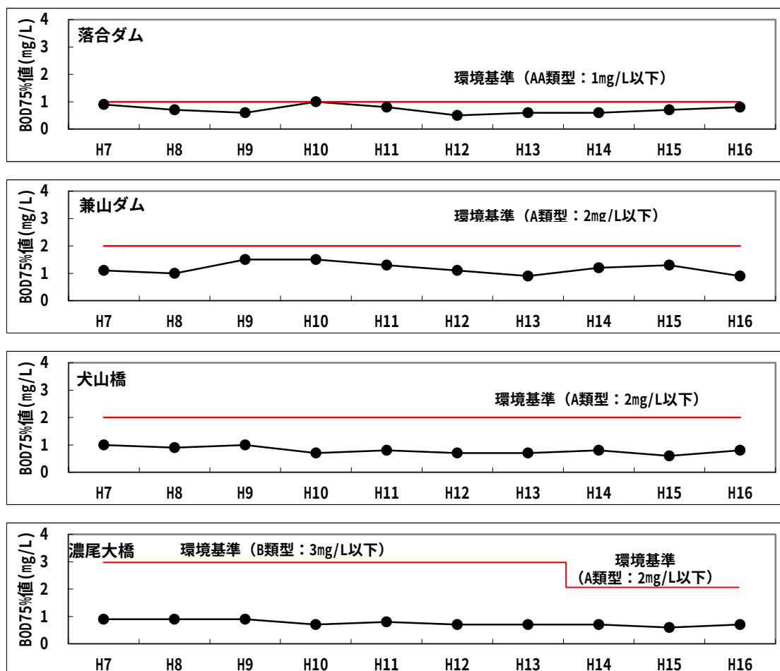
図 5.2(1) 木曽川環境基準点における BOD75%値経年変化 (平成 7 年～16 年)
