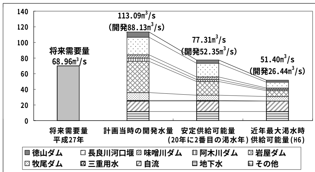
図 3.2 木曽川水系における安定供給可能量の変化（20 年の対象計算年：昭和 54 年～平成 10 年）
