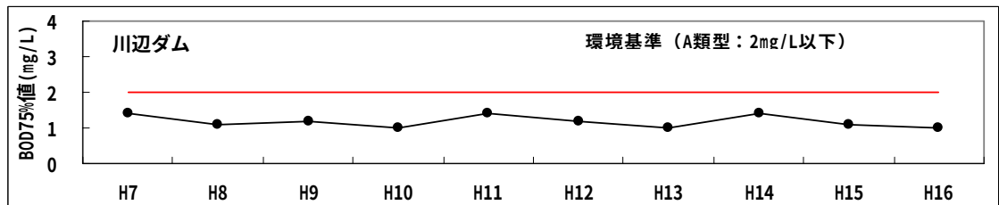
図 5.2(2) 木曽川環境基準点における BOD75%値経年変化 (平成 7 年～16 年)
