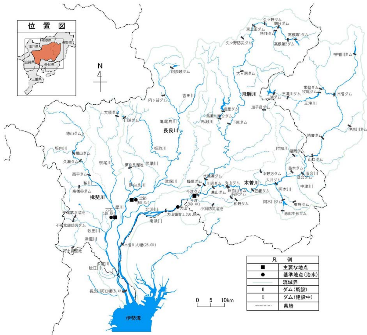
図 1.1 木曽川水系図
