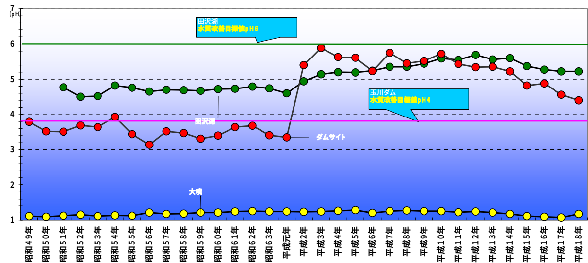
図 6-4 pH の推移
