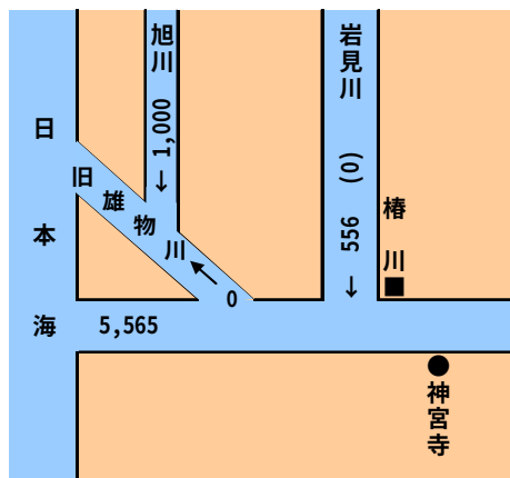
図 4-3 下流部流量配分図
