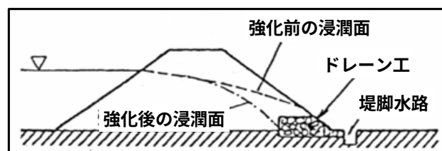
ドレーン工法
