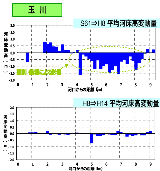
図 8-3 河床変動量の経年変化（玉川）
