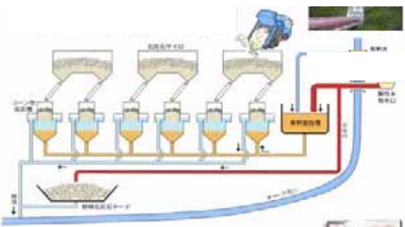
図 6-6 フローシート
