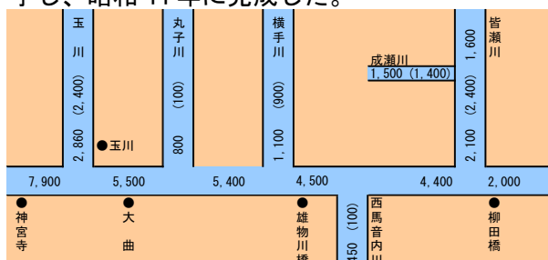
図 4-6 流量配分図（第 1 次改定計画）
