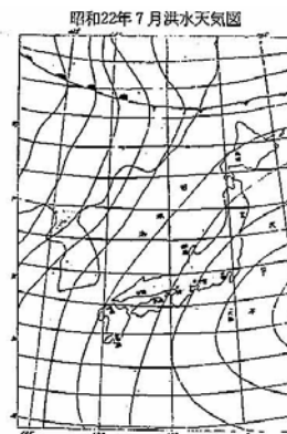
昭和22年7月洪水天気図
