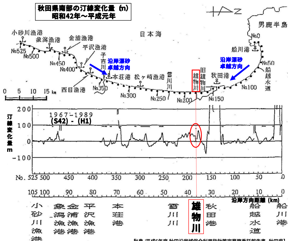
図 8-10 河口付近の海岸侵食状況
