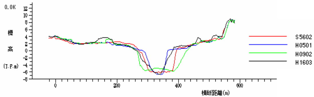
図 8-8 雄物川河口部 (0.0k) の横断図
