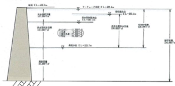
貯水池容量配分図
