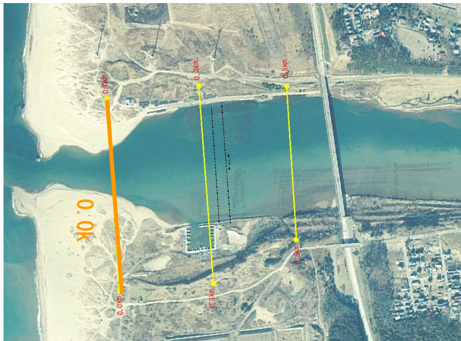
図 4-2 雄物川河口部平面図
