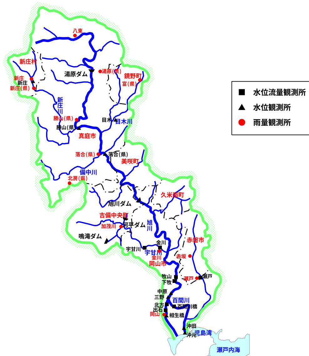
図-9.3.1 旭川水系観測所設置位置
