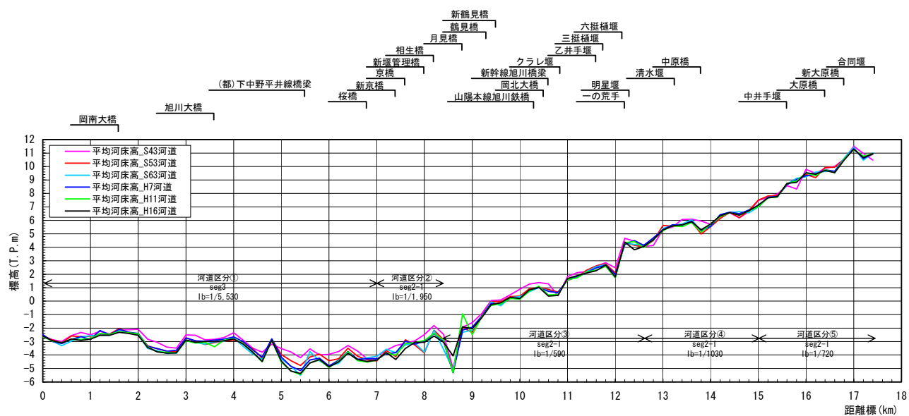
図-8.2.2(1) 旭川水系平均河床高縦断図(旭川)
