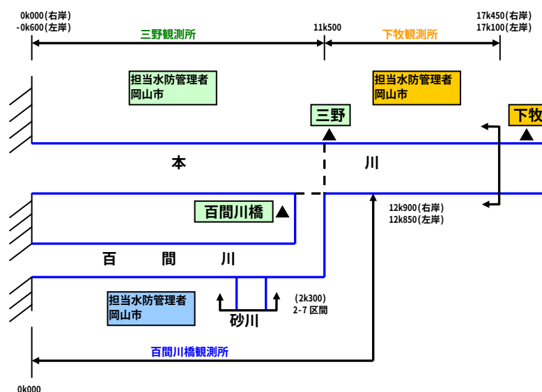
図-9.3.2 水防警報対象水位観測所の分担区域
