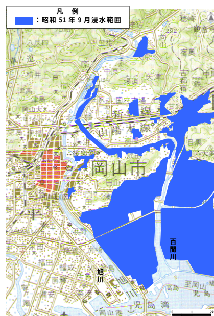
図-4.1.1 昭和 51 年浸水実績図
