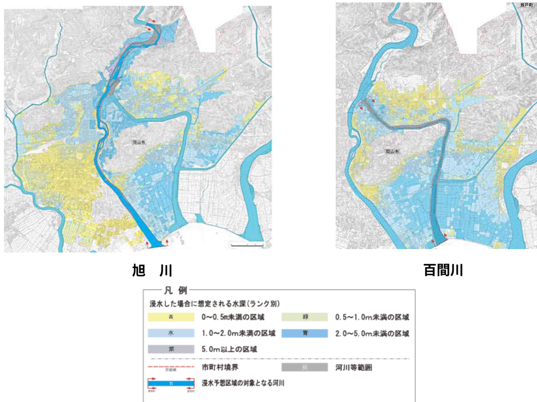
図-9.4.1 浸水想定区域図(国管理区間)
