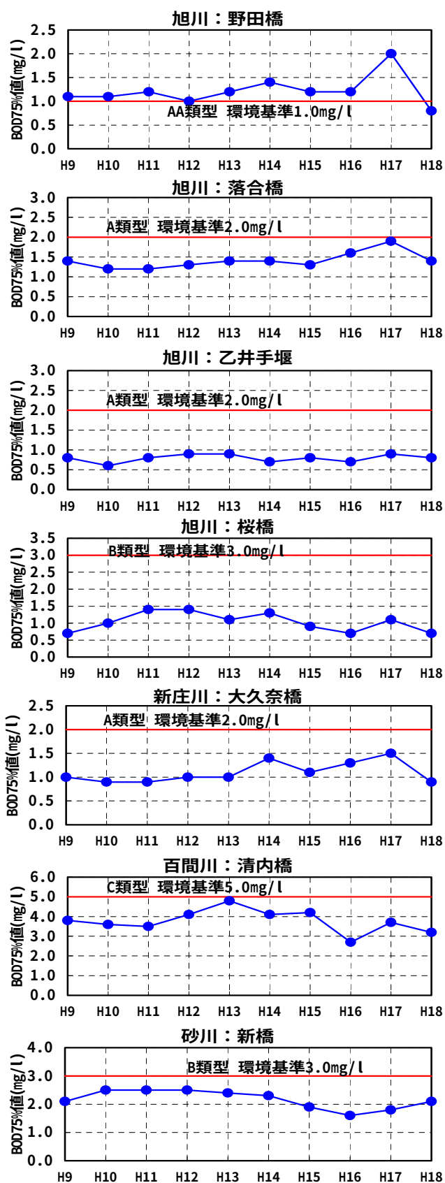
図-6.2.2 主要地点の水質(BOD75%値)経年変化図
