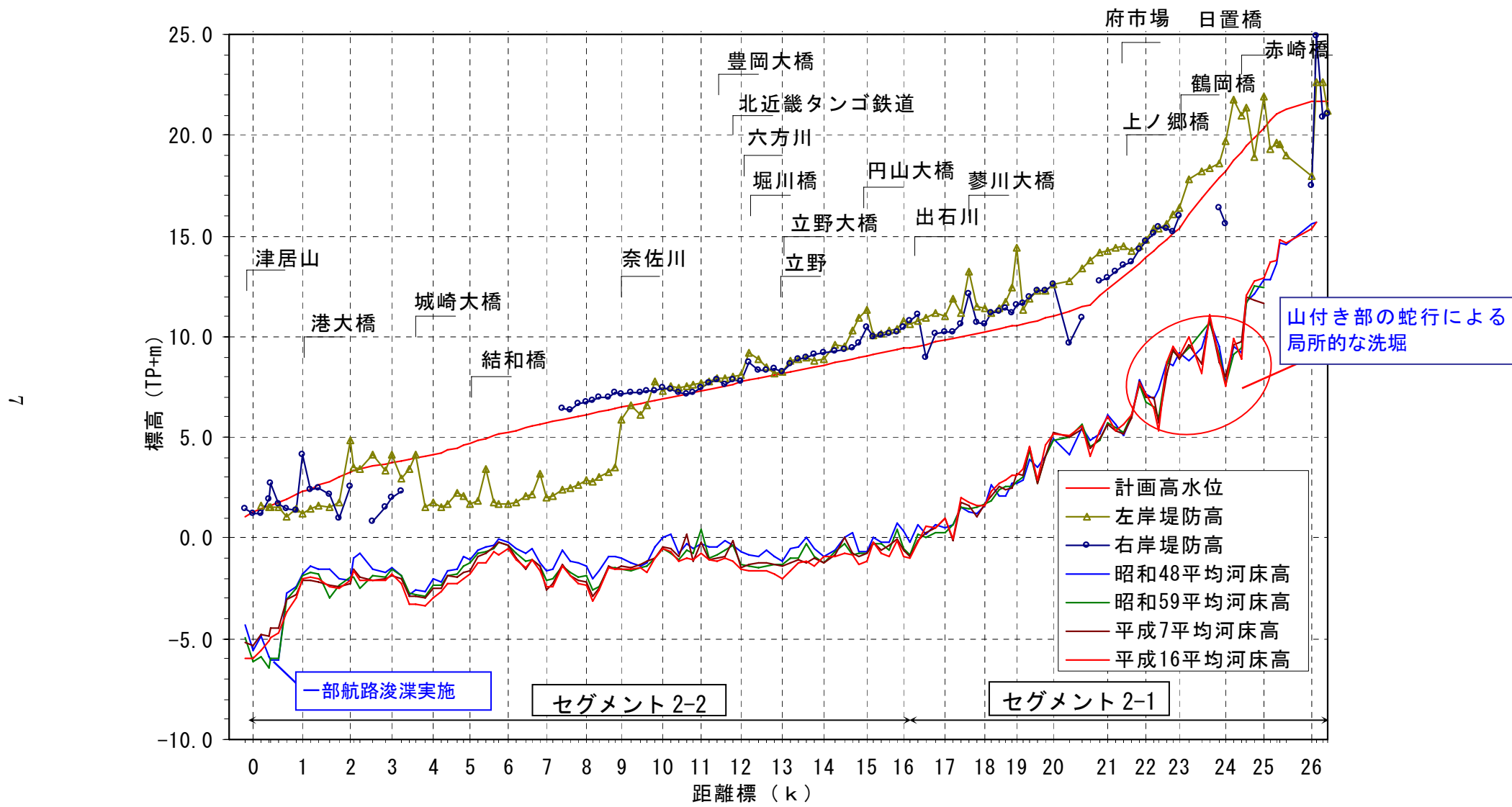
図 2-3 円山川平均河床高縦断図 (昭和 48 年～平成 16 年)
