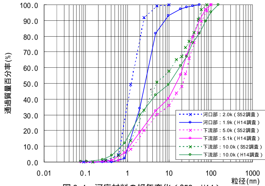
図 2-4 河床材料の経年変化 (S52 H14)
