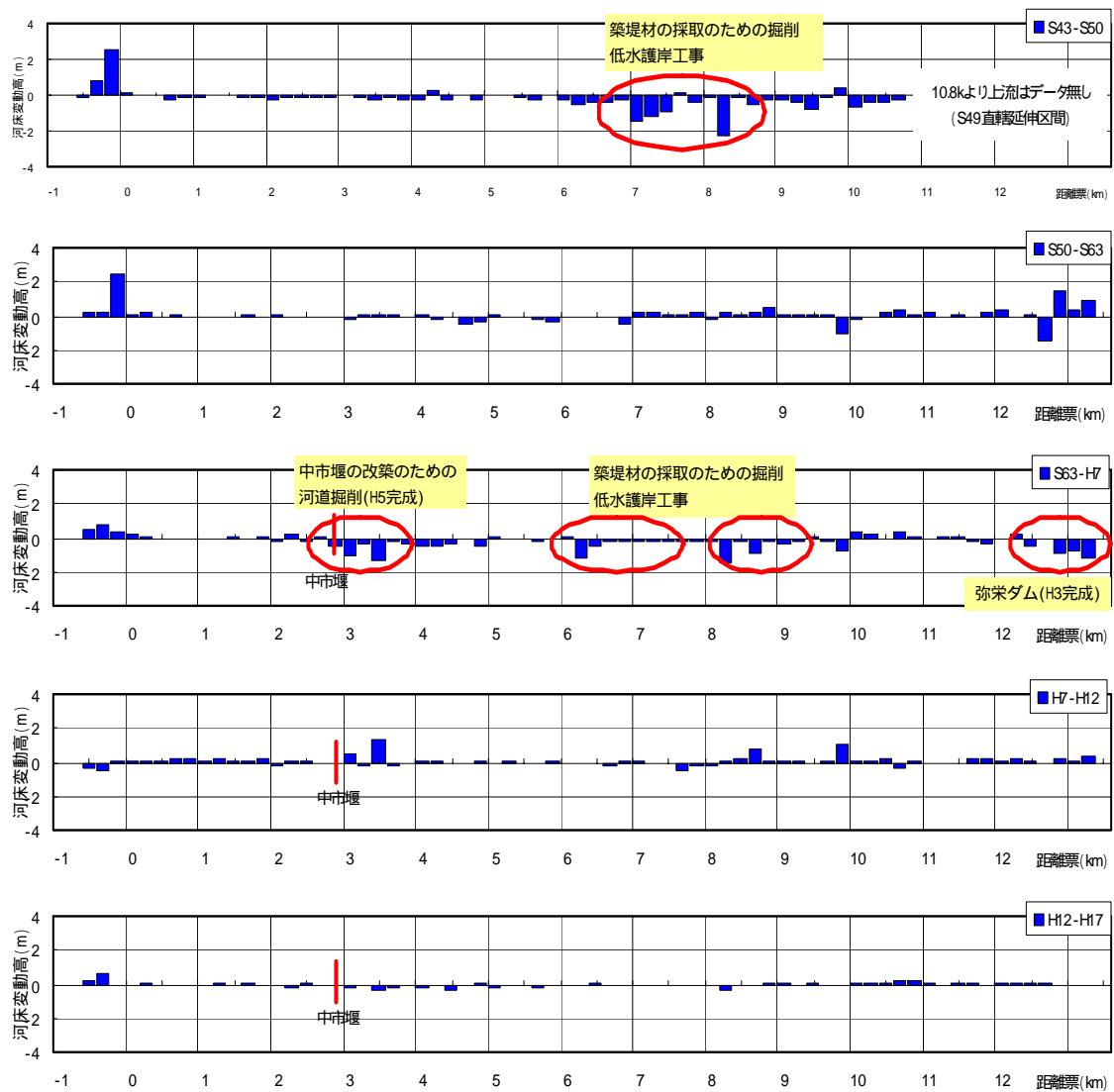
図 2-2 河床変動量の経年変化図 (小瀬川)
