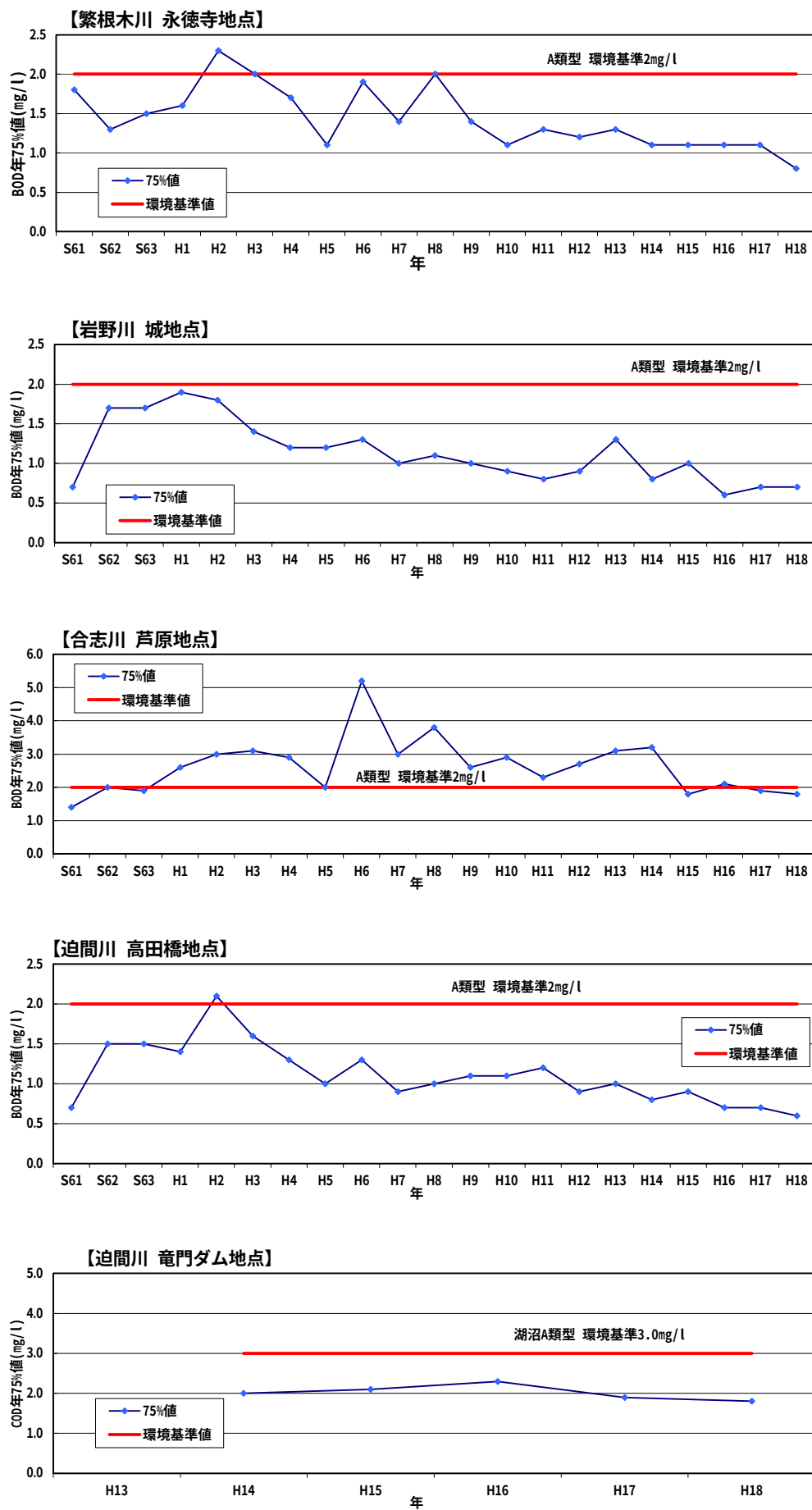
図-6-2(2) 近年 20 ヶ年の BOD75%値経年変化図（竜門ダムは COD）
