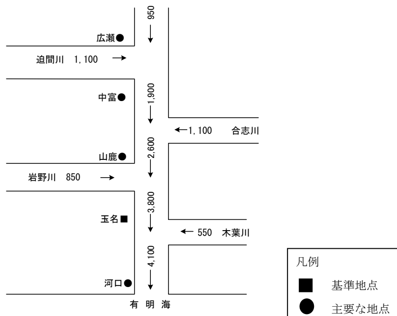
図 6-1 菊池川計画高水流量図 基本方針（案）
