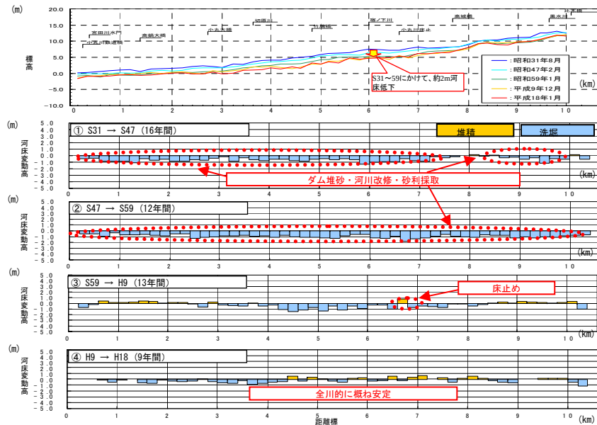
小丸川平均河床高経年変化図
