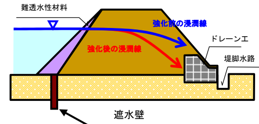
堤防の質的強化のイメージ図
