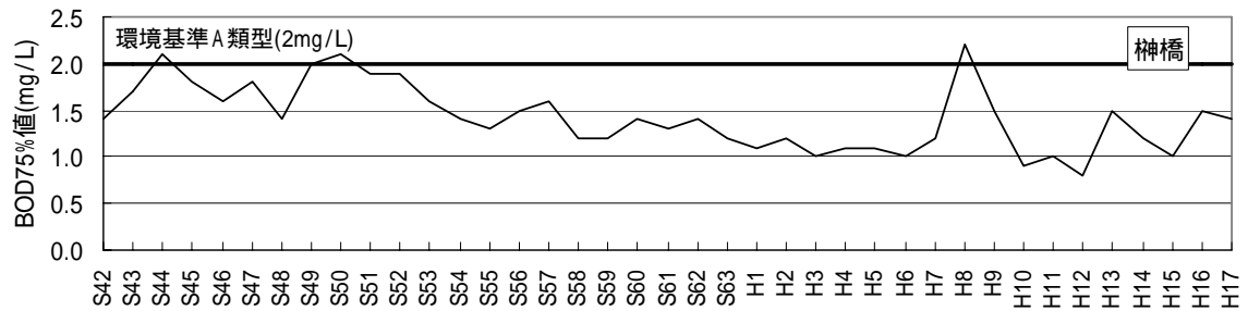
図 5-5 久慈川 榑橋地点における BOD 経年変化
