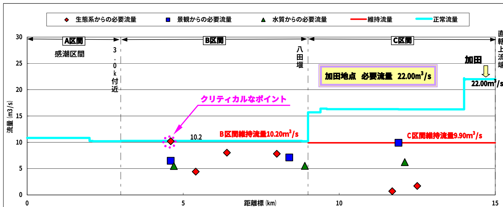
図 6-1(5) 仁淀川水収支縦断図 かんがい期(10/1～10/31)
