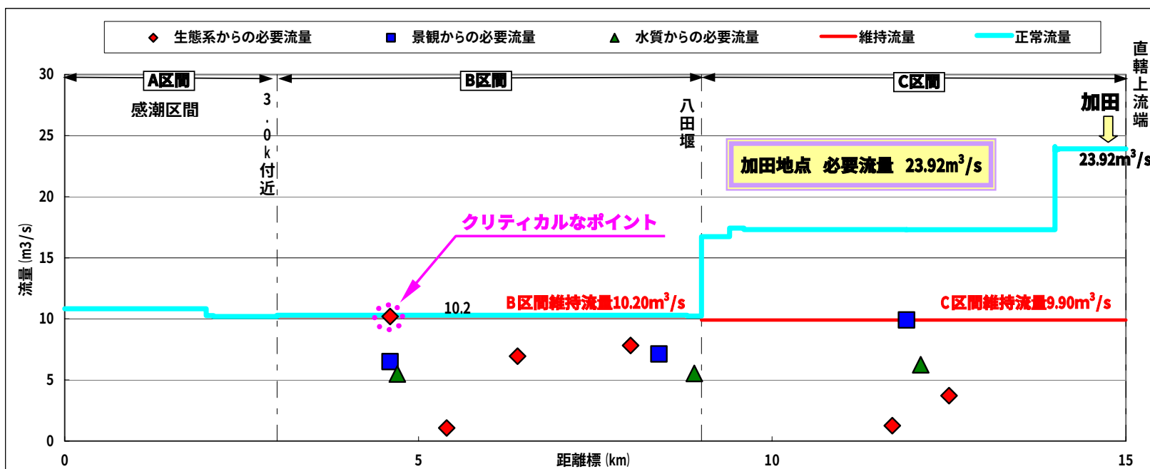
図 6-1(4) 仁淀川水収支縦断図 かんがい期(5/1~9/30)
