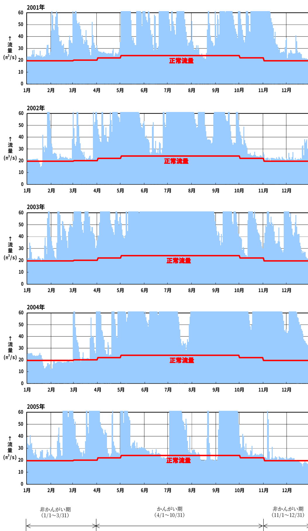
参考-図1 日平均流量図（加田地点）
