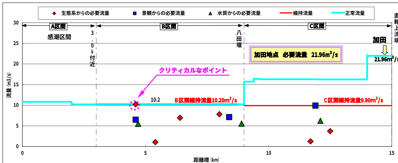
図 6-1(3) 仁淀川水収支縦断図 かんがい期(4/1~4/30)
