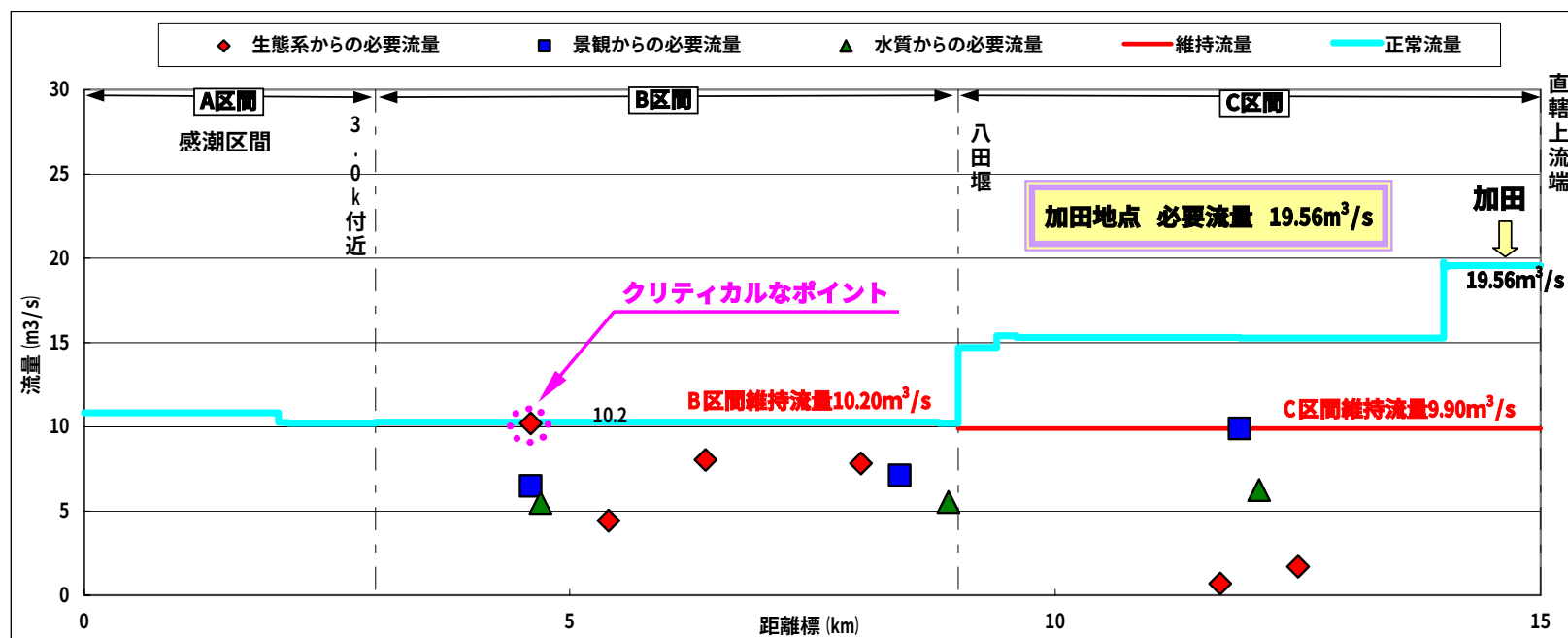
図 6-1(6) 仁淀川水収支縦断図 非かんがい期(11/1~12/31)
