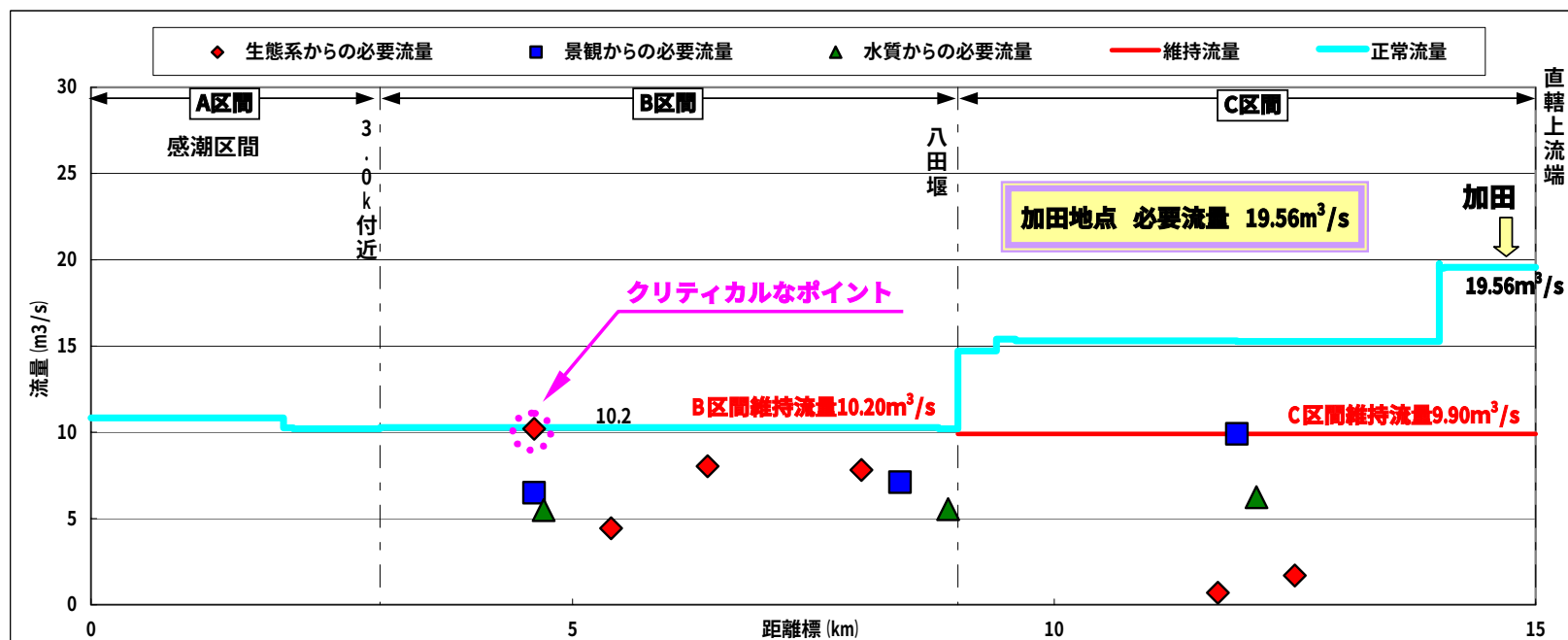
図 6-1(1) 仁淀川水収支縦断面図 非かんがい期(1/1~2/28)
