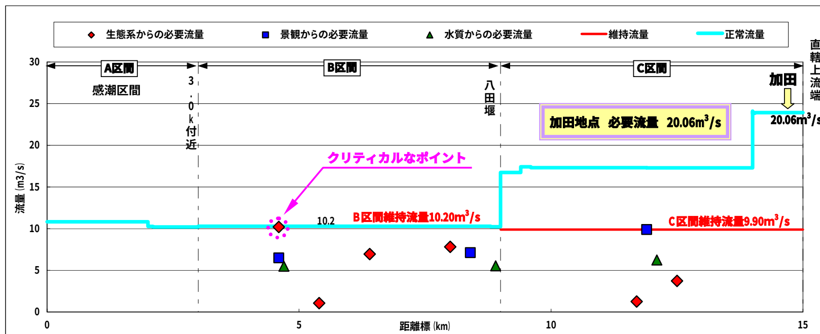
図 6-1(2) 仁淀川水収支縦断図 非かんがい期(3/1～3/31)
