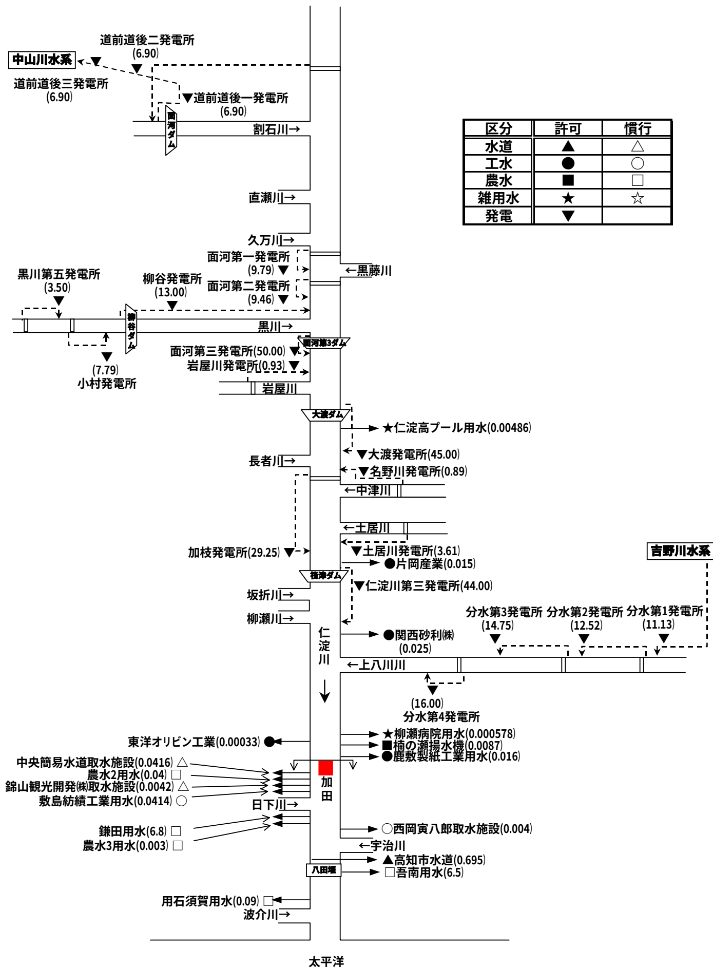
図 2-2 仁淀川水利用の現況模式図
