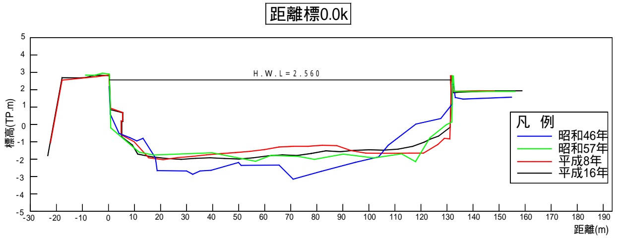
図3-2 北川河口部(0.0k)の横断面図
