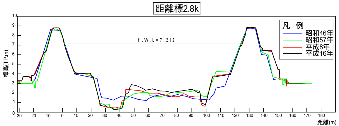
図2-4(1) 代表横断図（北川2.8k）
