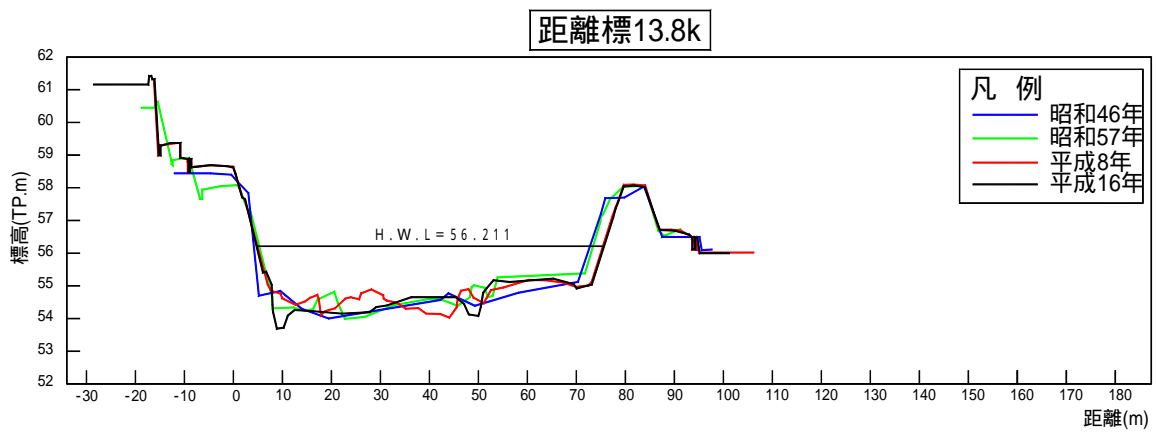
図2-4(2) 代表横断図（北川13.8k）
